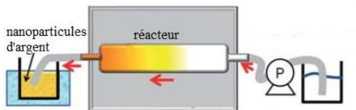
Figure 44: Dispositif expérimental décrit par Horikoshi et al. 133
