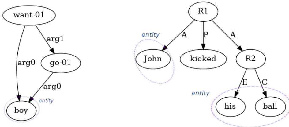
FIGURE 4.4 – Graphes sémantiques et quelques filets sémantiques pour les phrases “ The boy wants to go. ” (à gauche) et “ John kicked his ball. ” (à droite), respectivement basés sur un graphe AMR et un graphe UCCA.
