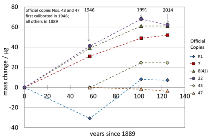
Fig. 5.9 Évolution de la masse des six témoins par rapport à celle du PIK (figure extraite de [64]).
