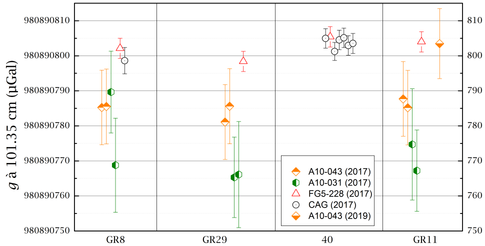
Fig. 5.17 Résultats par station de la comparaison nationale de 2017 à une hauteur de transfert de 101.35cm.
