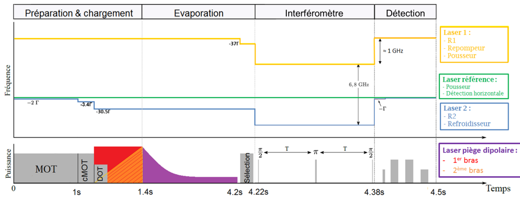
Fig. 3.18 Séquence totale de la mesure de g_{UF} . Les différentes fréquences et puissances des lasers sont représentées ici.
