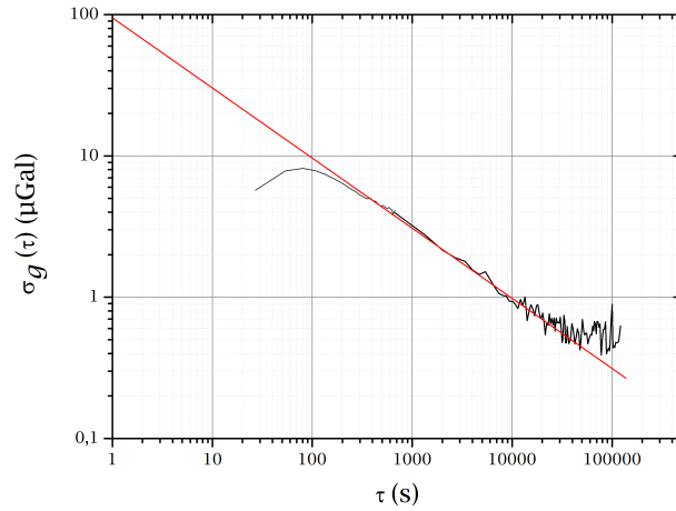
Fig. 3.35 Écart type d'Allan de la mesure continue de g en utilisant des atomes piégés.
