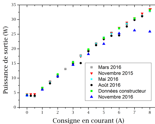
Fig. 3.2 Puissance de sortie du laser Kheopsys en fonction du courant d'entrée.
