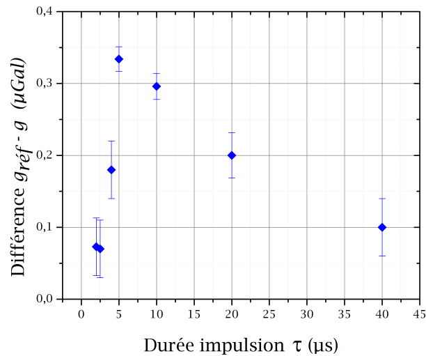
Fig. 4.23 Simulation de la différence des deux séquences d'interféromètres en fonction de la durée de l'impulsion Raman \tau pour une température de 2\mu\text{K} et une distribution atomique de type lorentzienne b .
