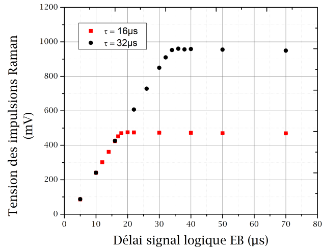
Fig. 4.5 Temps de réponse de l'échantillonneur-bloqueur pour des impulsions de 16 et 32 \mu s .
