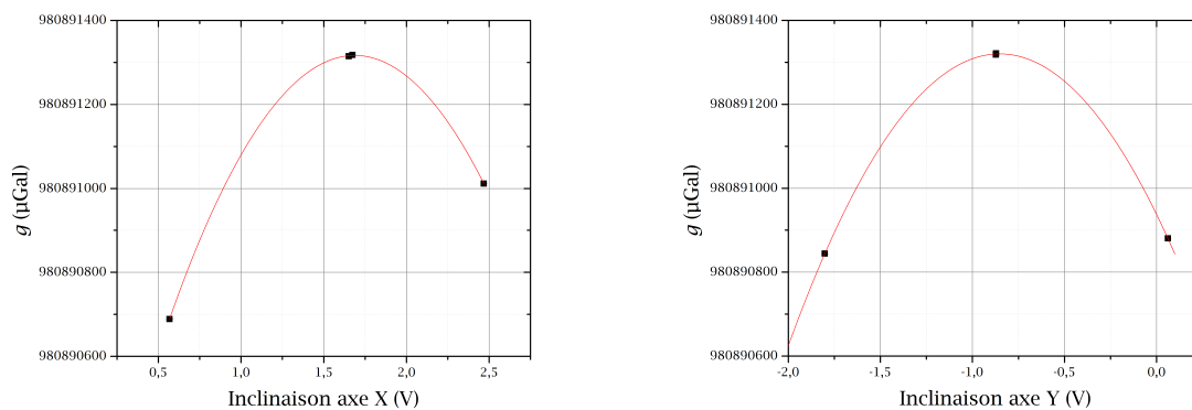
Fig. 2.16 Mesure de g en fonction de l'inclinaison du gravimètre pour les deux axes X et Y de l'inclinomètre respectivement à gauche et à droite.
