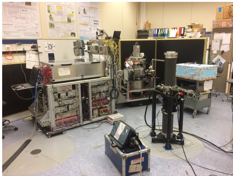
Fig. 5.14 Salle GR lors de la comparaison des gravimètres. Le FG5 #228 au premier plan est placé sur la station GR40 . Le CAG situé en arrière plan mesure sur la station GR8 .
