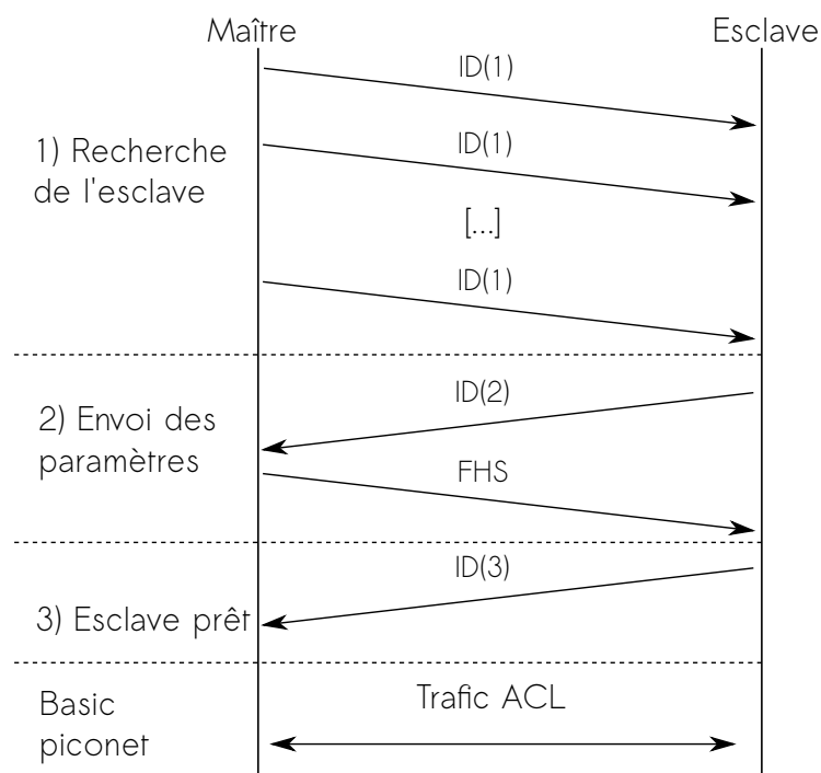
FIGURE 7.3: Procédure de paging
