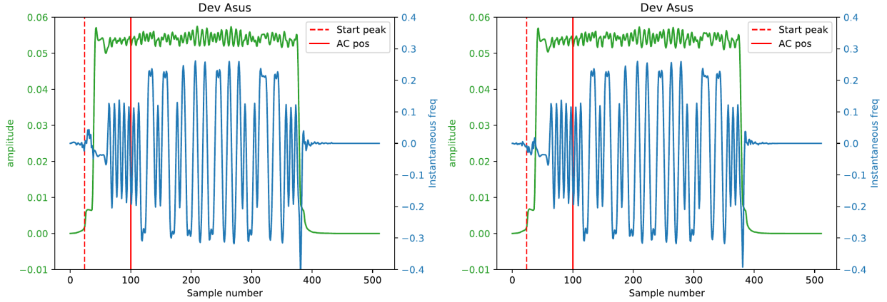
(a) Trace d'amplitude et de fréquence accumulées de 1464 paquets ID (Asus BT-400)
