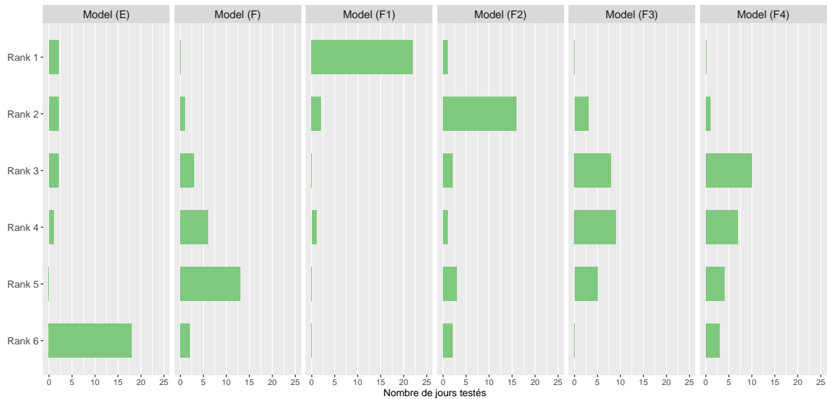
FIGURE 3.4 – Classement des 6 modèles (E),(F),(F1),(F2),(F3) et (F4) en compétition pour les 30 jours de test du mois de Novembre 2019. Le Rank 1 correspond au modèle dont la logloss est minimale tandis que le Rank 6 correspond au modèle qui a la plus mauvaise logloss pour un jeu de test donné.
