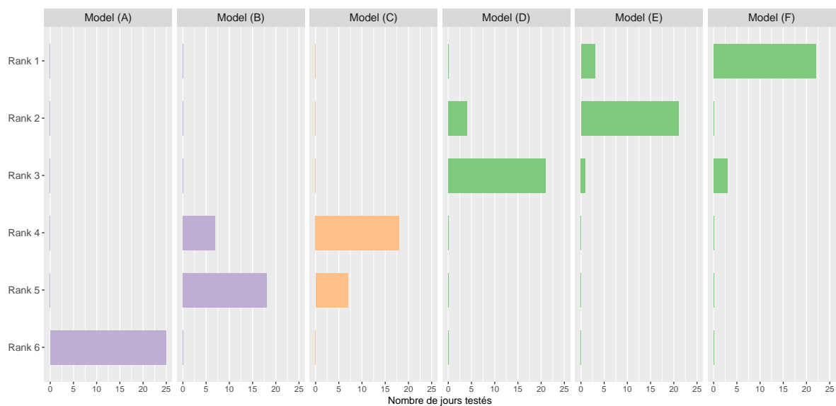
FIGURE C.3 – Classement des 6 modèles (A),(B),(C),(D),(E) et (F) en compétition pour les 30 jours de test du mois de Décembre 2019. Le Rank 1 correspond au modèle donc la logloss est minimale tandis que le Rank 6 correspond au modèle qui a la pire logloss pour un jeu de test donné.
