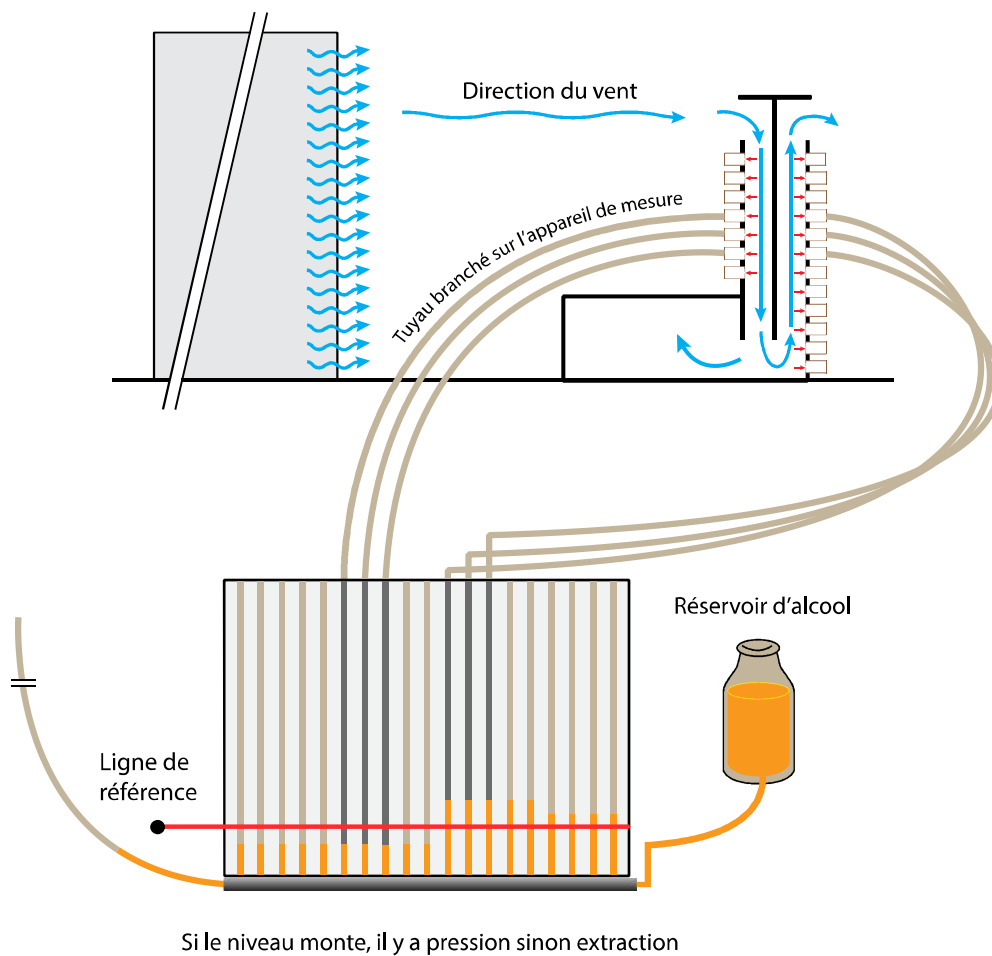
Figure 190 : Fonctionnement de la soufflerie
