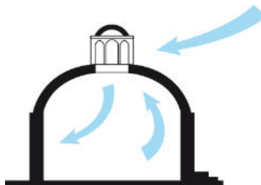
Figure 116 : Fonctionnement d'un Kolah Farangui
