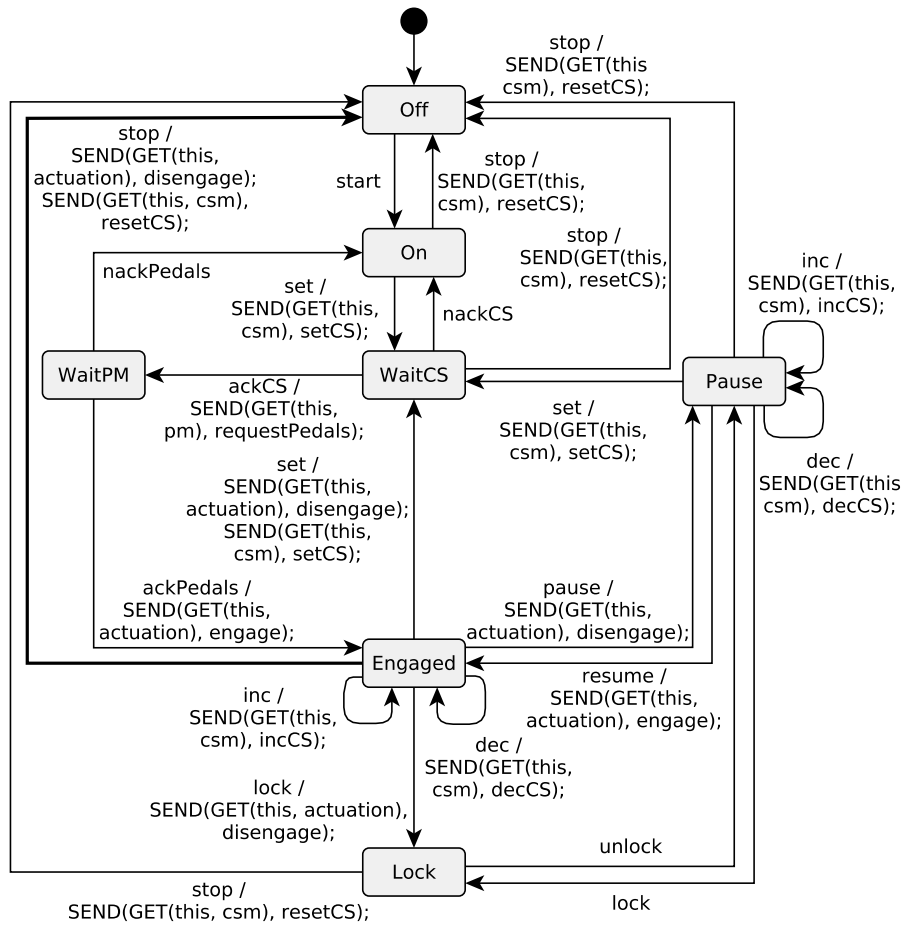
(a) Machine à états de la classe Controller .
