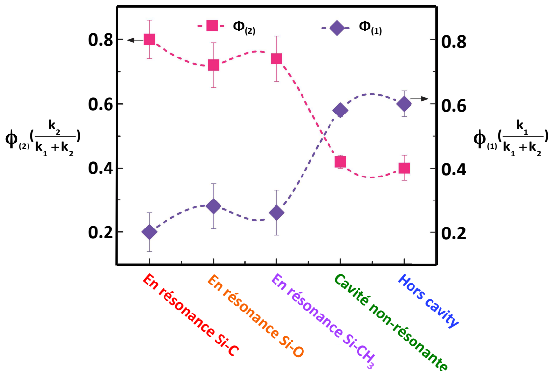
Figure 7. Graphique montrant le rendement du produit (1) ( \phi_{(1)} , losange violets) et (2) ( \phi_{(2)} , carrés rose) en régime de VSC de différents modes de vibrations de (R) , ainsi que dans une cavité non-résonante et hors cavité. Les marges d'erreur ont été déterminées à partir de l'écart-type d'au moins cinq expériences.
