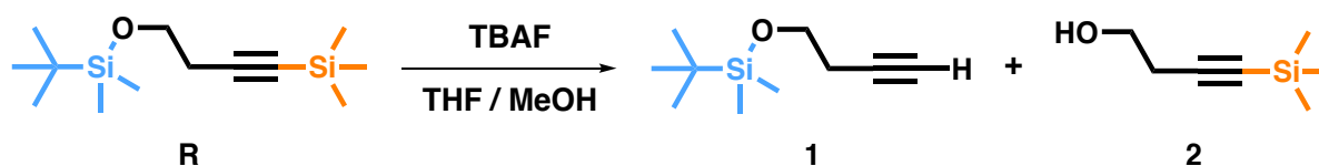
Figure 3. Les deux réactions de rupture de liaison silyles possibles (rupture de la liaison Si-C pour former (1) , rupture de la liaison Si-O scission pour former (2) ) pour la réaction entre (R) et le TBAF à température ambiante dans un mélange de méthanol et de THF.
