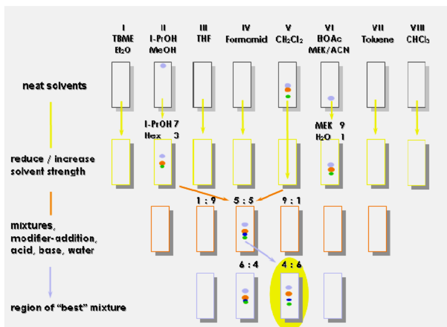
Figure 14: Schéma d'optimisation des solvants d'élution
