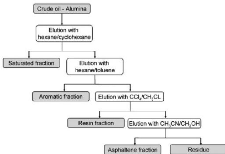
Figure 5 : Schéma du fractionnement SARA[2]
