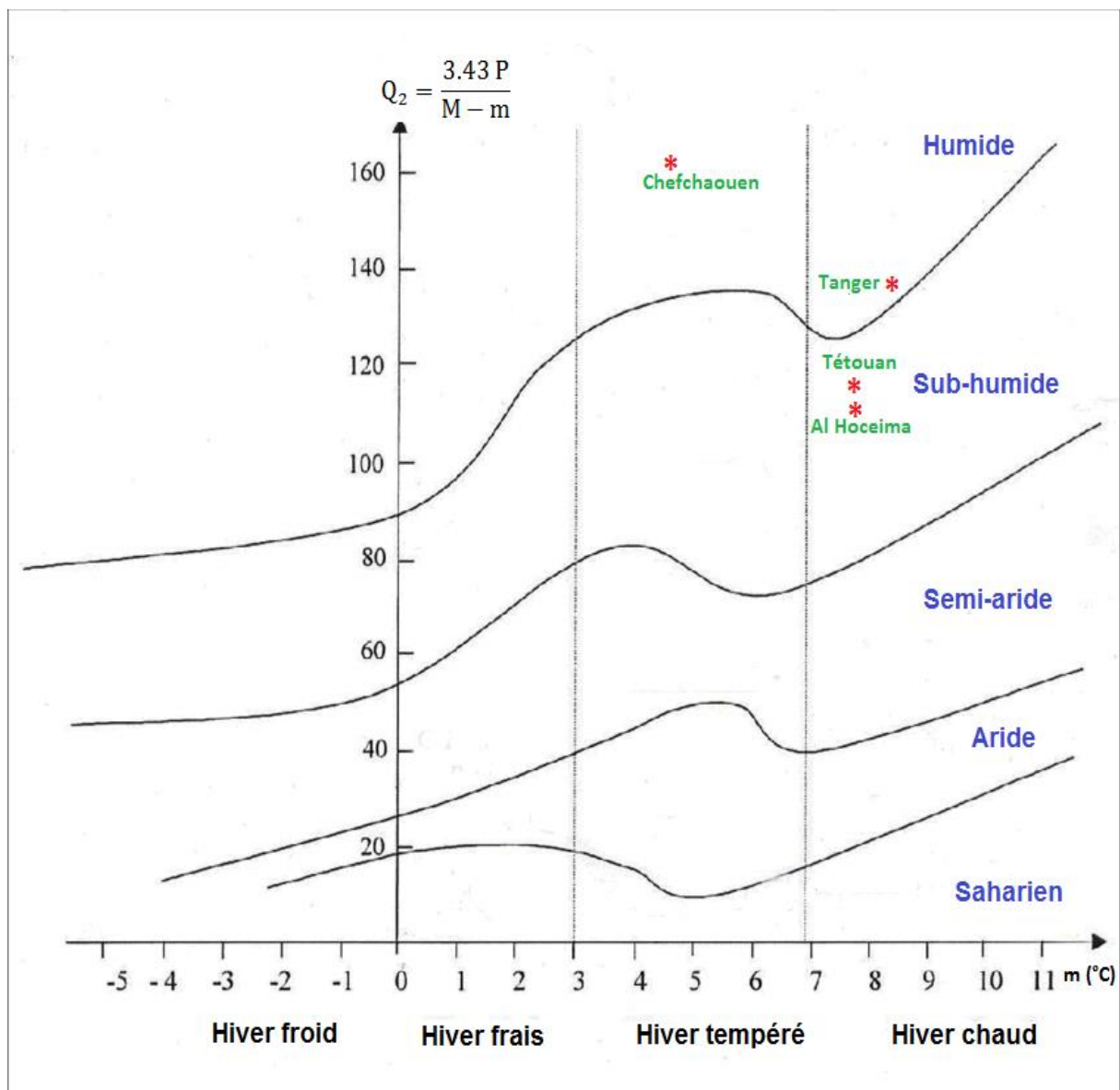
Figure 6 : Projection des stations climatiques dans le climagramme d'EMBERGER.
