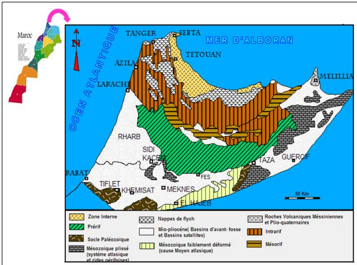
Figure 4 : Carte géologique simplifiée du Rif (Suter, 1980) (carte géologique du Rif au 1/500000).
