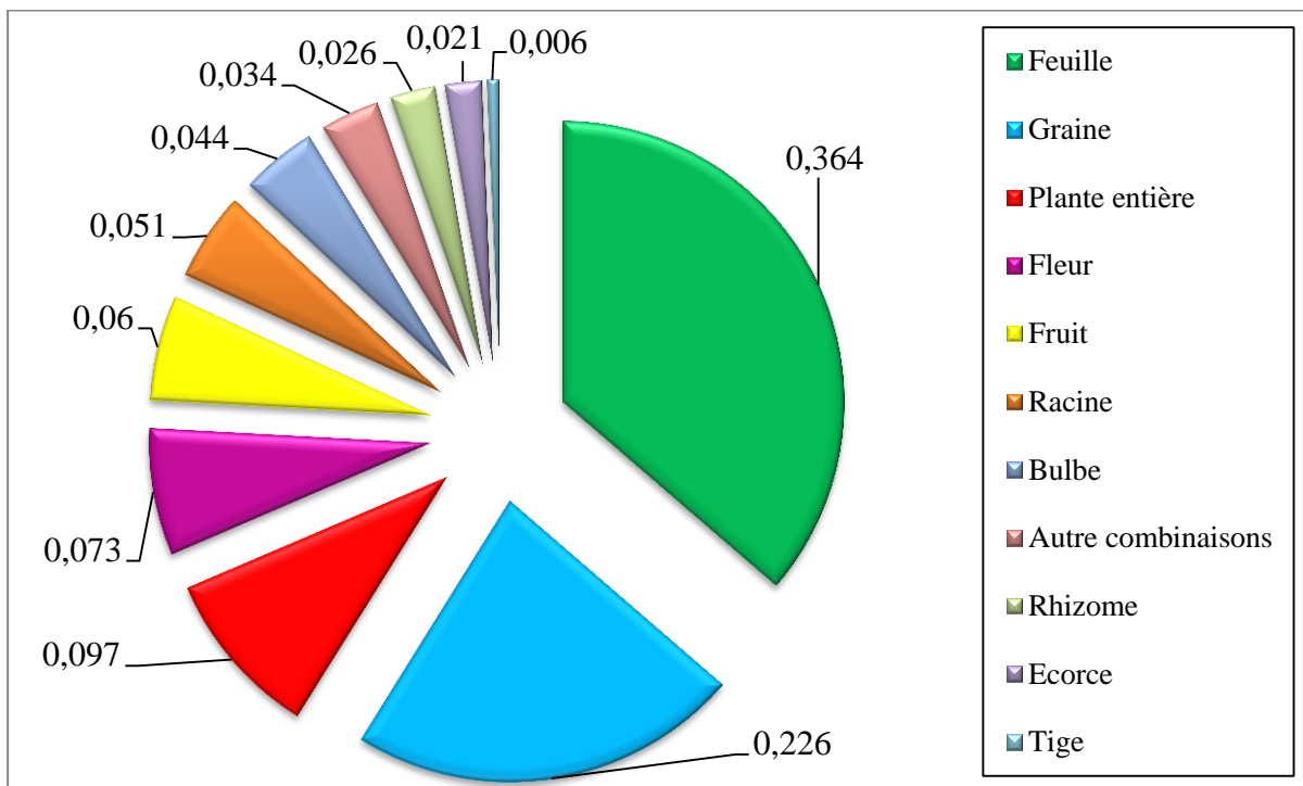
Figure 17 : Différentes parties de PAM utilisées dans la zone d'étude et leur PPV.
