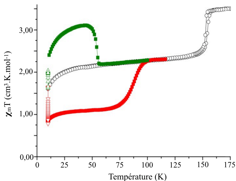
Figure 23. Évolution du produit \chi_m T en fonction de la température du composé [\text{Fe}^{\text{II}}(\text{trz-py})_2\{\text{Pt}^{\text{II}}(\text{CN})_4\}].3\text{H}_2\text{O} sous excitation lumineuse à 510 nm, et à 830 nm. [62]
