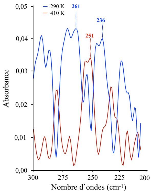
Figure 13. Spectres infrarouge dans la zone 300 à 200 cm -1 du complexe (6) à 290 K (BS) et 410 K (HS).
