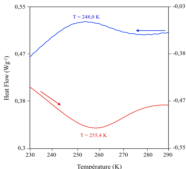
Figure 9. Profil DSC du composé NR50-TS à une vitesse de balayage 4 K.min -1 .
