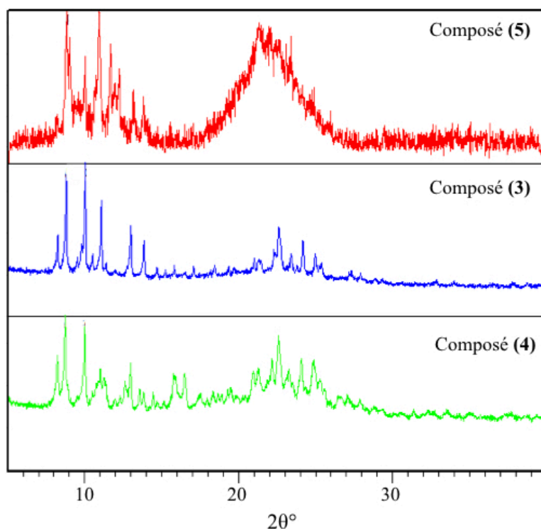
Figure 22. Diffractogrammes de poudre des composés (3) , (4) et (5) .
