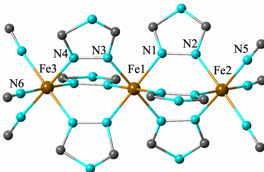
Figure 8. Structure moléculaire du complexe trinuécléaire ordonné complexe [Fe 3 (naphtrtz) 6 (tCNSPr) 6 ] ( 6 ).
