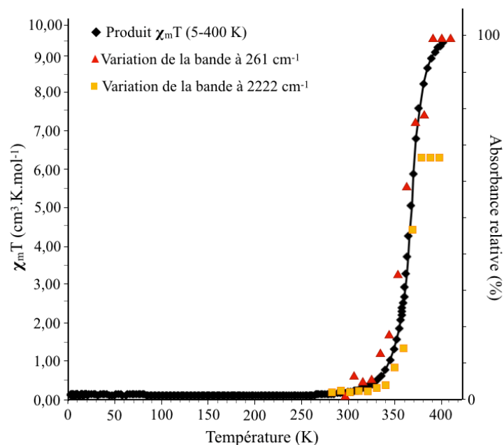
Figure 15. Corrélation entre la susceptibilité magnétique et les absorbances relatives et normalisées pour les bandes infrarouge à 2222\text{ cm}^{-1} (ABS vs. T) et 261\text{ cm}^{-1} (1-ABS vs. T) en fonction de la température.
