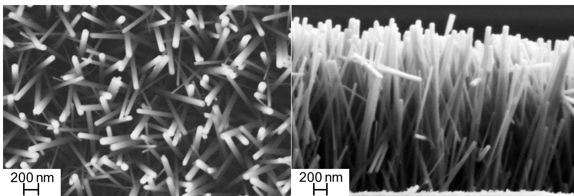
Figure III-8. Images MEB en vue de dessus et en vue transversale des nanofils de ZnO synthétisés avec de l'acétate de zinc (0,025 M de Zn(Ac)_2 et de HMTA à 90^\circ C pendant 4h et post recuit 30 min à 500^\circ C ).
