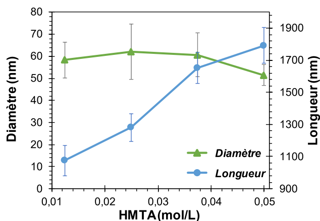
Figure III-4. Influence de la concentration en HMTA sur le diamètre et la longueur des nanofils de ZnO (0,025 M de Zn(NO_3)_2 à 90^\circ C pendant 4h et post recuit 30 min à 500^\circ C ).
