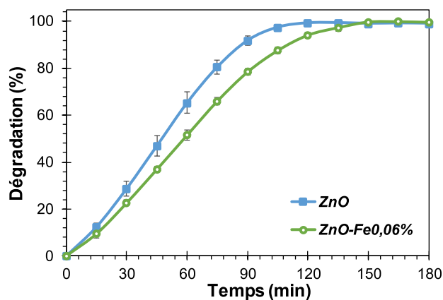
Figure V-13. Taux de dégradation de MO par photocatalyse sous lumière UV en présence de ZnO ou ZnO-Fe0,06% lors du cycle 1 ([MO] = 10 \mu\text{M} , V = 30 mL agité, \lambda \sim 365 \text{ nm} ).
