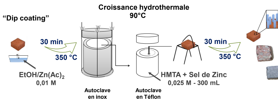
Figure II-3. Schéma de la synthèse hydrothermale pour les matériaux du génie civil.
