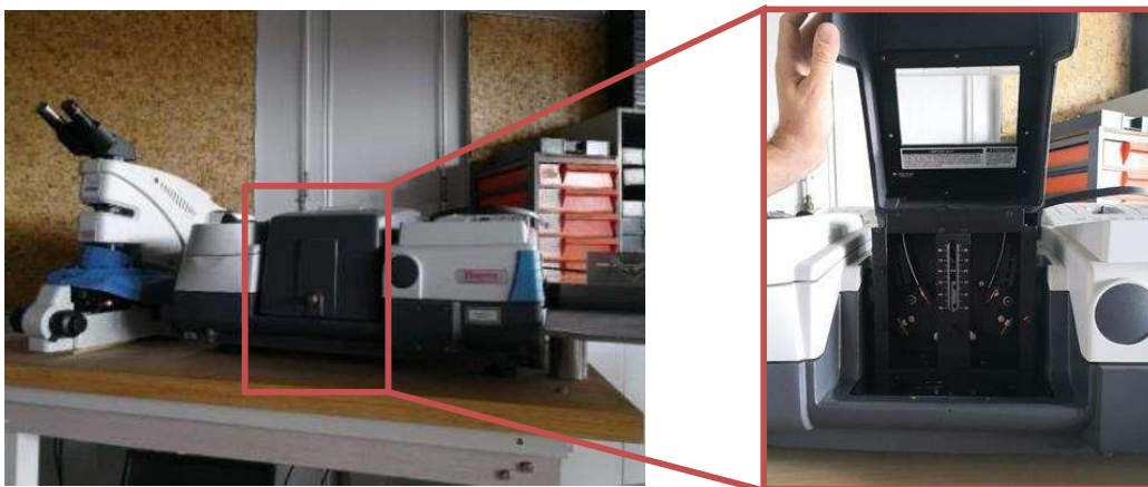
Figure II-10. Photo du FT-IR Nicolet 6700 (Thermo) utilisé à l'ICMPE.
