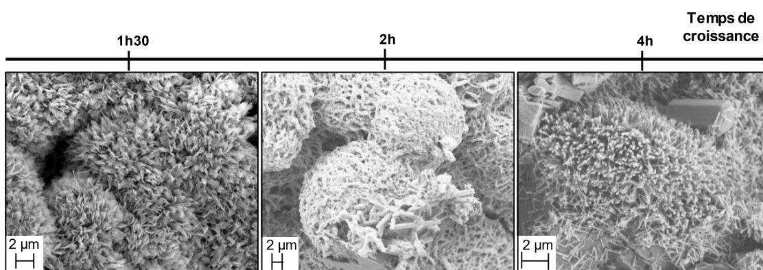
Figure IV-16. Images MEB des nanofils synthétisés sur les bétons pendant 1h30, 2h et 4h (0,025 M de Zn(NO_3)_2 et de HMTA à 90^\circ C et post recuit 30 min à 350^\circ C ) [12].
