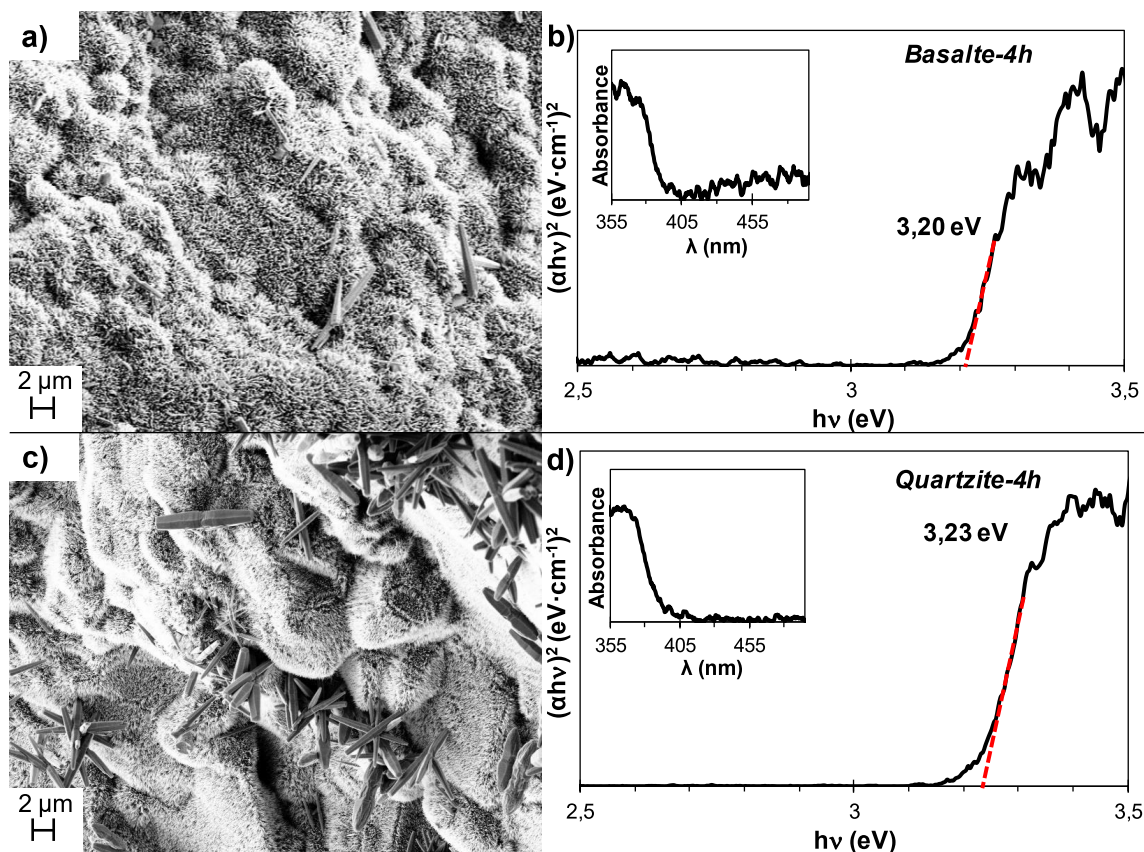
Figure VI-1. Images MEB et spectres d'absorbance UV-Visible transformés par le modèle de Tauc-Lorentz sur les basaltes (a,b) et sur les quartzites (c,d)(0,025 M de nitrate de zinc et de HMTA à 90°C pendant 4h et post recuit 30 min à 350°C).
