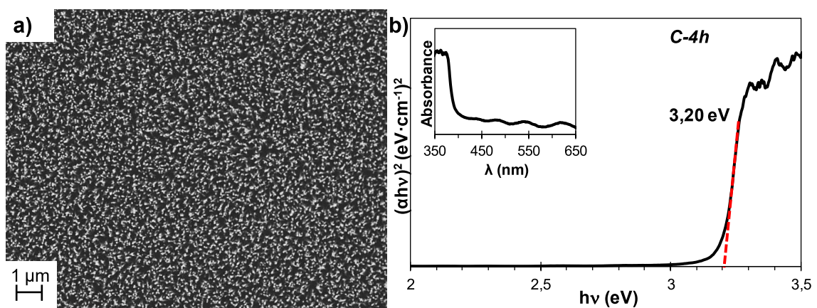
Figure IV-3. Image MEB (a) et spectre d'absorbance UV-Visible transformé par le modèle de Tauc-Lorentz (b) de C-4h (0,025 M de Zn(NO_3)_2 et de HMTA à 90°C pendant 4h et post recuit 30 min à 350°C) [11] .
