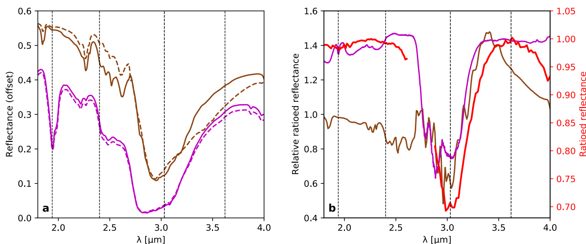
FIG. 5.19 : a. Spectres RELAB de jarosite (spectres marron, décalés verticalement de 0,1 pour la lisibilité) issus de deux régions différentes : Rublev (trait plein, JBA78) et St Léger (pointillés, JB701); ainsi que de gypse (spectres violets, JBE64) pour deux tailles de grains : < 45 \mu\text{m} (trait plein) et 45\text{--}90 \mu\text{m} (pointillés). Ces spectres issus de la base de données RELAB ont été téléchargés via la PDS spectral library (Milliken, 2020).
