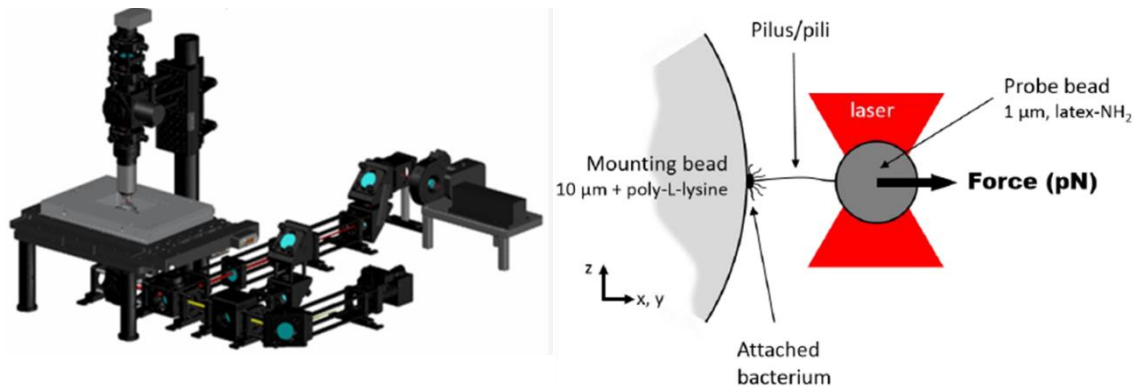
Figure 12 : Dispositif de la pince optique et configuration expérimentale pour l'étude des pili de L. lactis à l'échelle de la molécule unique (Castelain et al. 2016a).
