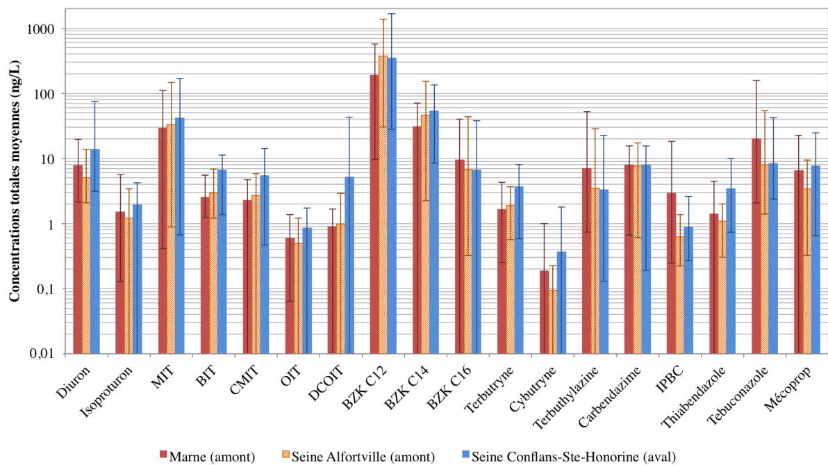
FIGURE 60 – Concentrations totales moyennes mesurées dans les eaux de rivière de l'agglomération parisienne (n=10). Les barres d'erreur représentent les valeurs minimales et maximales mesurées.
