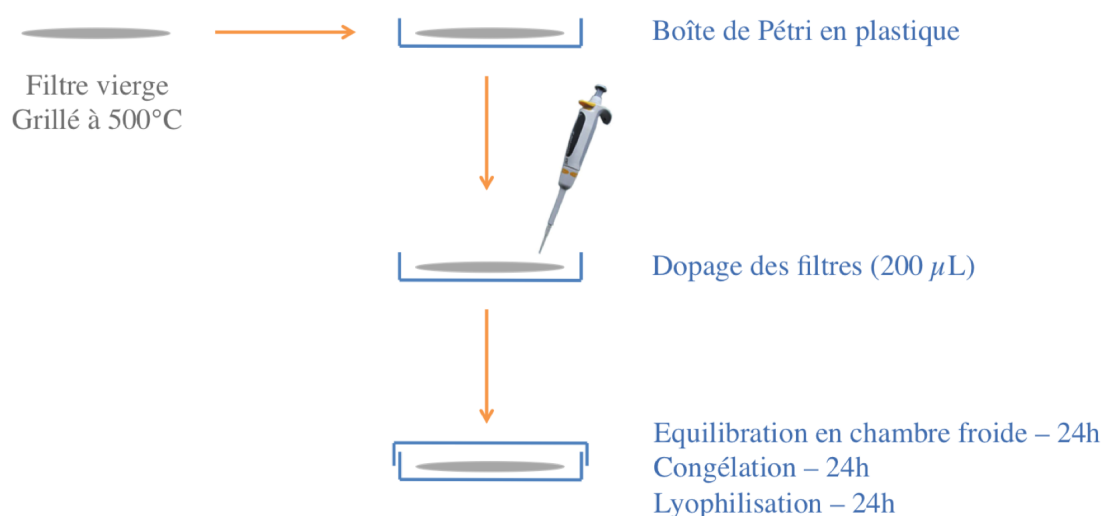
FIGURE 21 – Protocole de dopage des filtres vierges pour la détermination des rendements d'extraction MAE.
