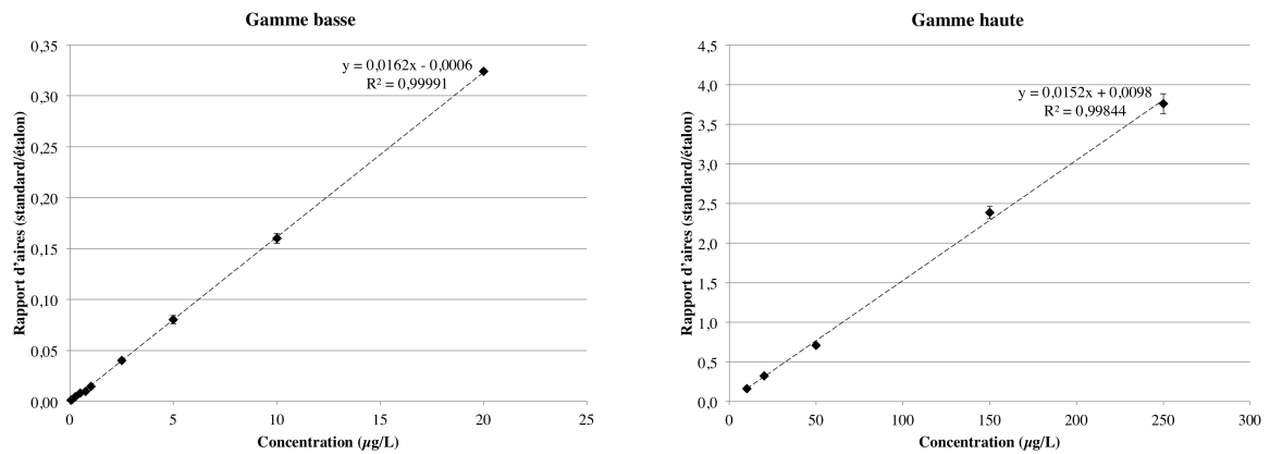
FIGURE 16 – Droites d'étalonnage de l'isoproturon obtenues avec les cinq répétitions de gammes
