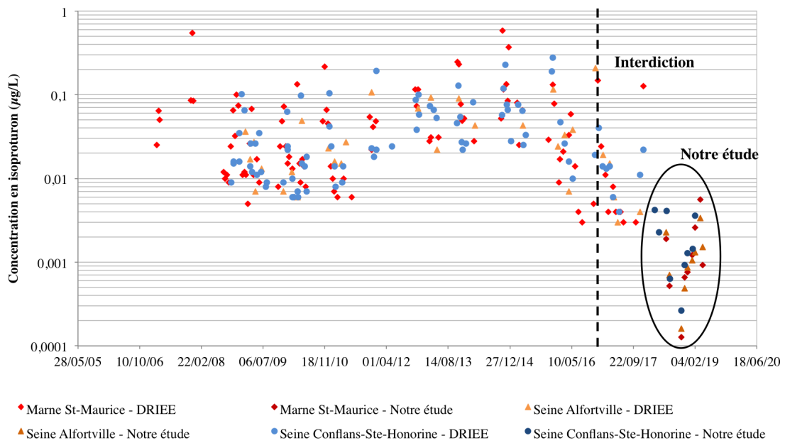
FIGURE 59 – Évolution de la concentration de l’isoprothuron en fraction dissoute des eaux de surface de la Marne et de la Seine depuis 2005.
