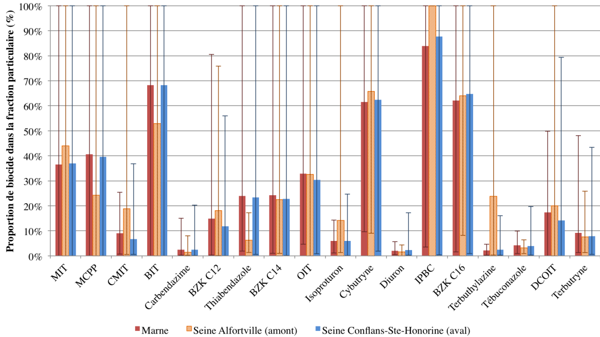
FIGURE 63 – Proportions particulières moyennes des biocides dans les échantillons d’eau de surface de la Marne et de la Seine (n=10). Les barres d’erreur représentent les valeurs minimales et maximales calculées.
