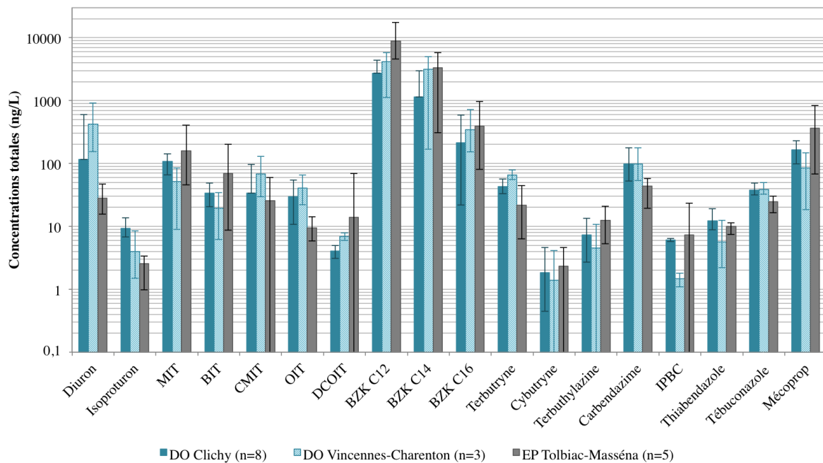
FIGURE 50 – Concentrations totales moyennes dans les RUTP échantillonnés. Les barres d'erreur représentent les concentrations minimales et maximales mesurées.
