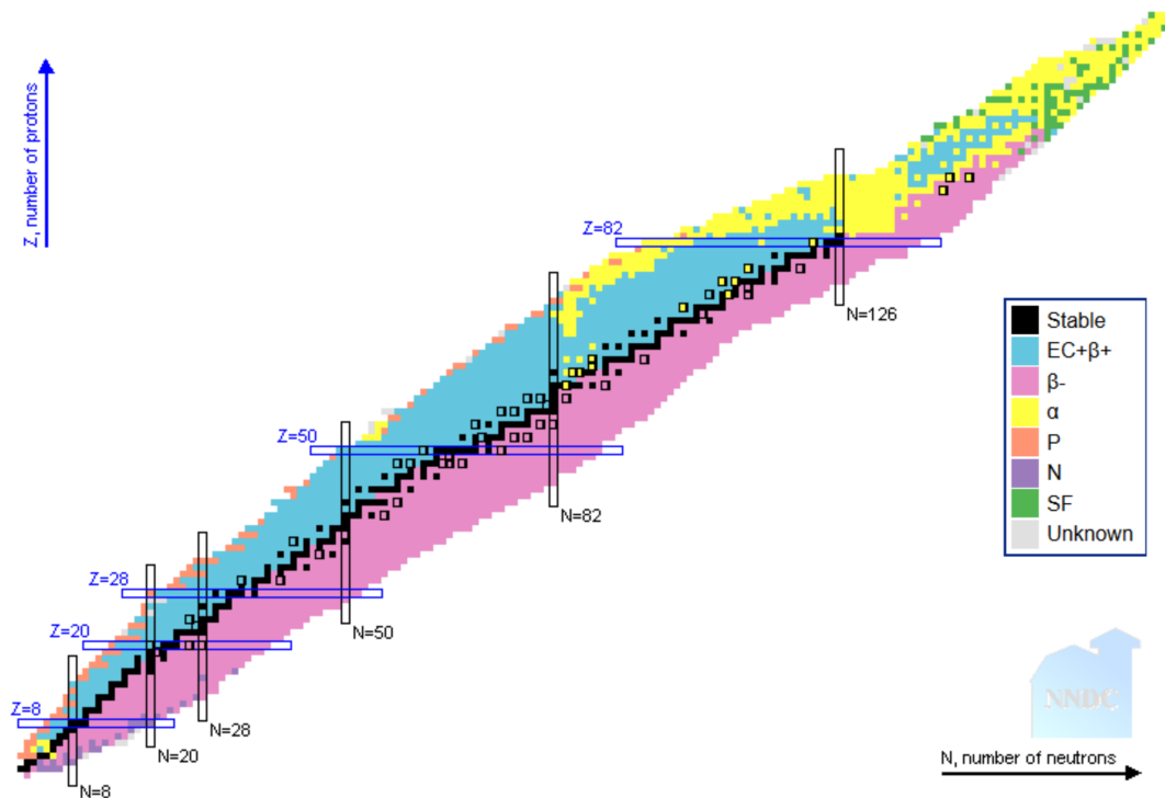
FIGURE 1.1 – Vallée de stabilité. La plupart des noyaux connus sont représentés en fonction de leur nombre de neutrons (abscisse) et de leur nombre de protons (ordonnée). Le code couleur désigne la stabilité ou le mode de désintégration : EC+ \beta^+ désigne la désintégration par capture électronique ou par processus \beta^+ , \beta^- la désintégration par processus \beta^- , \alpha la désintégration par processus \alpha , P désigne la désintégration par émission de proton, N la désintégration par émission de neutron, et SF la fission spontanée. La figure est issue du National Nuclear Data Center ( https://www.nndc.bnl.gov/nudat2/ ).
