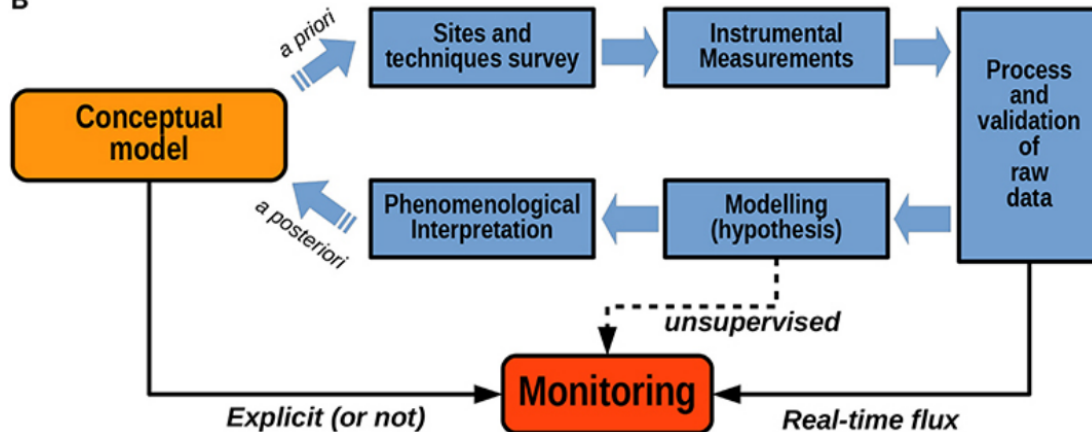
FIGURE 0.1 – Processus de recherche dans le contexte de la volcanologie d’après Beauducel et al. (2020).
