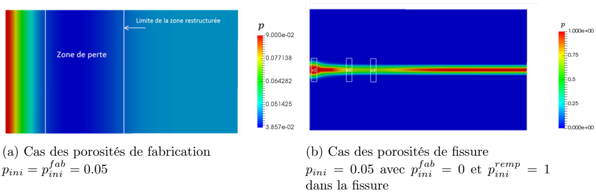
FIGURE II.3.9 – Évolution de la fraction volumique de porosité sous gradient thermique imposé (attention aux échelles différentes)
