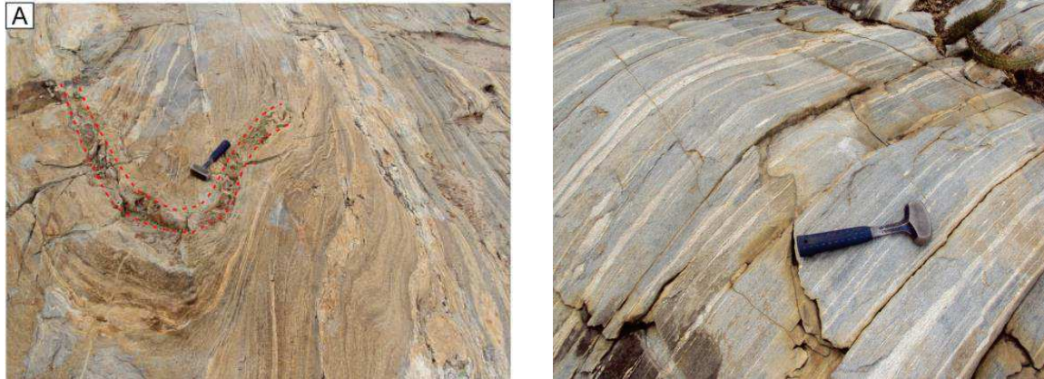
Figura 31 : Rochas do Complexo Jáguaetama. A) Metatexito com níveis de rocha cálcio-silicática (tracejado em vermelho). B) Ortognaisse de composição granítica milonitizado. Fonte: Pinéo, 2017
