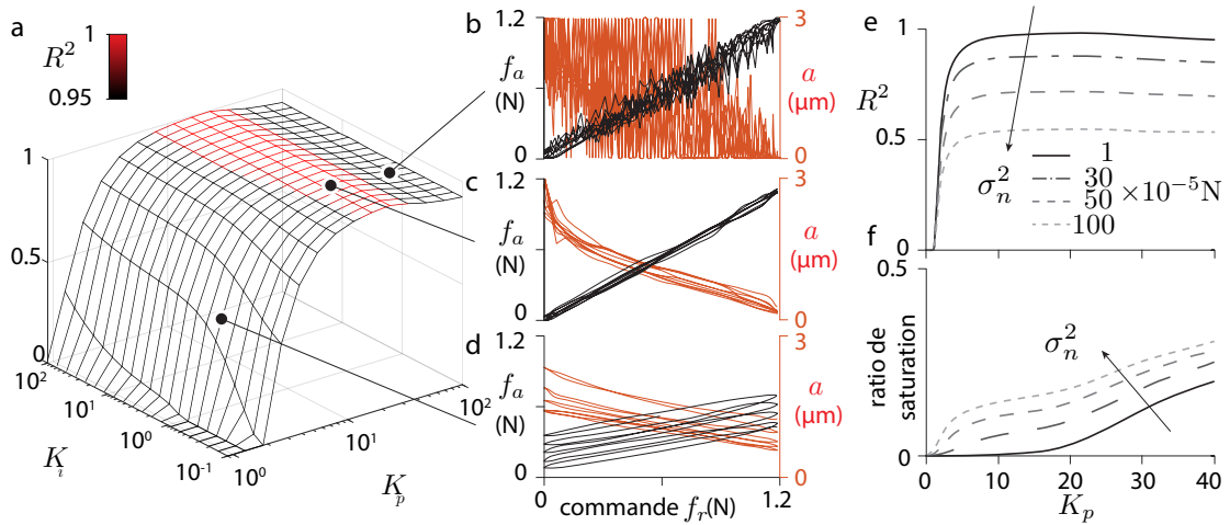
FIGURE 3.2 – a . La fidélité du contrôle est donnée par le paramètre R^2 en comparant f_a = f_r pour chaque couple de coefficients K_i and K_p . b . K_i = 2 et K_p = 40 . Signal sur-correcté, résultant en l’ajout non-négligeable de bruit c . K_i = 2 et K_p = 10 . L’équilibre parfait entre convergence rapide et peu de bruit. d . K_i = 2 et K_p = 1 . Gain faible donnant peu de satisfaction dans la correction de la perturbation. e . Effet du bruit du capteur sur la précision du contrôle. f . Effet du bruit du capteur sur la saturation du contrôleur.
