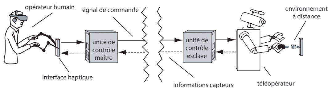
FIGURE 2.5 – L'homme interagit avec l'interface haptique, les commandes sont transmises au robot téléopérateur par les unités de contrôles pour agir sur l'environnement à distance. Adapté de (Passenberg et al., 2010)
