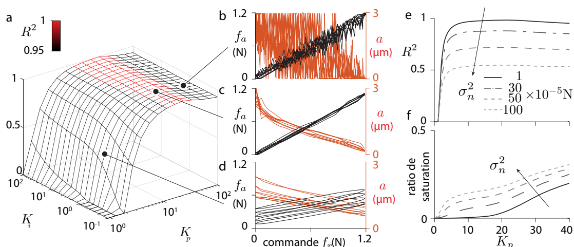
FIGURE 3.2 – a. La fidélité du contrôle est donnée par le paramètre R^2 en comparant f_a = f_r pour chaque couple de coefficients K_i and K_p . b. K_i = 2 et K_p = 40 . Signal sur-corrigé, résultant en l’ajout non-négligeable de bruit c. K_i = 2 et K_p = 10 . L’équilibre parfait entre convergence rapide et peu de bruit. d. K_i = 2 et K_p = 1 . Gain faible donnant peu de satisfaction dans la correction de la perturbation. e. Effet du bruit du capteur sur la précision du contrôle. f. Effet du bruit du capteur sur la saturation du contrôleur.
