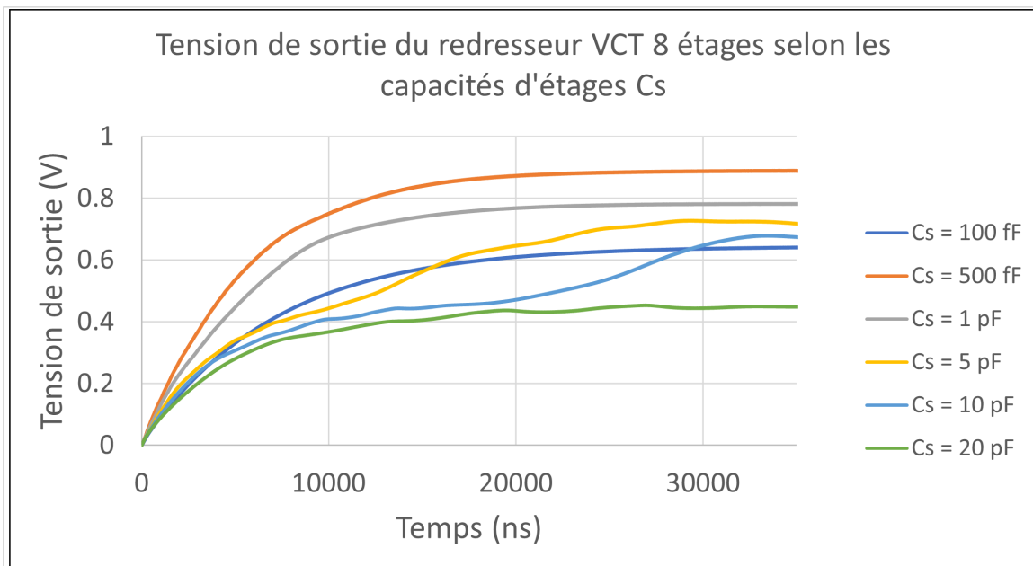
FIGURE 83 – Impact des capacités d'étage sur la tension de sortie du redresseur VCT 8 étages
