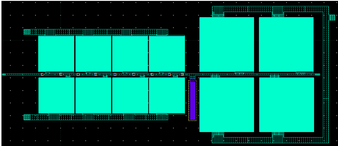
FIGURE 70 – Visualisation post-layout de la pompe de charge
