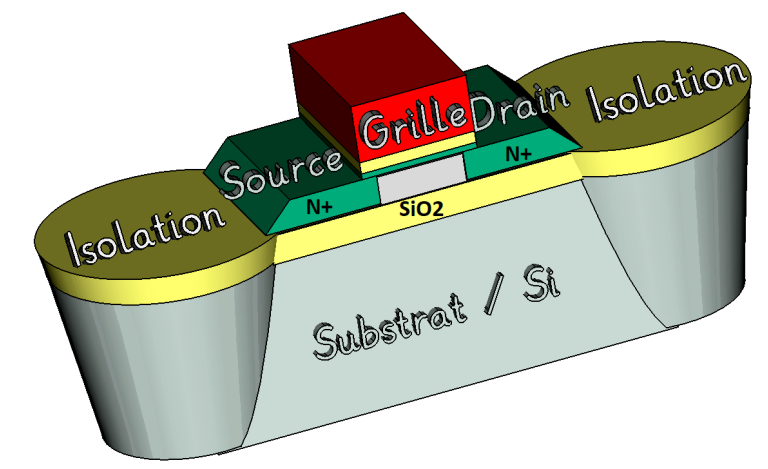
FIGURE 13 – Vue en coupe d'un transistor en technologie CMOS FDSOI
