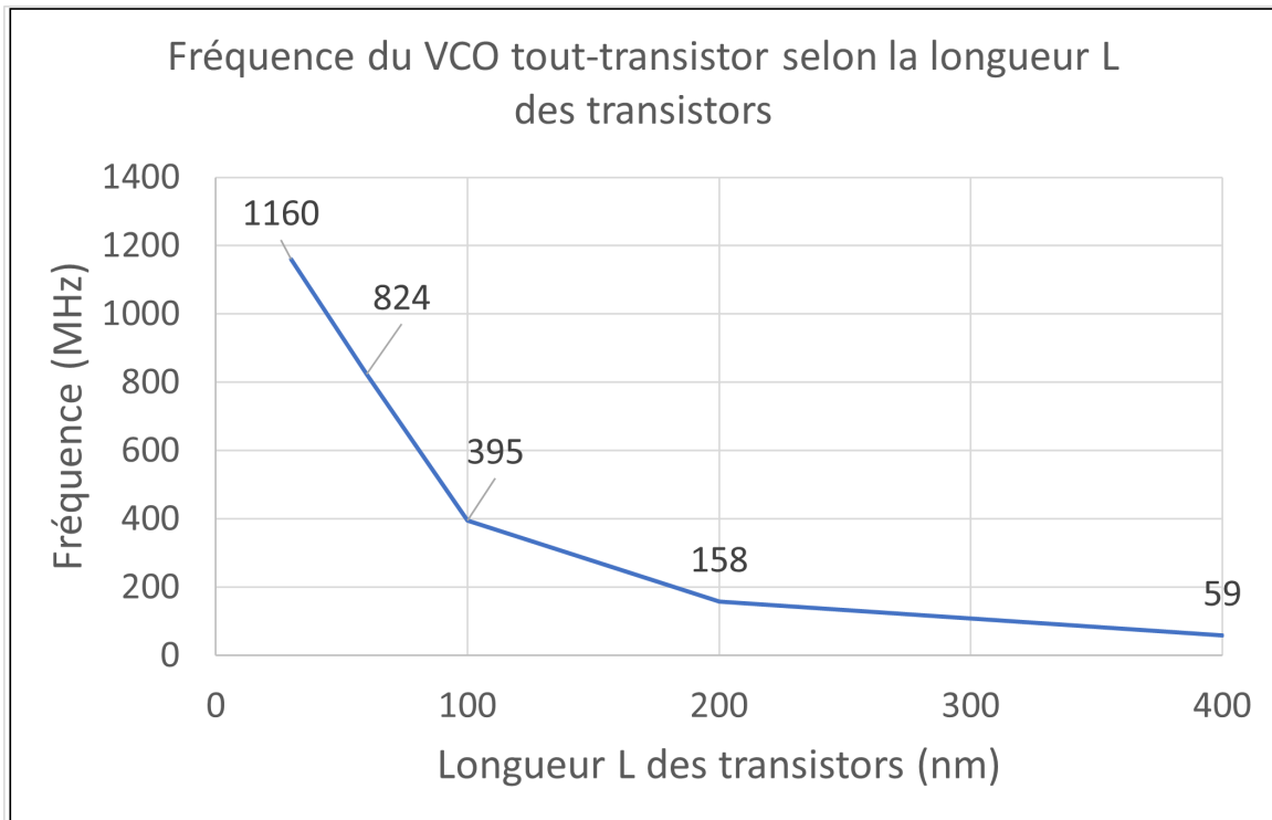
FIGURE 75 – Impact de la longueur L des transistors sur la fréquence du VCO
