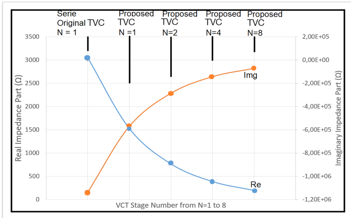
FIGURE 87 – Impact de la structure proposée (TVC = VCT) et du nombre d'étage du redresseur VCT sur l'impédance d'entrée [89]
