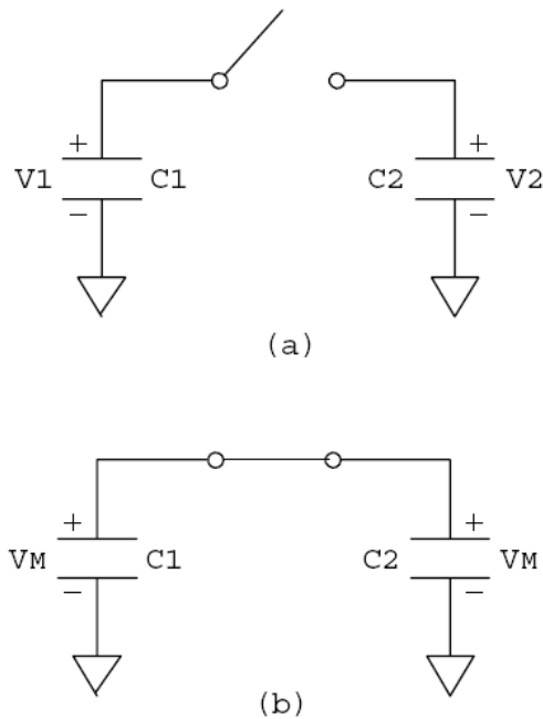
FIGURE 122 – Mise en parallèle de capacités chargées différentes [85]
