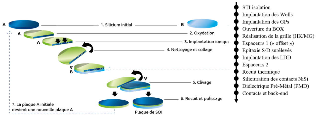
FIGURE 17 – Étapes détaillées de fabrication d'un transistor en FDSOI [25]
