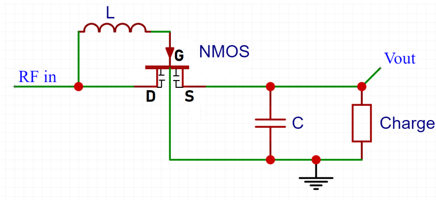
FIGURE 41 – Schéma d'un redresseur inductor-peak
