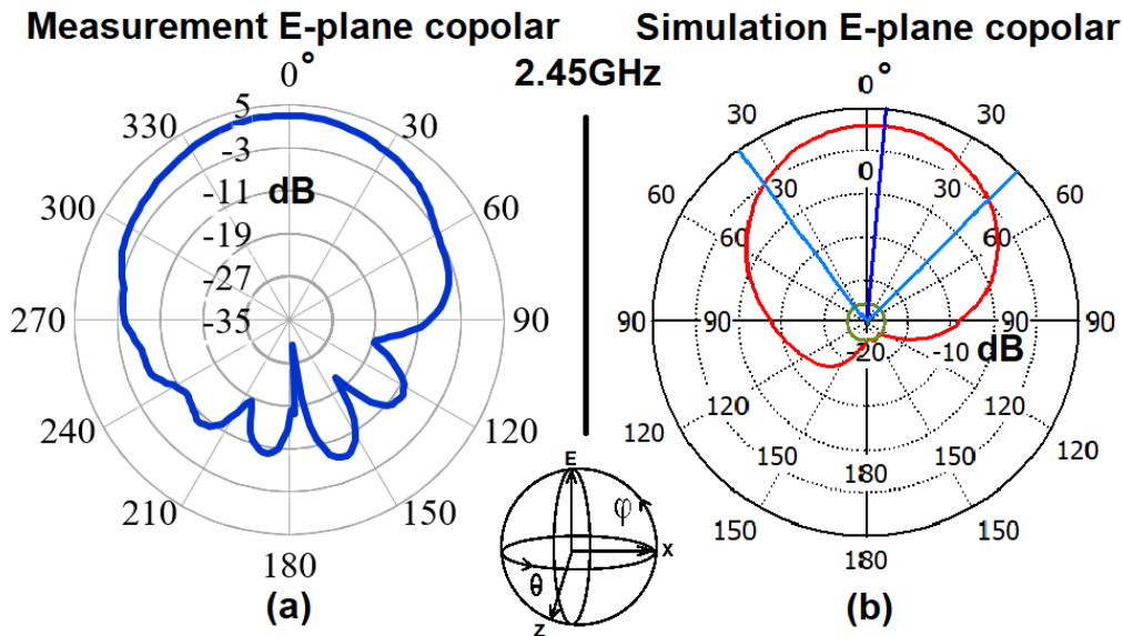
FIGURE 116 – Diagramme de polarisation au plan E en co-polarisation simulé et mesuré de l'antenne proposée
