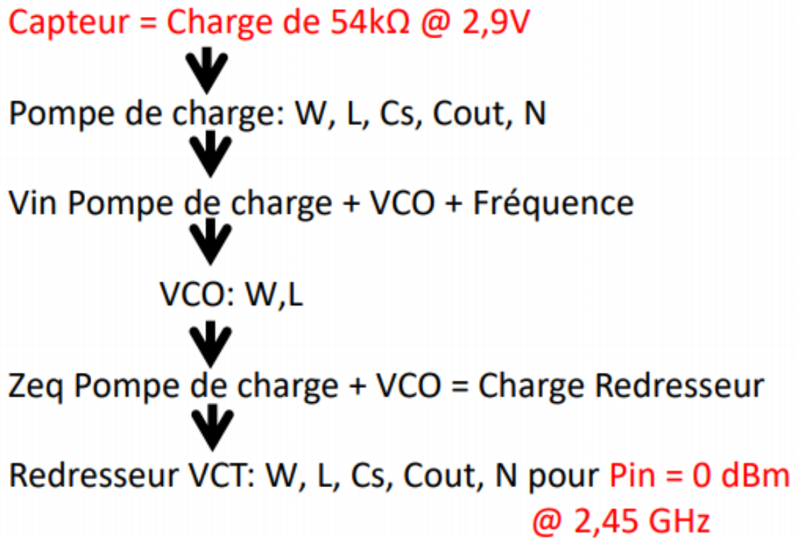
FIGURE 59 – Méthodologie de dimensionnement des paramètres des circuits proposés
