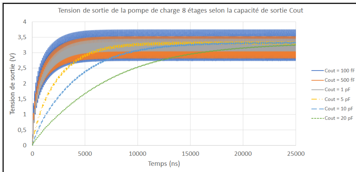
FIGURE 62 – Impact de la capacité de sortie sur la tension de sortie de la pompe de charge
