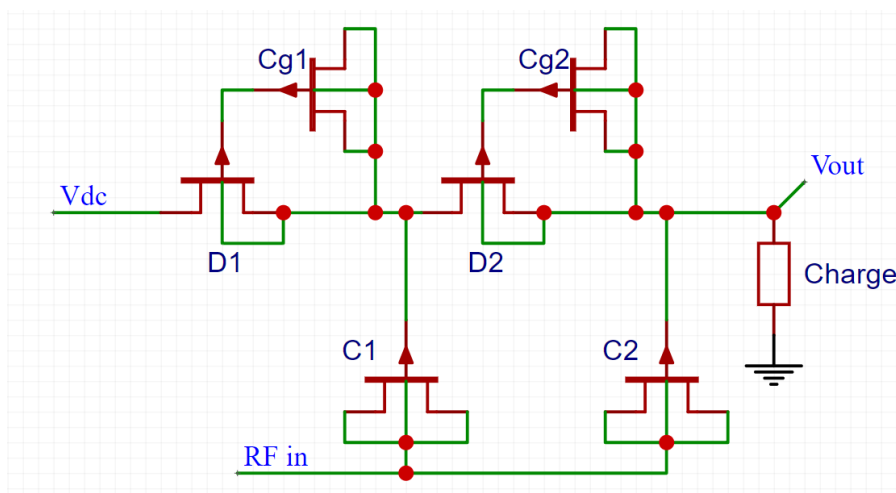
FIGURE 42 – Schéma d'un redresseur P-MOS à grille flottante
