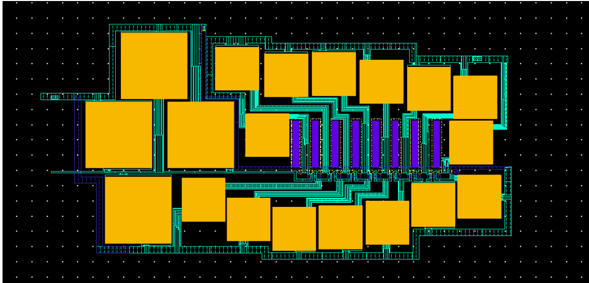
FIGURE 88 – Visualisation du layout et des parasites du redresseur VCT à 8 étages
