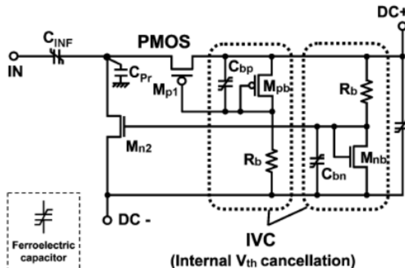
FIGURE 43 – Schéma de la technique de compensation de la tension seuil [54]
