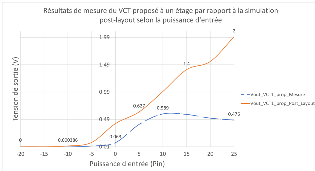
FIGURE 104 – Courbes comparatives des tensions de sortie des redresseurs VCT proposés en mesures et simulations selon la charge
