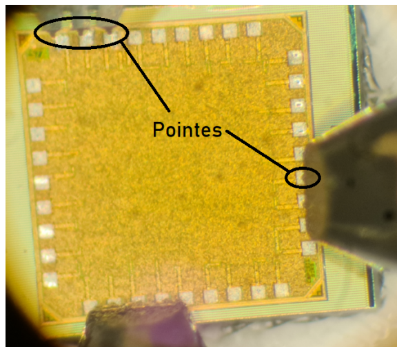
FIGURE 101 – Photographie des sondes posées sur la puce
