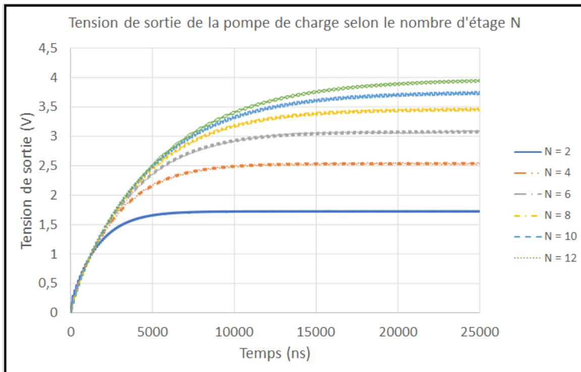
FIGURE 67 – Impact du nombre d'étage sur la tension de sortie de la pompe de charge
