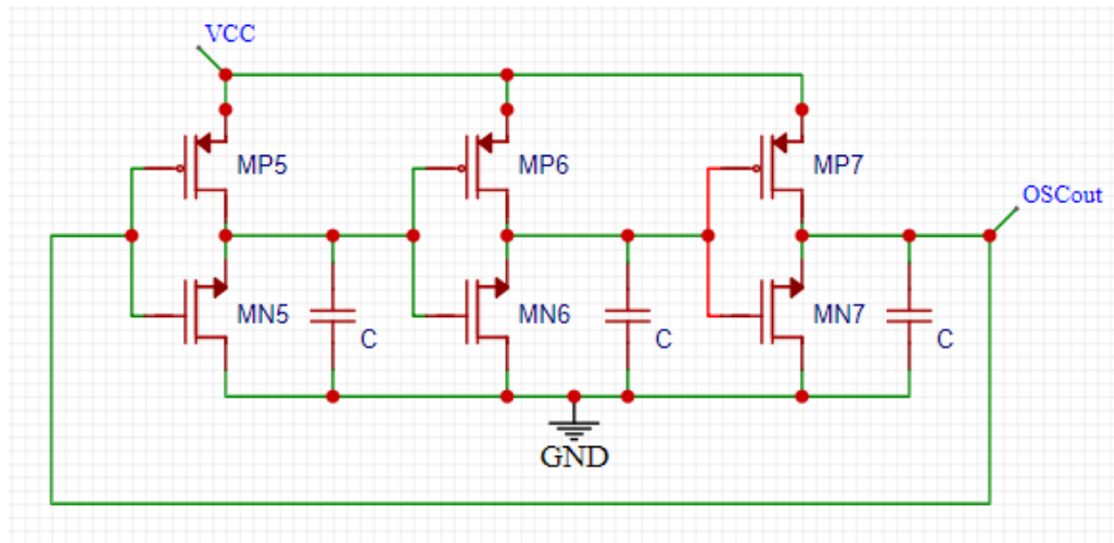
FIGURE 54 – Structure d'un oscillateur en anneau à base d'inverseurs et de capacités
