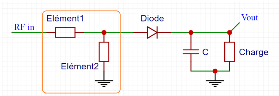
FIGURE 46 – Positionnement du circuit d'adaptation d'impédance devant un redresseur série n'en est pas de même en technologie intégrée où il faut prendre en compte l'espace physique nécessaire pour le réaliser en plus des effets parasites. Il faut également prendre en compte l'adaptation à 50 ohms des appareils de mesures.
