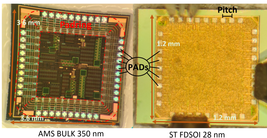
FIGURE 96 – Photographie de la surface des puces en BULK 350 nm et FDSOI 28 nm
