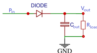
FIGURE 34 – Schéma d'un redresseur série
