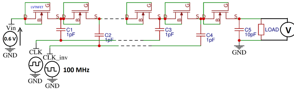
FIGURE 106 – Schéma de la pompe de charge proposée à 8 étages
