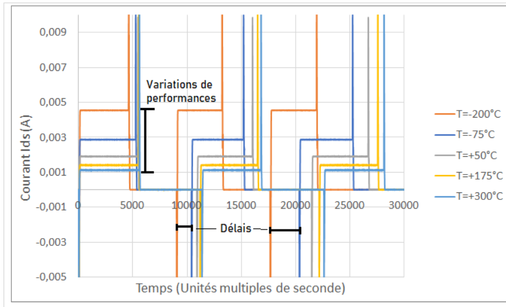
FIGURE 33 – Relevé du courant I_{ds} lors de la commutation du transistor NMOS selon la température
