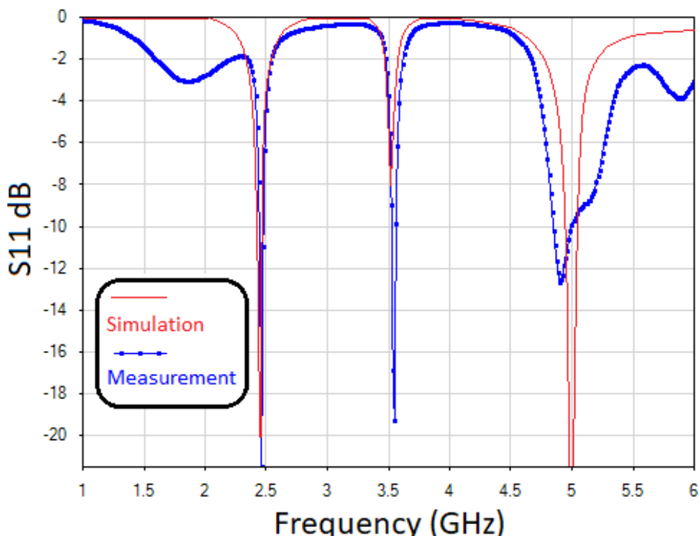
FIGURE 115 – Paramètre S11 de réflexion simulé et mesuré de l'antenne proposée
