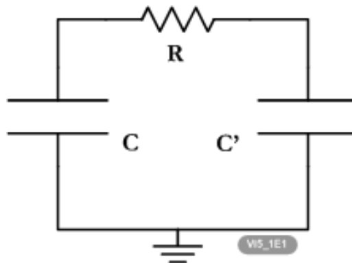
FIGURE 124 – Mise en parallèle par le biais d'une résistance [114]
