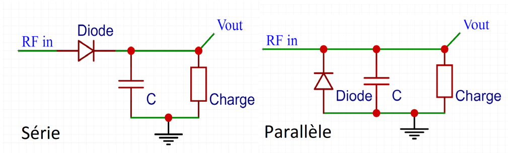
FIGURE 39 – Schéma des structures série et parallèle
