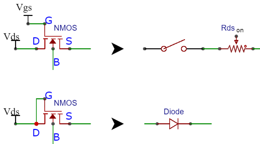
FIGURE 19 – Équivalence des modes de fonctionnement et connexions d'un transistor
