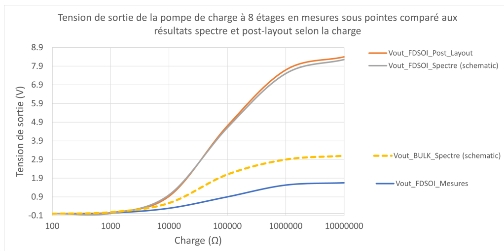
FIGURE 107 – Courbes comparatives des tensions de sortie de la pompe de charge à 8 étages proposée en mesures et simulations
