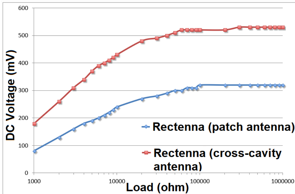
FIGURE 119 – Tension de sortie issues des rectennes avec l'antenne standard et proposée en cavité à croix
