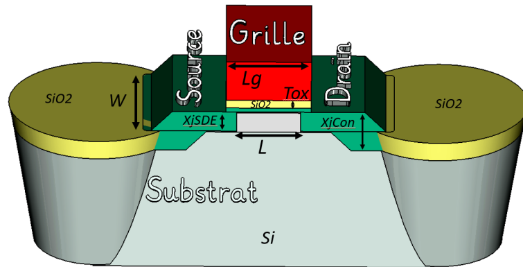
FIGURE 7 – Vue en coupe d'un transistor en technologie BULK
