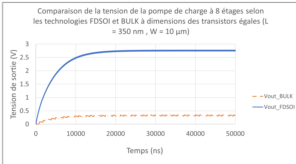
FIGURE 93 – Comparaison de la tension de sortie de la pompe de charge en FDSOI et BULK à dimensions égales pour V_{in} = 600 \text{ mV}
