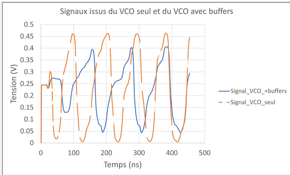
FIGURE 77 – Impact du rajout des buffers sur le signal générée par le VCO
