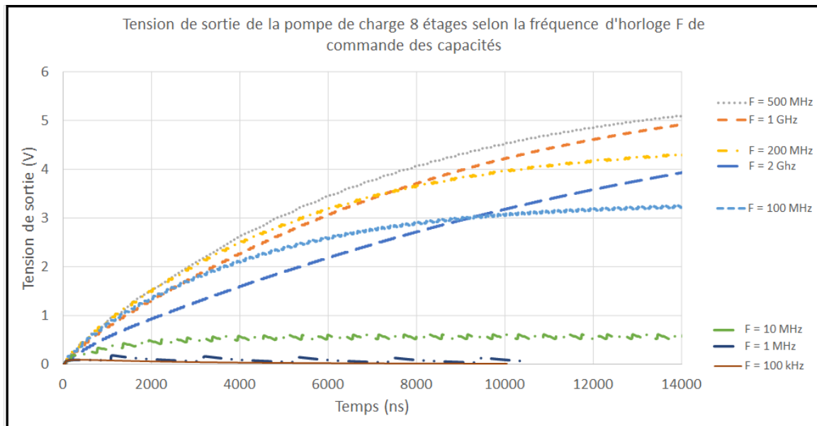
FIGURE 69 – Impact de la fréquence d'horloge sur la tension de sortie de la pompe de charge
