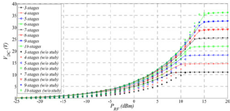
FIGURE 51 – limitation du nombre d'étage de la pompe de charge de Dickson [95]
