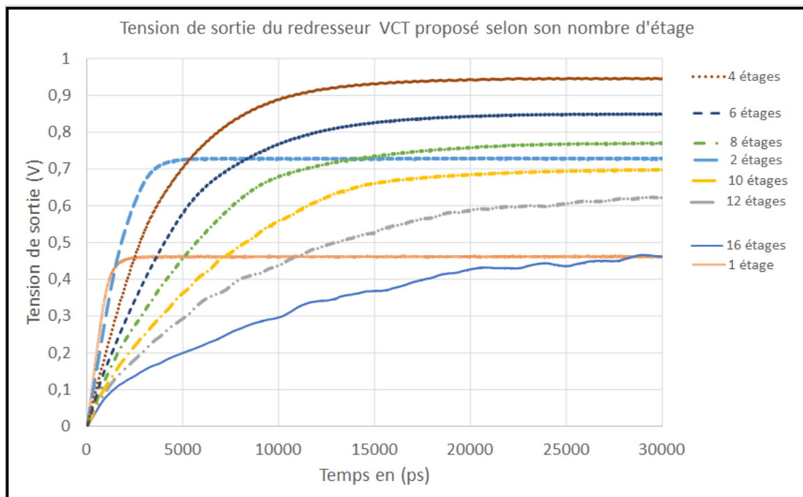
FIGURE 86 – Impact du nombre d'étage du redresseur VCT proposé sur la tension de sortie
