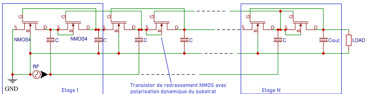
FIGURE 45 – Redresseur proposé avec technique d'annulation de la tension de seuil et polarisation du substrat
