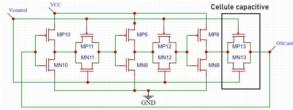
FIGURE 56 – Structure d'un oscillateur en anneau à base d'inverseurs et de cellule capacitives à transistors
