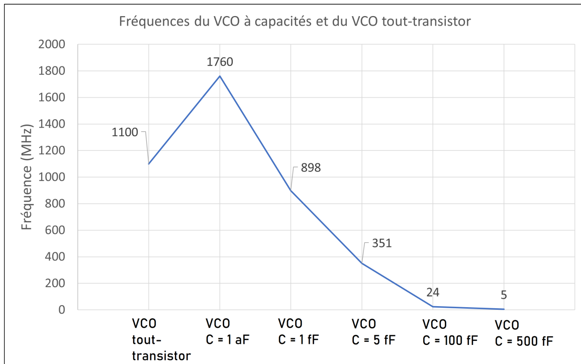
FIGURE 72 – Fréquences générées par le VCO tout-transistor et le VCO avec différentes valeurs de capacités
