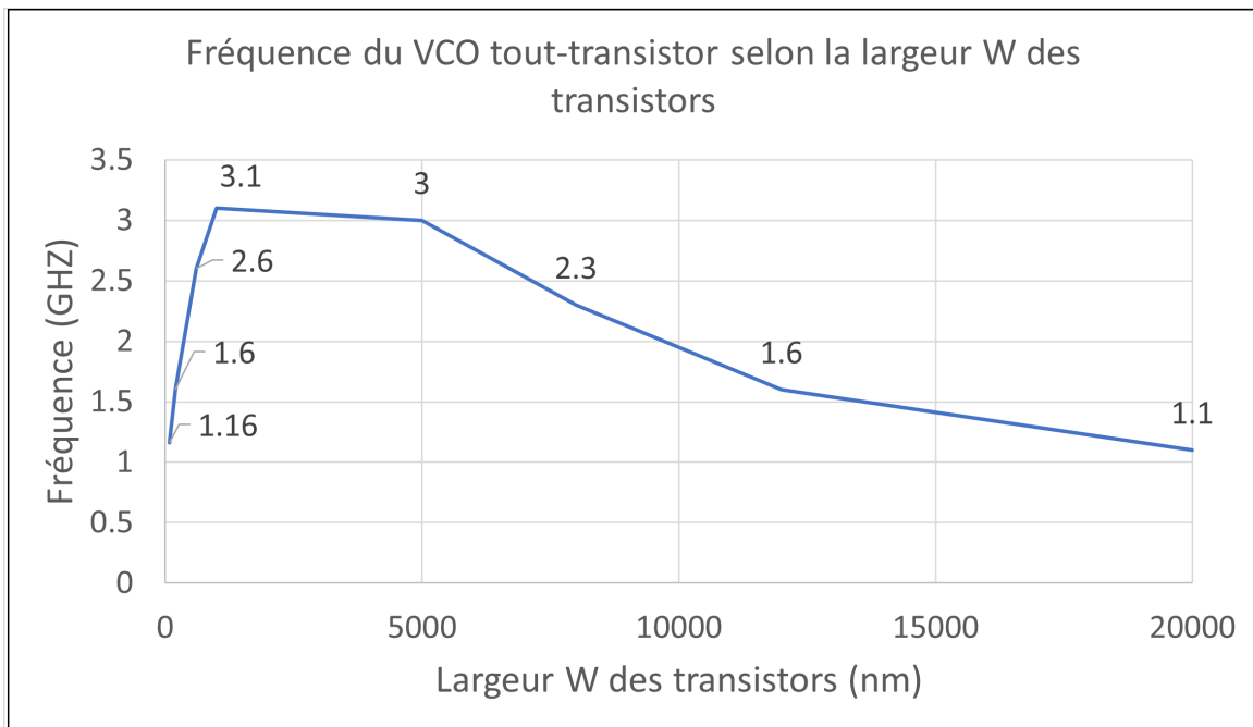
FIGURE 74 – Impact de la largeur W des transistors sur la fréquence du VCO
