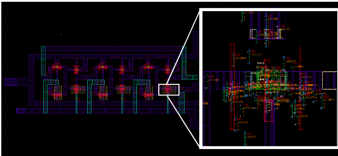
FIGURE 79 – Visualisation des parasites sur le VCO après la réalisation du layout.
