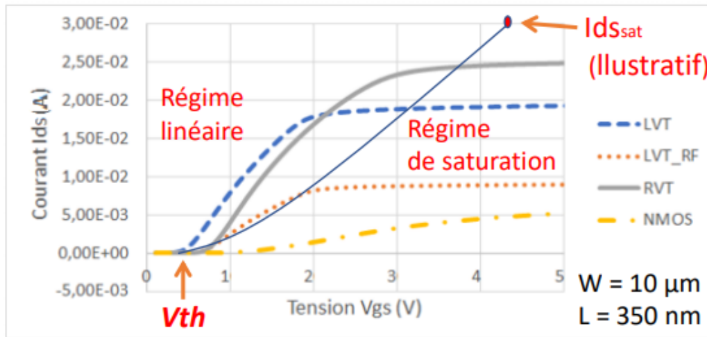
FIGURE 21 – Caractéristiques I_{ds}(V_{gs}) selon les transistors des technologies BULK et FDSOI avec les mêmes dimensions W = 10 \mu\text{m} et L = 350 \text{ nm}
