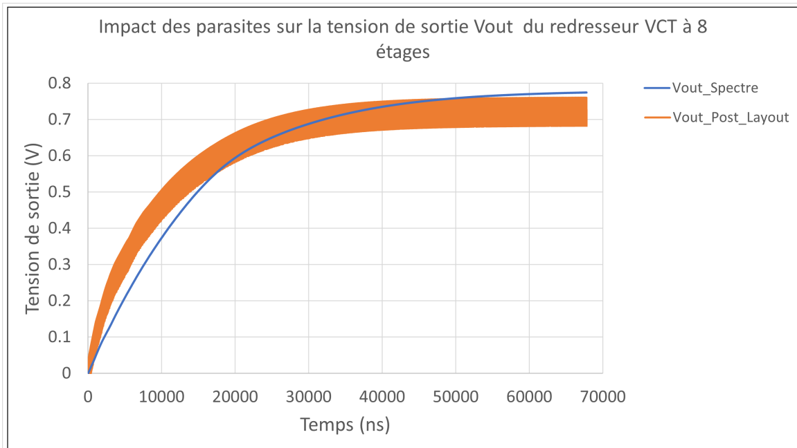
FIGURE 89 – Visualisation de la suppression des effets capacitifs par division de ligne du redresseur VCT à 8 étages
