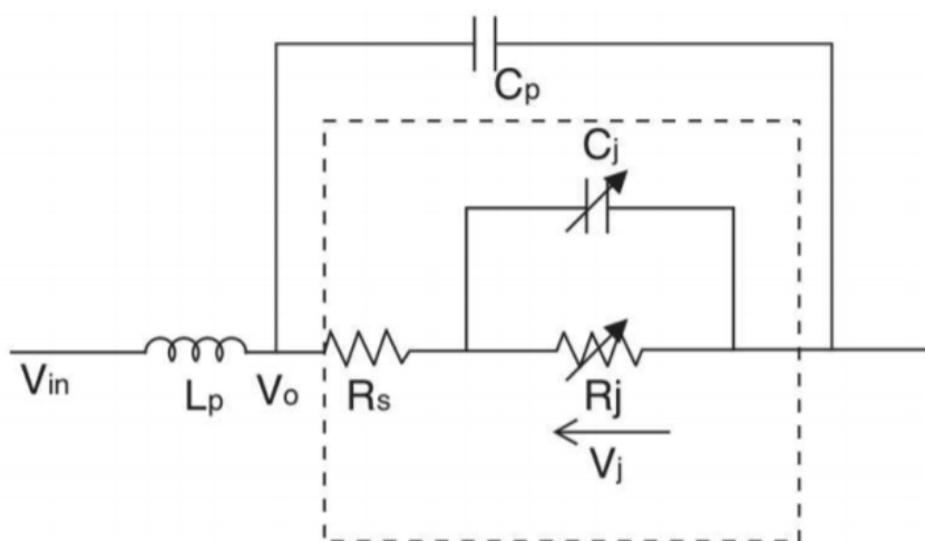
FIGURE 37 – Modèle parasitique de la diode [32]
