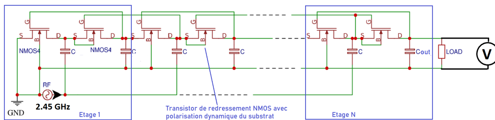
FIGURE 102 – Schéma du redresseur VCT proposé
