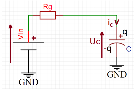
FIGURE 120 – Charge d'une capacité par un générateur et sa résistance
