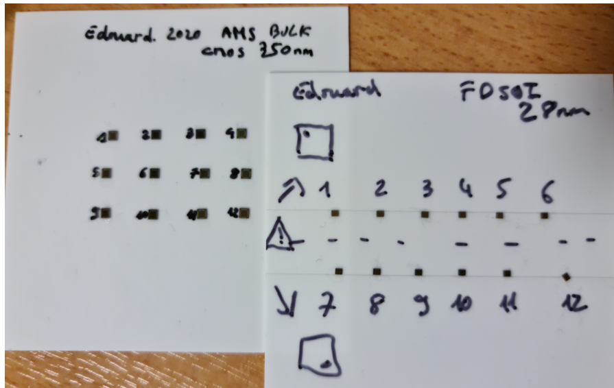
FIGURE 95 – Photographie des jeux de puces nues réalisées en BULK 350 nm par AMS et en FDSOI 28 nm par ST Microelectronics
