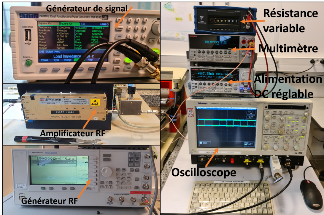
FIGURE 100 – Photographie des équipements nécessaires pour la mesure sous pointes
