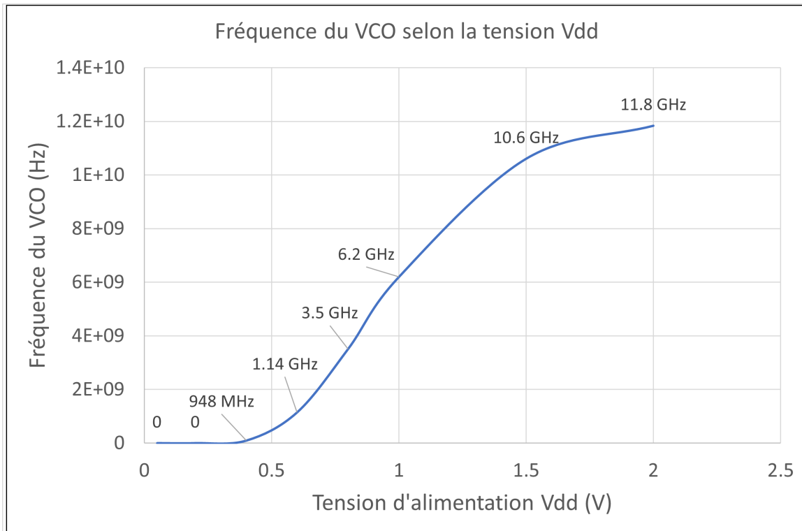
FIGURE 73 – Fréquence du VCO tout-transistor selon la tension Vdd injectée
