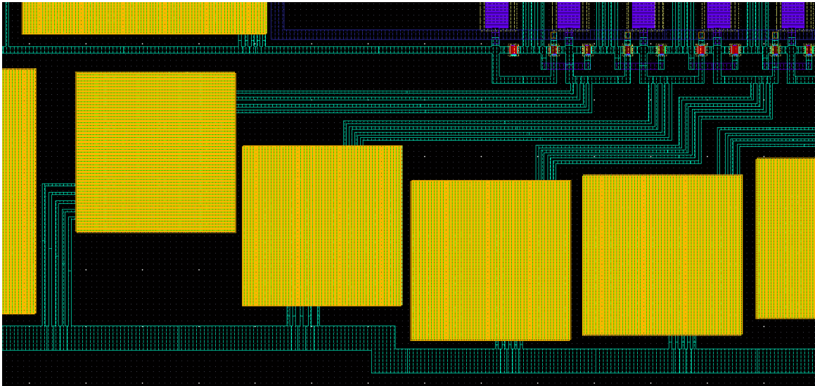
FIGURE 89 – Visualisation de la suppression des effets capacitifs par division de ligne du redresseur VCT à 8 étages
