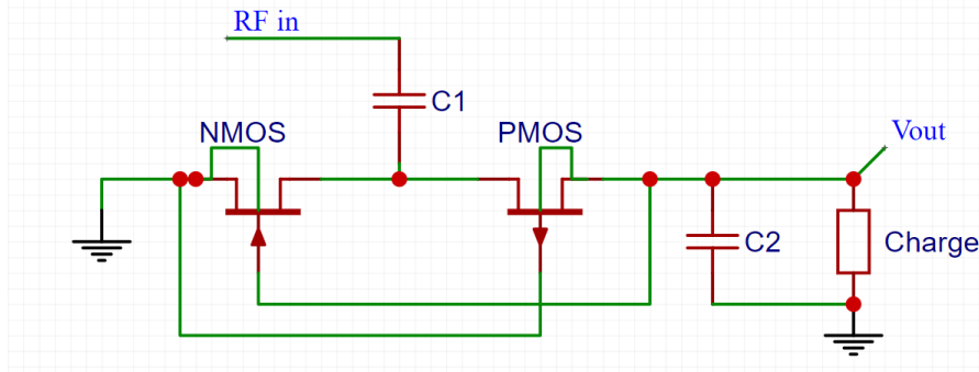
FIGURE 44 – Schéma d'un redresseur série avec technique de compensation autonome de tension seuil [57]
