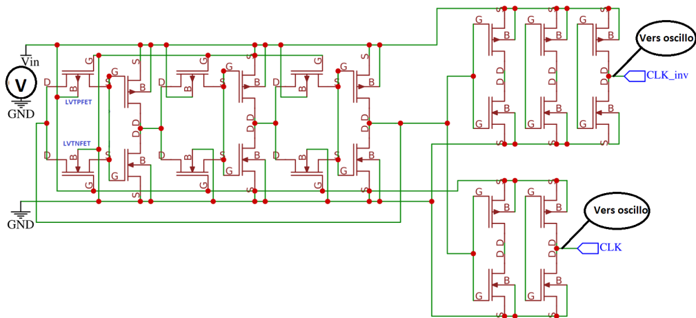
FIGURE 108 – Schéma complet du VCO proposé
