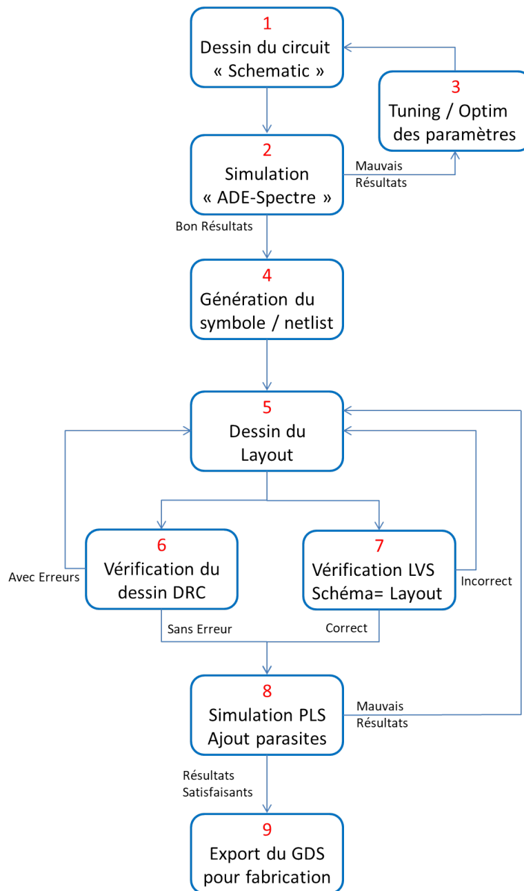
FIGURE 8 – Étapes de conception jusqu'à réalisation d'un circuit intégré
