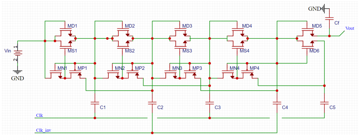
FIGURE 53 – Structure améliorée de Dickson NCP-2
