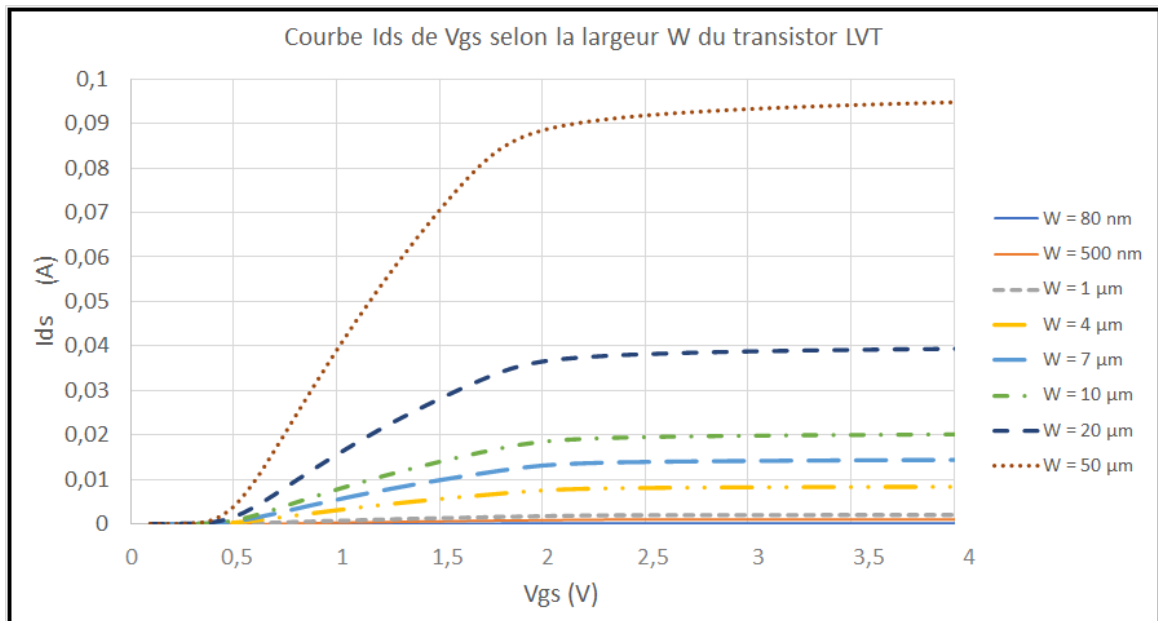
FIGURE 60 – Impact de la largeur du transistor monté en diode sur la caractéristique I_d(V_{ds})
