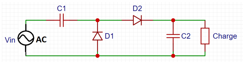
FIGURE 49 – Schéma du circuit de redressement de Greinacher, Cockroft et Walton
