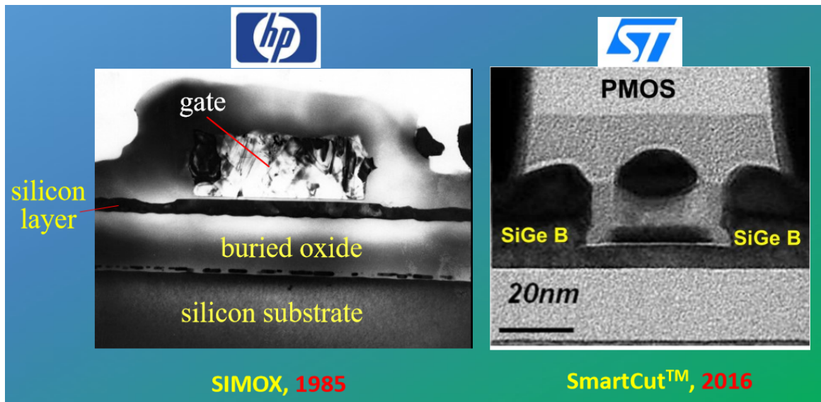
FIGURE 12 – Précision de la technique Smart Cut comparée au procédé SIMOX
