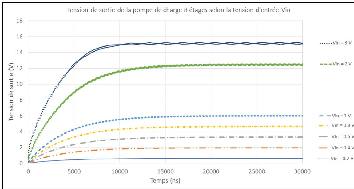
FIGURE 68 – Impact de la tension d'entrée sur la tension de sortie de la pompe de charge
