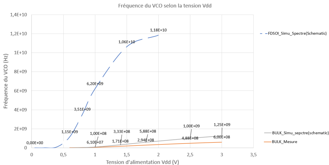
FIGURE 109 – Courbes comparatives des fréquences du VCO proposées selon la tension d'alimentation Vdd en mesures et simulations
