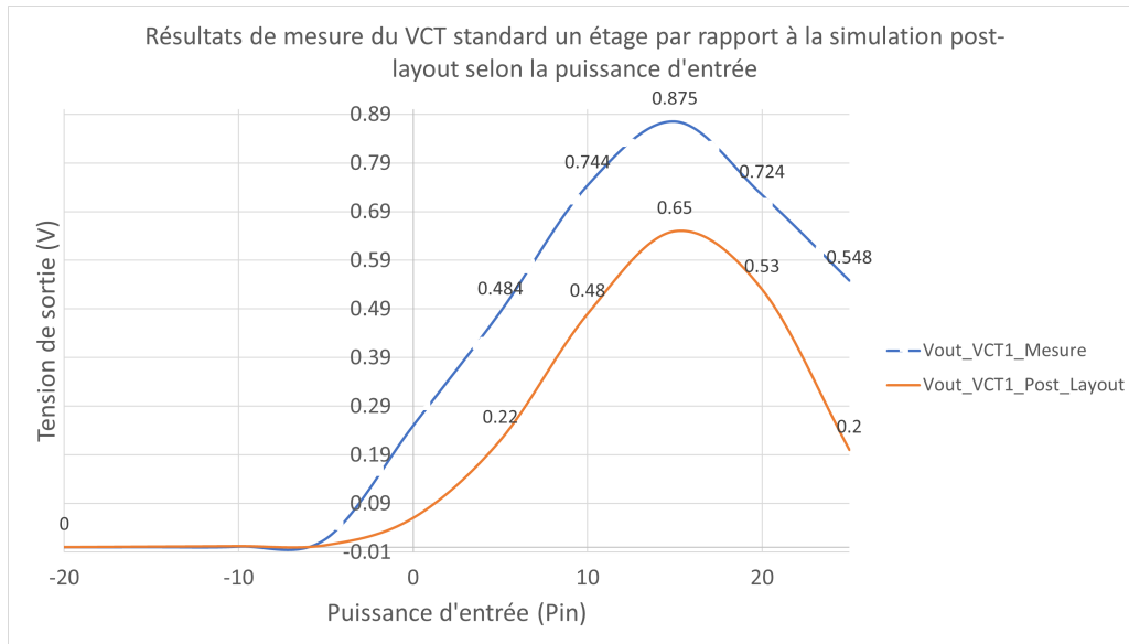
FIGURE 103 – Courbes comparatives des tensions de sortie des redresseurs VCT standards en mesures et simulations selon la charge
