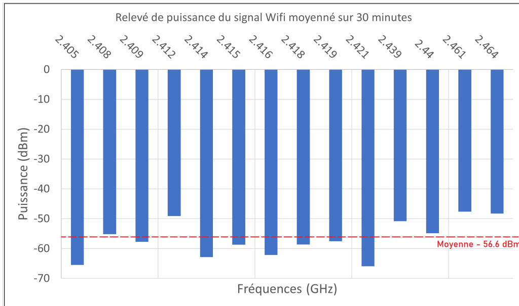
FIGURE 5 – Relevé des puissances moyennées sur 30 minutes à des fréquences proches de 2.45 GHz (soit la bande wifi, zigbee et bluetooth)
