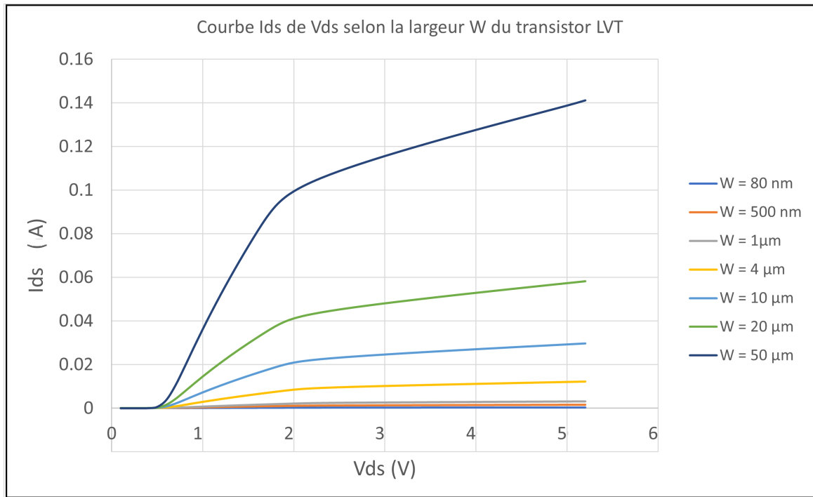
FIGURE 60 – Impact de la largeur du transistor monté en diode sur la caractéristique I_d(V_{ds})
