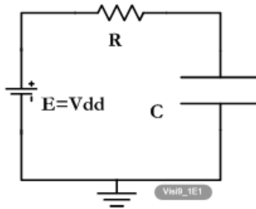
FIGURE 123 – Charge d'une capacité [85]
