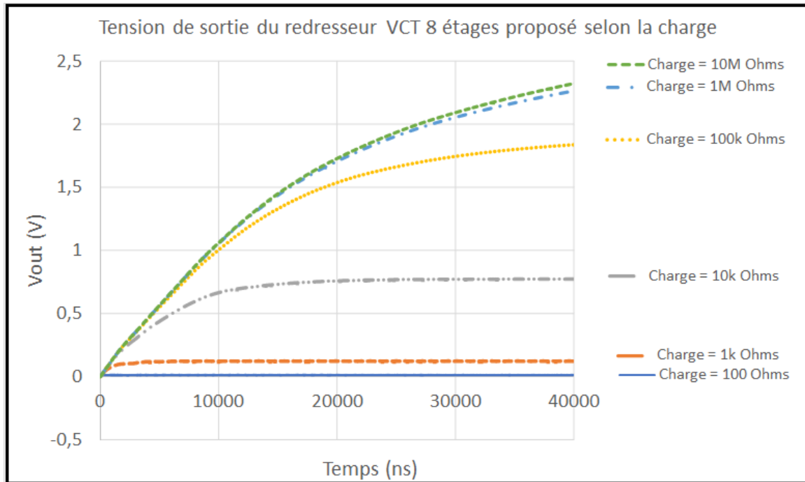
FIGURE 84 – Impact de la charge sur la tension de sortie du redresseur VCT à 8 étages
