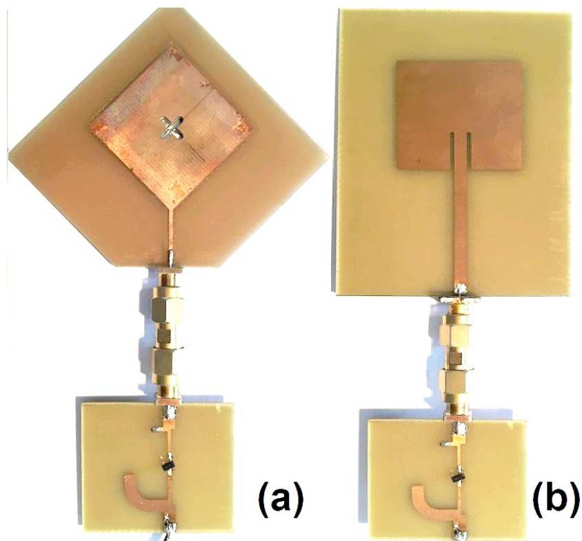
FIGURE 118 – Photographies des circuits de rectification réalisés en FR4 : (a) antenne double polarisation en croix. (b) patch standard rectangulaire.
