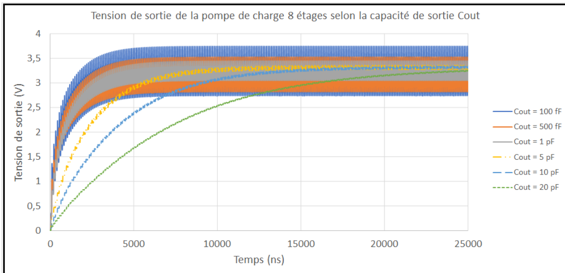
FIGURE 64 – Impact de la capacité de sortie sur la tension de sortie de la pompe de charge montrée sur la figure 65.
