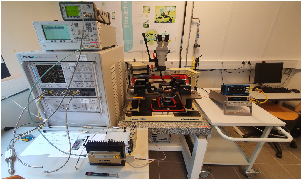
FIGURE 97 – Photographie du setup utilisé pour la mesure sous pointes des puces en BULK et FDSOI
