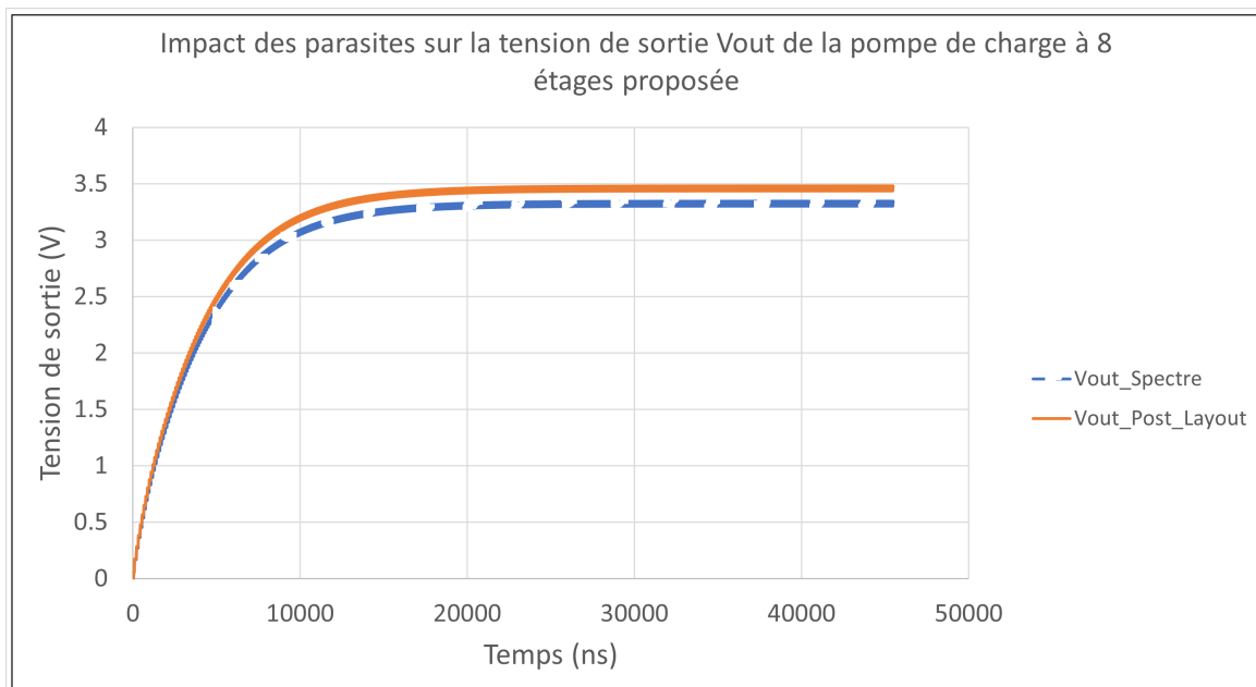
FIGURE 71 – Impact des parasites sur la tension de sortie de la pompe de charge
