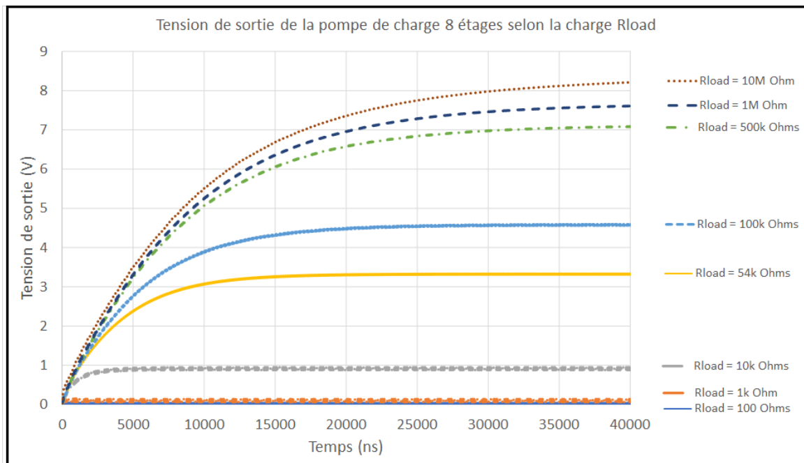
FIGURE 66 – Impact de la charge sur la tension de sortie de la pompe de charge
