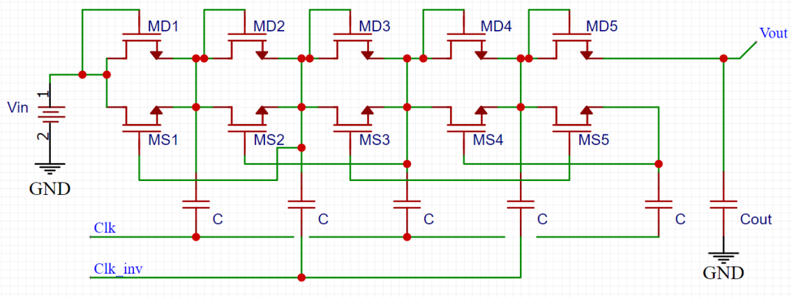
FIGURE 52 – Structure améliorée de Dickson NCP-1
