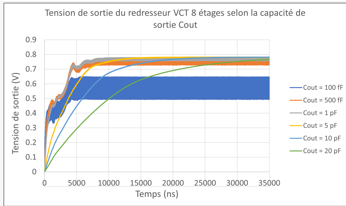
FIGURE 82 – Impact de la capacité de sortie sur la tension de sortie du redresseur VCT 8 étages et la qualité (pas oscillation) du signal. L'évolution de la tension de sortie du redresseur VCT selon C_s est montré sur la figure 83.
