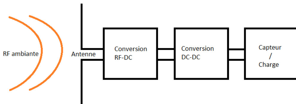
FIGURE 4 – Schéma bloc simplifié d'un système de récupération d'énergie RF
