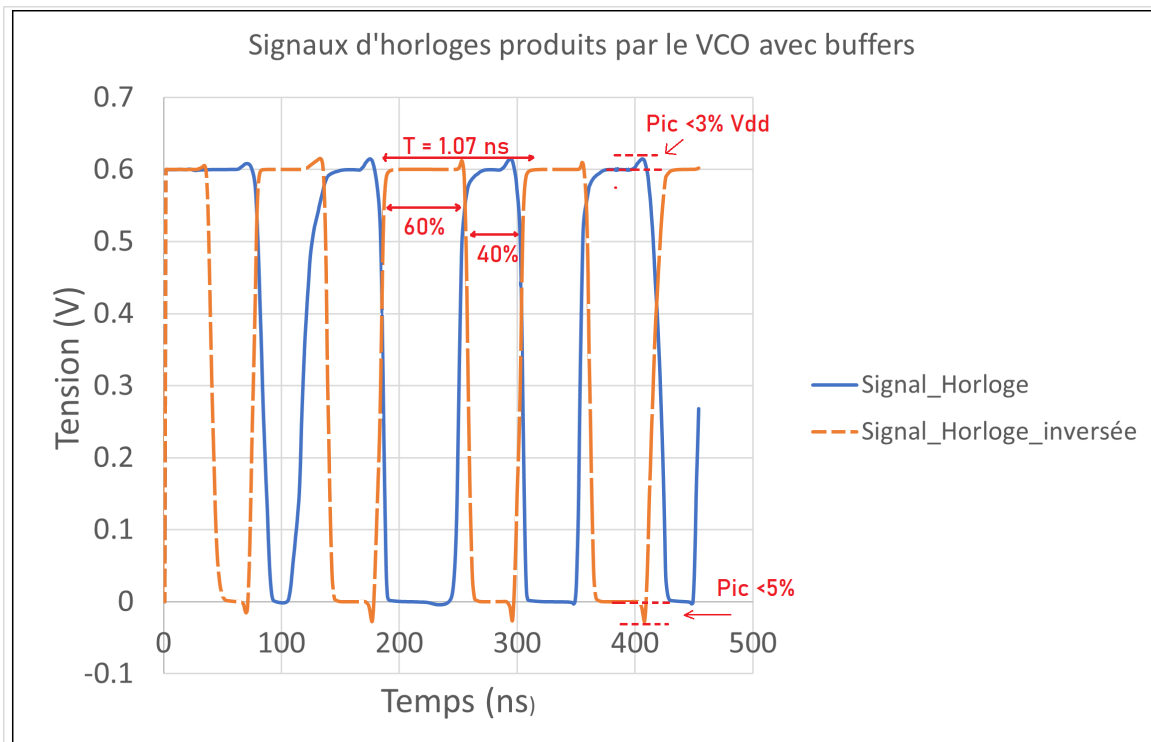
FIGURE 77 – Impact du rajout des buffers sur le signal générée par le VCO
