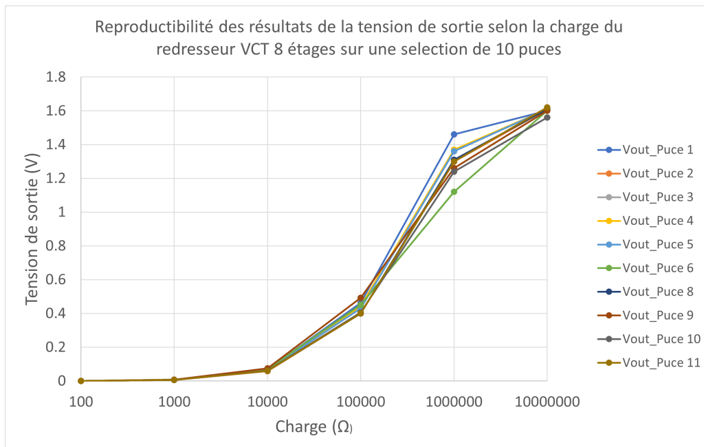
FIGURE 113 – Étude de la reproductibilité des résultats sur un jeu de 10 puces en mesurant la tension de sortie sur un circuit redresseur VCT
