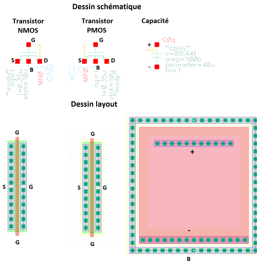
FIGURE 10 – Représentations schématiques et layout des transistors et d'une capacité en BULK 350 nm
