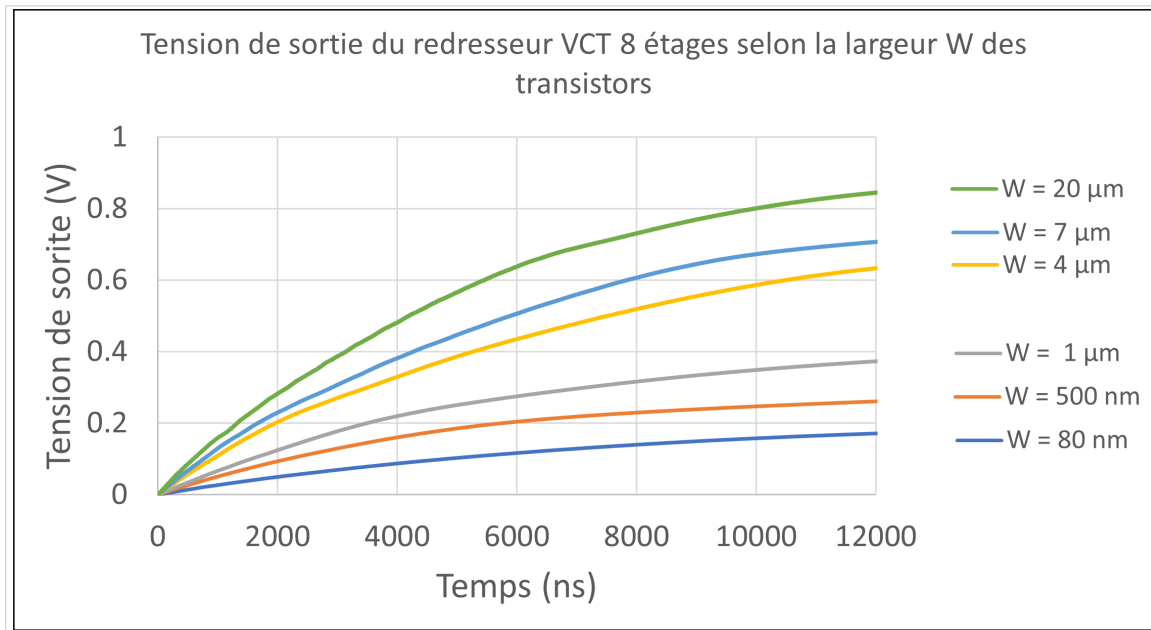
FIGURE 81 – Impact de la largeur du transistor sur la tension de sortie du redresseur VCT à 8 étages
