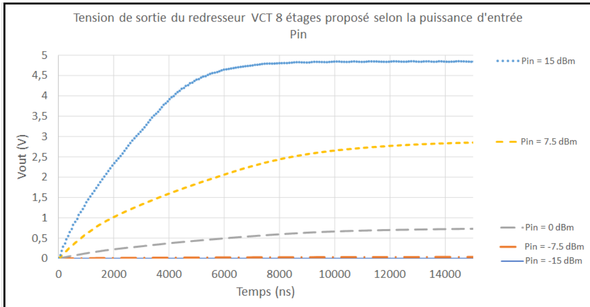
FIGURE 85 – Impact de la puissance d'entrée sur la tension de sortie du redresseur VCT à 8 étages
