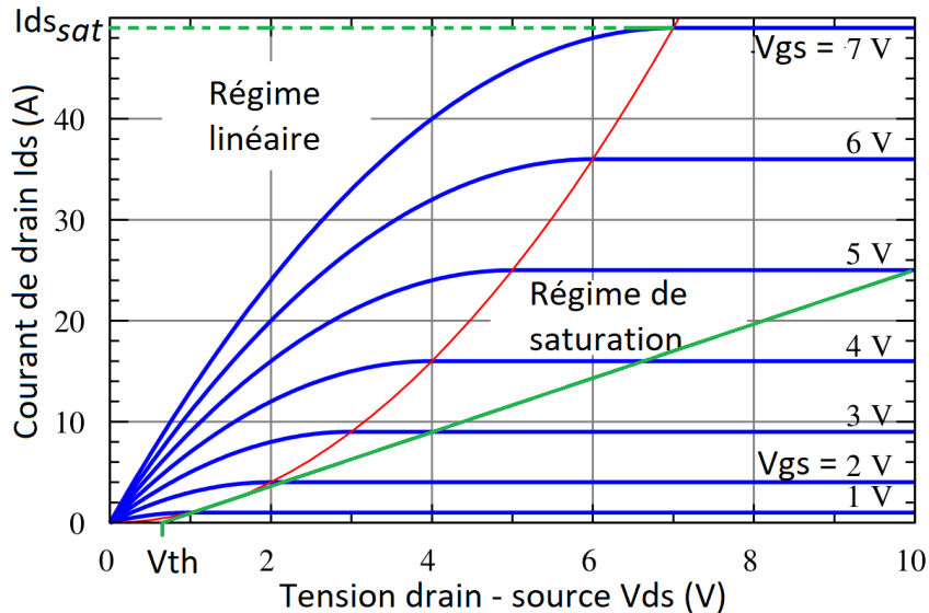
FIGURE 18 – Exemple générique de la caractéristique I-V d'un transistor MOSFET - hors design-kits des travaux de thèse
