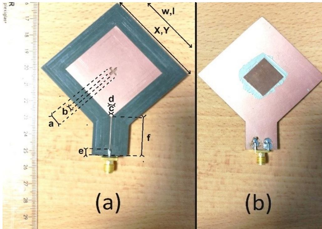
FIGURE 114 – Photographie du prototype d'antenne réalisé. (a) vue dessus. (b) vue dessous. Les dimensions des paramètres sur la figure sont les suivants : w = l = 39,4 mm, X = Y = 60 mm, a = 6 mm, b = 1,6 mm, c = 0,5 mm, d = 4 mm, e = 4,8 mm, f = 22 mm.
