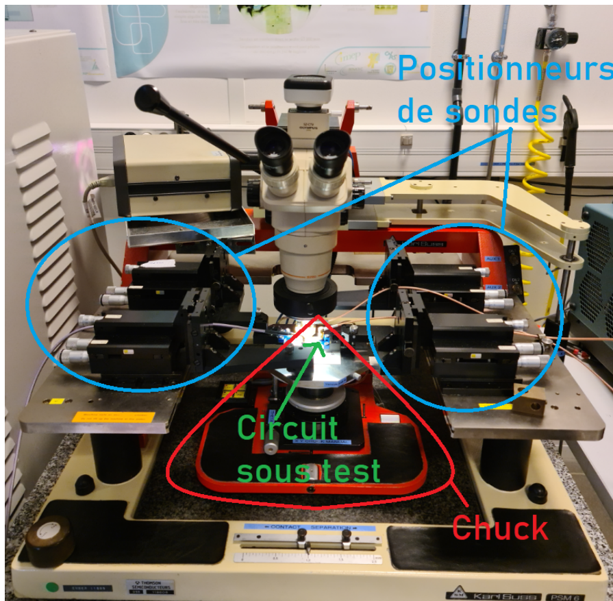
FIGURE 98 – Photographie de la station permettant la pose des sondes et la mesure sous pointes
