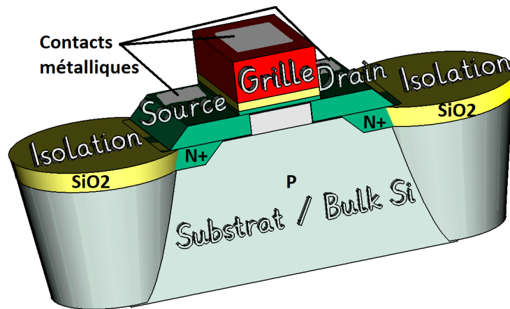
FIGURE 9 – Vue en coupe d'un transistor N en technologie CMOS BULK
