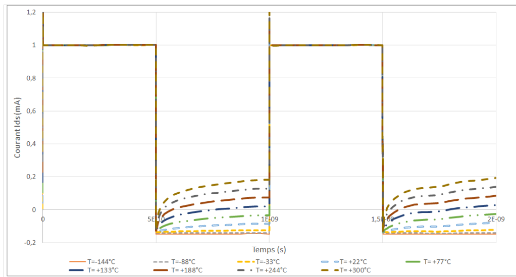
FIGURE 32 – Relevé du courant I_{ds} lors de la commutation du transistor LVT N selon la température
