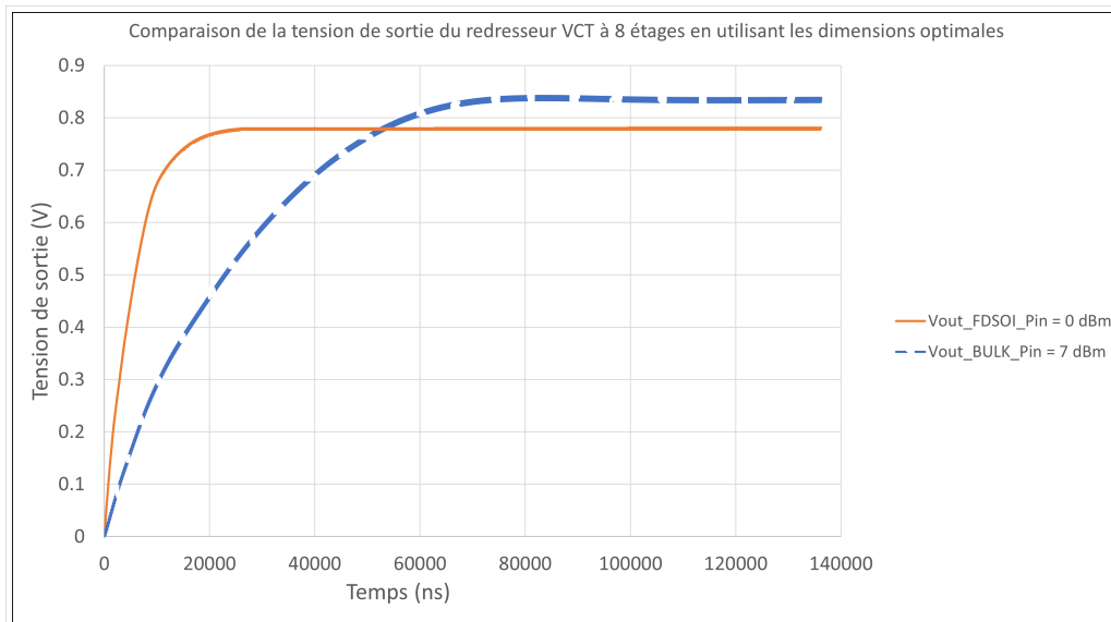
FIGURE 92 – Comparaison de la tension de sortie du redresseur VCT en FDSOI et BULK à dimensions optimales à 0 et +7 dBm
