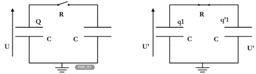
FIGURE 121 – Mise en parallèle d'une capacité chargée et d'une non chargée [112]
