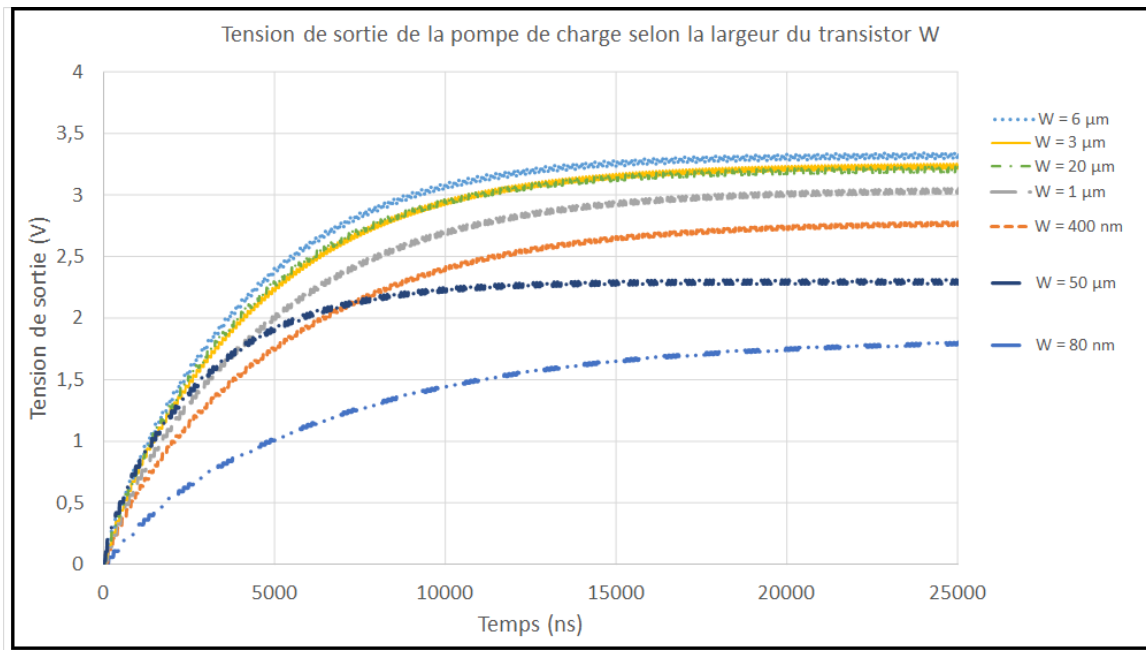
FIGURE 63 – Impact de la largeur du transistor sur la tension de sortie de la pompe de charge
