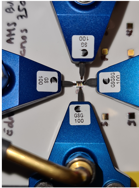
FIGURE 99 – Photographie des sondes entourant la puce pour la mesure
