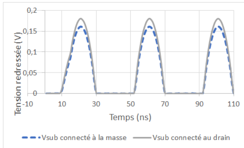
FIGURE 27 – Effet de la polarisation sur le redressement d'un signal alternatif par un transistor LVT en diode
