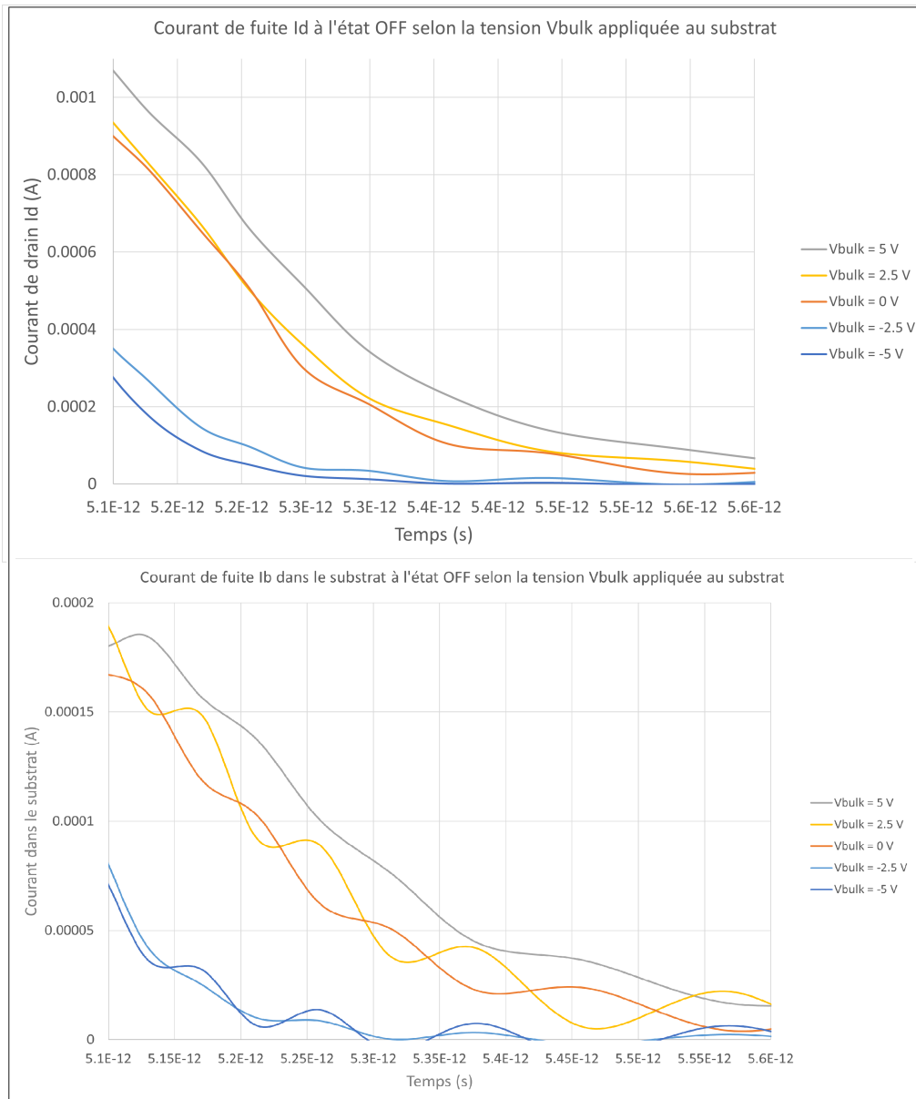
FIGURE 26 – Pertes à l'état "OFF" du transistor dans les courants de drain et bulk
