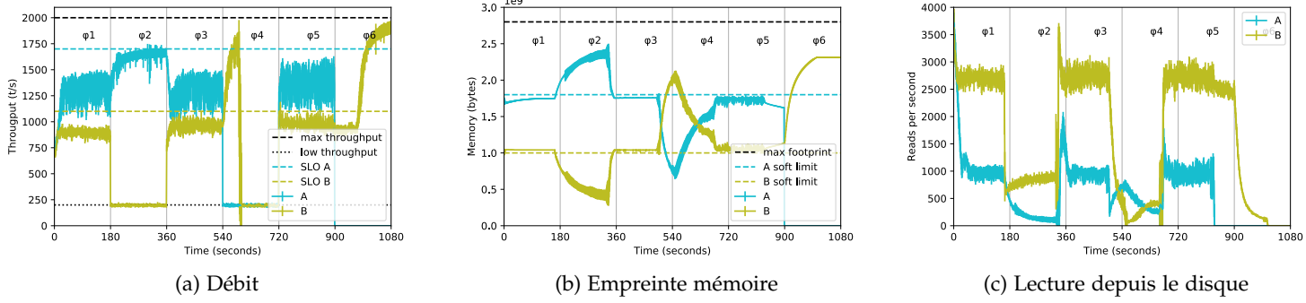
FIGURE 32 – MemOpLight récupérant 2% de l’empreinte mémoire chaque seconde
