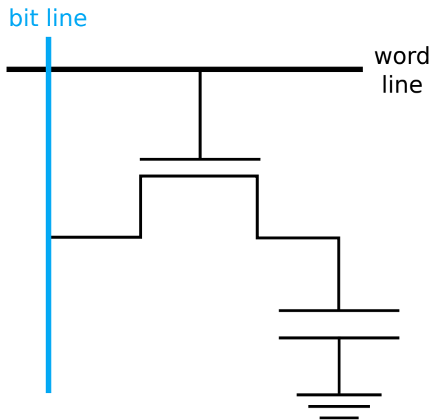
FIGURE 8 – Une cellule de DRAM [80, Figure 8.2]
