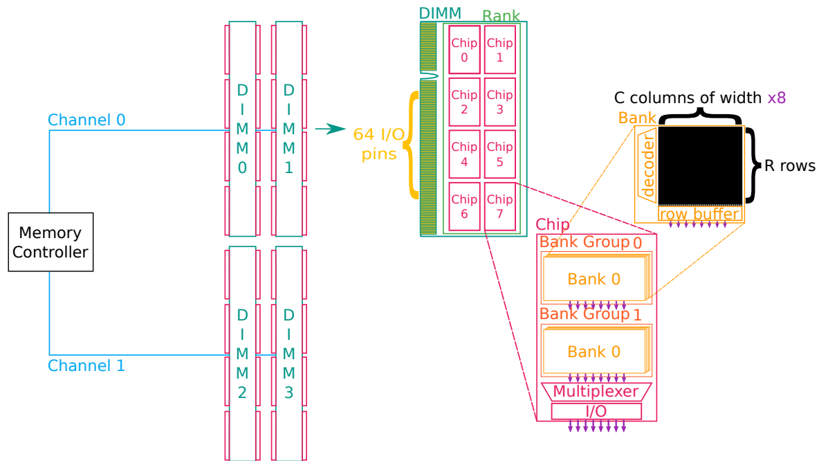
FIGURE 9 – L'organisation de la DDR4 telle que standardisée par le JEDEC [81]
