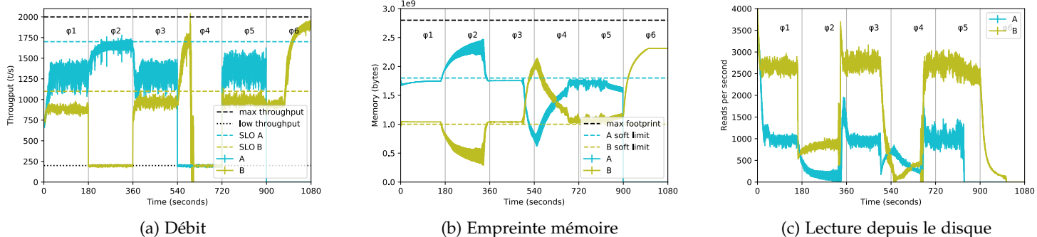
FIGURE 28 – MemOpLight récupérant 1% de l’empreinte mémoire chaque seconde
