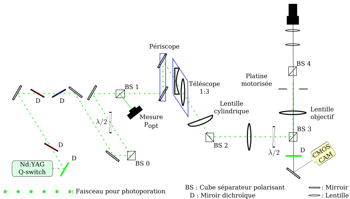
FIGURE 2.6 – Montage optique pour la photoporation.
