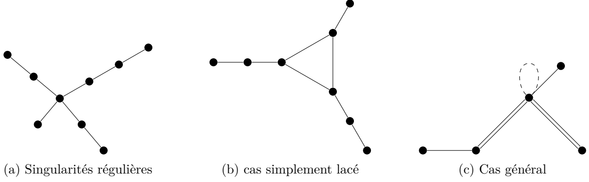
Figure 1.2: Exemples de diagrammes associés à des connexions
