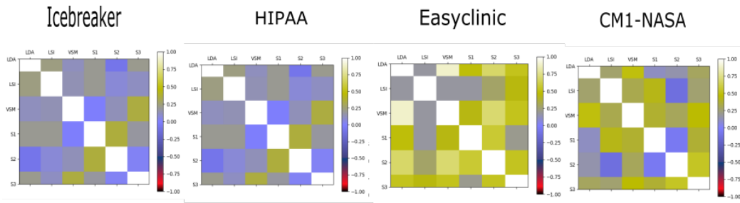
Fig. 6.1 Corrélation entre les mesures et les scores de similarité : cas d'étude académiques. Les mesures de similarité fournies par les techniques VSM , LSI et LDA sont fortement corrélées entre elles. De même les scores de similarité S_1 , S_2 et S_3 sont fortement corrélés entre eux. Toutefois les informations capturées par les mesures de similarité fournies par les techniques VSM , LSI et LDA et les scores de similarité S_1 , S_2 et S_3 sont différentes.
