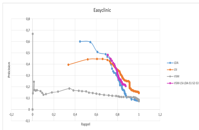
Fig. 6.18 Courbe rappel-précision : cas Easyclinic VSM-LSI-LDA-S1-S2-S3 a les meilleures performances entre les seuils 0.7 et 0.8
