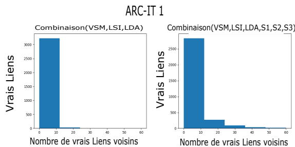
Fig. 6.8 Vérification de la Cluster Hypothesis pour la classe des vrais liens : cas ARC-IT1 L'axe des abscisses représente le nombre de liens parmi les 100 plus proches voisins d'un lien donné qui sont de la même classe que ce dernier ; l'axe des ordonnées représente le nombre de liens ayant parmi leurs 100 plus proches voisins x liens de la même classe, x étant donné par l'axe des abscisses. Par exemple, l'histogramme à gauche indique qu'il y a 3000 vrais liens ayant dans leur plus proches voisins entre 0 et 10 vrais liens.
