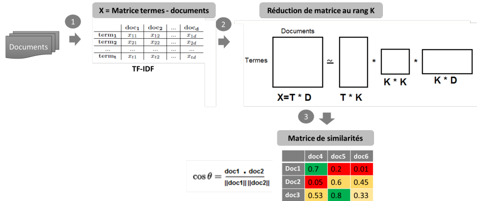
Fig. 4.7 Résumé du fonctionnement de la technique LSI La matrice termes-documents est décomposée en trois sous-matrices. Le produit de ces matrices donne les similarités entre les documents.
