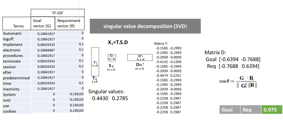
Fig. 4.8 Illustration du calcul de LSI avec l'exigence 1245 et le but 113 Les énoncés des artefacts sont transformés en matrice termes-documents ; Cette matrice est réduite au rang K = 2 ; la mesure de similarité entre les artefacts est supérieure à 0.5
