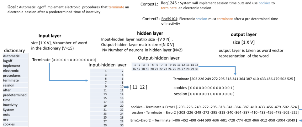
Fig. 4.2 Illustration de la technique Skip-Gram avec le terme « Terminate » du but 113 La couche d’entrée est multipliée par l’ensemble de pondération de la couche cachée d’entrée; le résultat est multiplié avec l’ensemble de pondération de la couche cachée de sortie; un nouveau vecteur de représentation du terme « Terminate » est obtenu; les vecteur de représentation des termes de contexte sont obtenu grâce à leur position dans le vocabulaire V; les vecteurs d’erreur sont calculés par soustraction des vecteurs des termes de contextes avec le nouveau vecteur du terme « Terminate »; la somme des vecteurs d’erreur permet d’obtenir le vecteur d’erreur final, qui correspond à la représentation vectoriel du terme « Terminate ».
