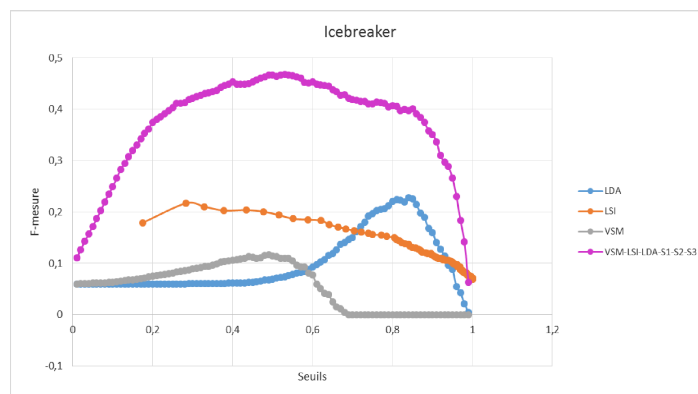
Fig. 6.22 Courbe F-mesure : cas Icebreaker VSM-LSI-LDA-S1-S2-S3 a les meilleures performances sur l'ensemble des seuils.
