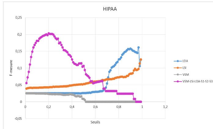
Fig. 6.23 Courbe F -mesure : cas HIPAA VSM-LSI-LDA-S1-S2-S3 a les meilleures performances entre les seuils 0.1 et 0.7 et LSI et LDA ont les meilleures performances aux seuils 0.7 à 1
