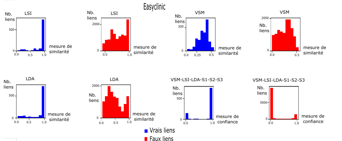
Fig. 6.12 Répartition des mesures de confiance et de similarité des vrais et des faux liens : cas Easyclinic
