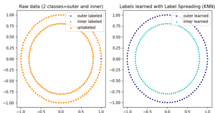
Fig. 4.11 Illustration de l'algorithme LabelSpreading la structure des observations non annotées est cohérente avec la structure des deux classes outer label et inner label , de sorte que l'étiquette de chaque classe peut être propagée par apprentissage à l'ensemble des cercles.
