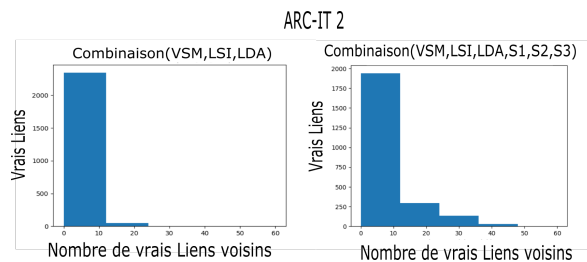
Fig. 6.9 Vérification de la Cluster Hypothesis pour la classe des vrais liens : cas ARC-IT2 L'axe des abscisses représente le nombre de liens parmi les 100 plus proches voisins d'un lien donné qui sont de la même classe que ce dernier ; l'axe des ordonnées représente le nombre de liens ayant parmi leurs 100 plus proches voisins x liens de la même classe, x étant donné par l'axe des abscisses. Par exemple, l'histogramme à gauche indique qu'il y a 2000 vrais liens ayant dans leur plus proches voisins entre 0 et 10 vrais liens.
