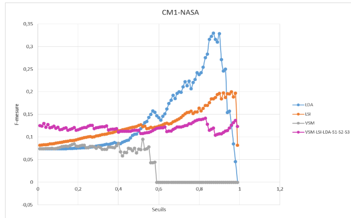
Fig. 6.25 Courbe F -mesure : cas CM1-NASA VSM-LSI-LDA-S1-S2-S3 a les meilleures performances aux seuils 0 à 0.3. LDA et LSI ont les meilleures performances aux seuils 0.4 à 1
