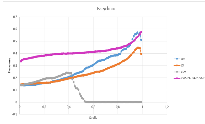
Fig. 6.24 Courbe F -mesure : cas Easyclinic VSM-LSI-LDA-S1-S2-S3 a les meilleures performances sur l'ensemble des seuils.
