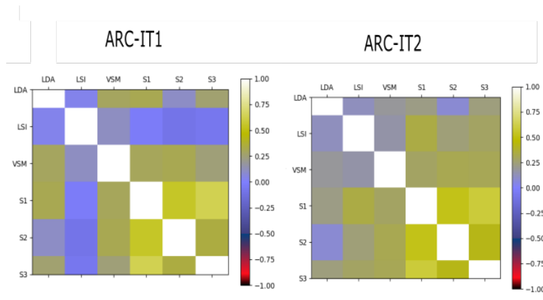
Fig. 6.2 Corrélation entre les mesures et les scores de similarités : cas d'étude industriels. Les mesures de similarité fournies par les techniques VSM , LSI et LDA sont fortement corrélées entre elles. De même les scores de similarité S_1 , S_2 , S_3 sont fortement corrélés entre eux. Toutefois les informations capturées par les mesures de similarité fournies par les techniques VSM , LSI et LDA et les scores de similarité S_1 , S_2 et S_3 sont différentes.
