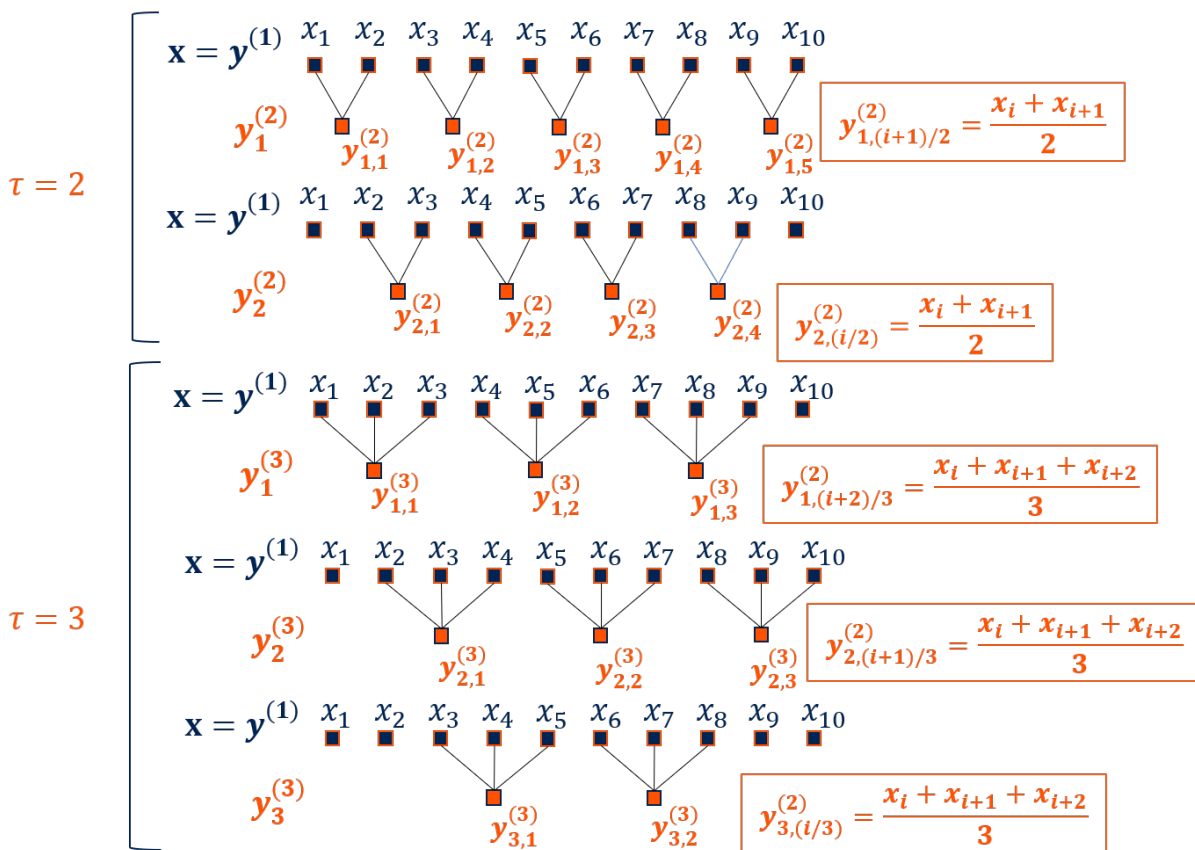
FIGURE 2.3 – Exemple de la procédure multi-échelle de composite coarse-grained pour un signal d'origine \mathbf{x} de 10 échantillons aux échelles temporelles \tau = 2 et \tau = 3 .
