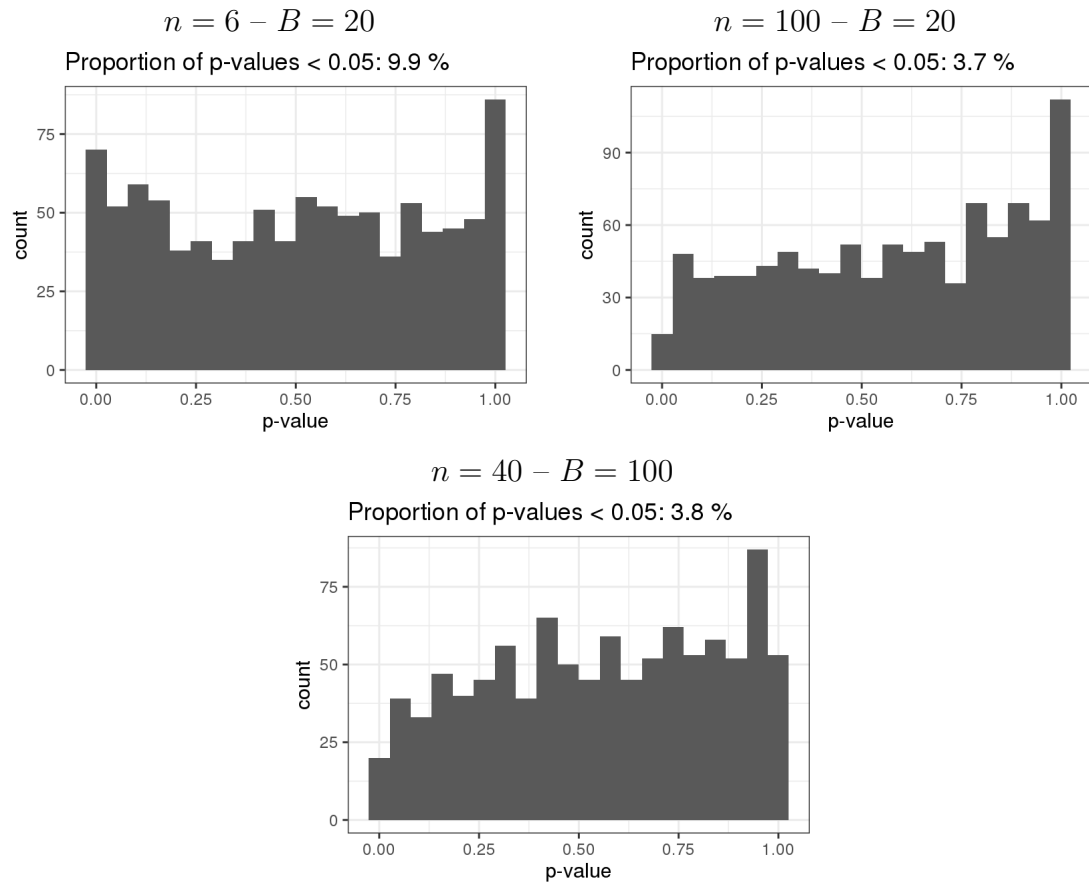
FIGURE 3.7: Distribution des p -valeurs p_{\text{Simés}} (définies dans l'équation 3.12) pour l'analyse différentielle d'arbres à partir de la simulation sur données GWAS, pour différentes valeurs de n (nombre total d'arbres dans les deux conditions) et B (nombre de feuilles dans les arbres).
