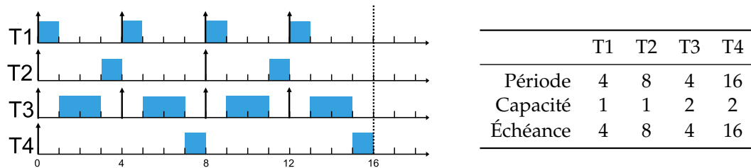
FIGURE 3.1 – Exemple d'ordonnancement obtenu avec la politique Earliest Deadline First .
