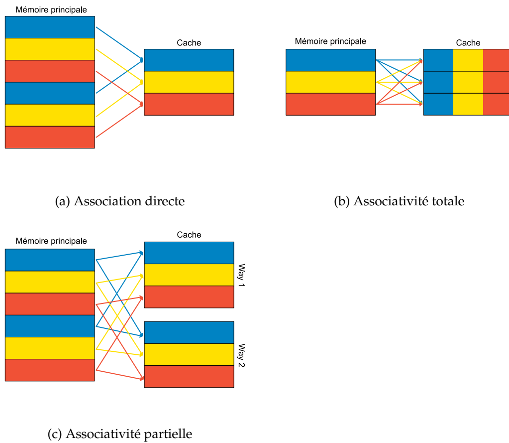
FIGURE 2.9 – Politiques de correspondances
