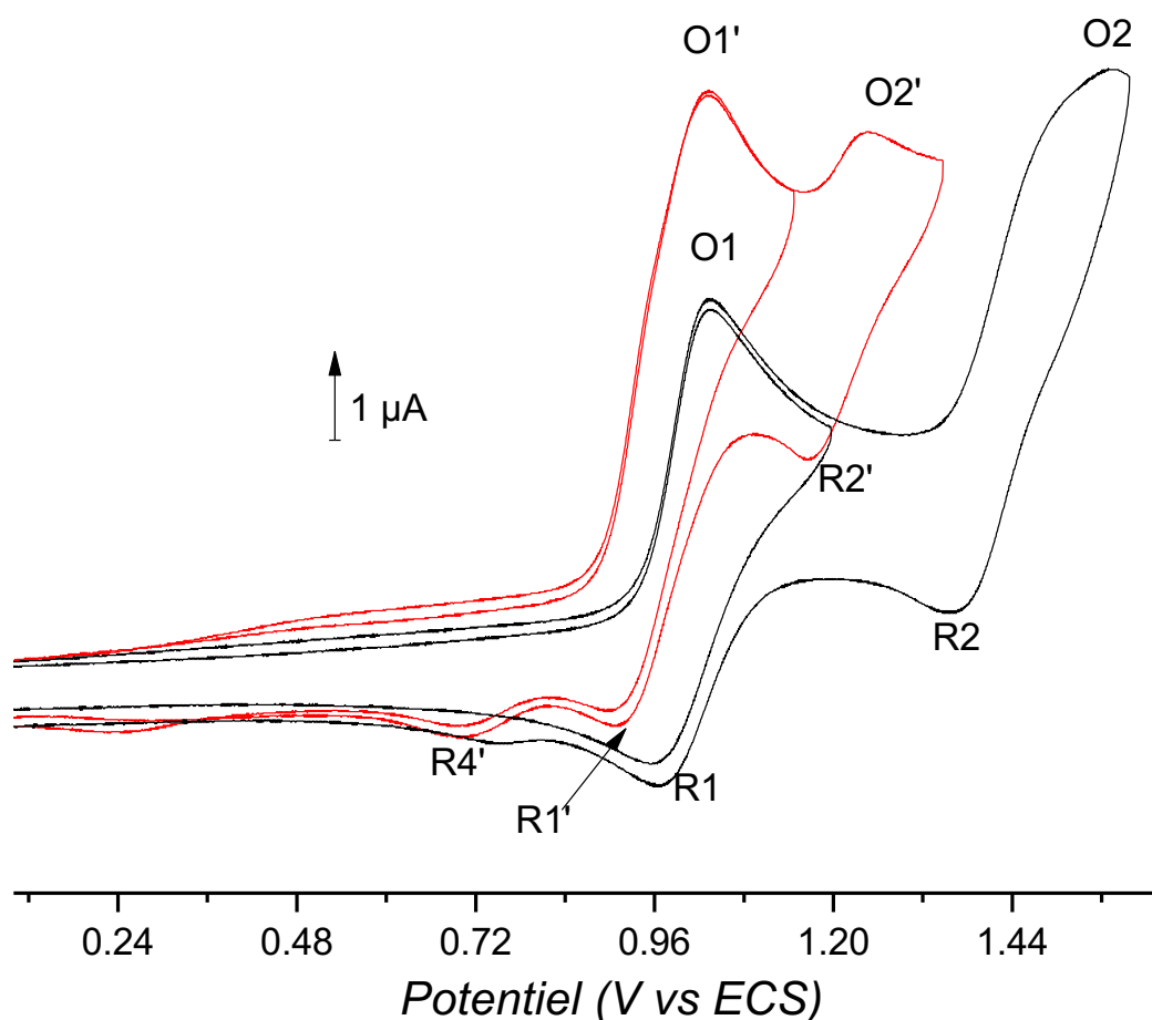
Figure 86. Voltammogrammes cycliques de Ni-PhDTP dans le \text{CH}_2\text{Cl}_2 (en noir) et dans un mélange \text{CH}_2\text{Cl}_2/\text{CH}_3\text{CN} (4:1 v/v) (en rouge) ( c = 5 \cdot 10^{-4} \text{ M} , 0,1 \text{ M TEAPF}_6 , électrode de travail : Pt \varnothing = 2 \text{ mm} , v = 100 \text{ mV}\cdot\text{s}^{-1} ). [89]
