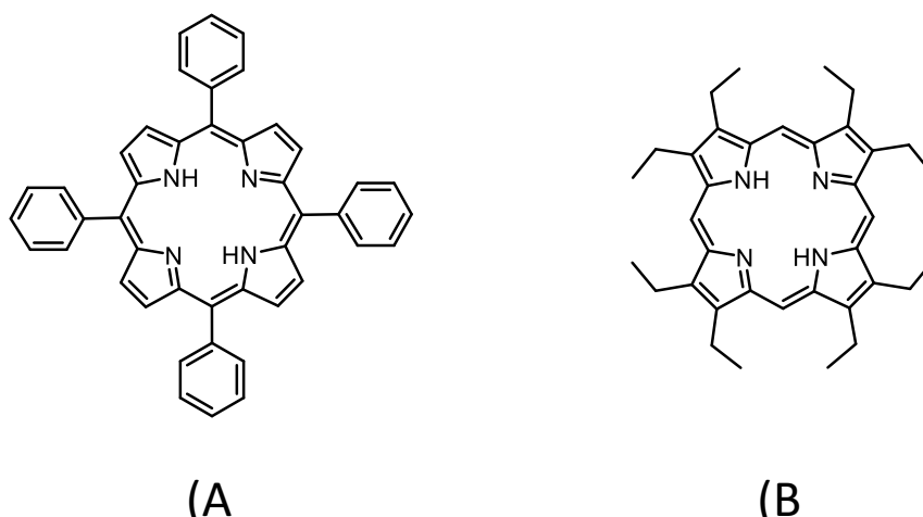
Figure 6. Structures de la tétraphénylporphyrine (A) et de l'octaéthylporphyrine (B) sous forme base libre.
