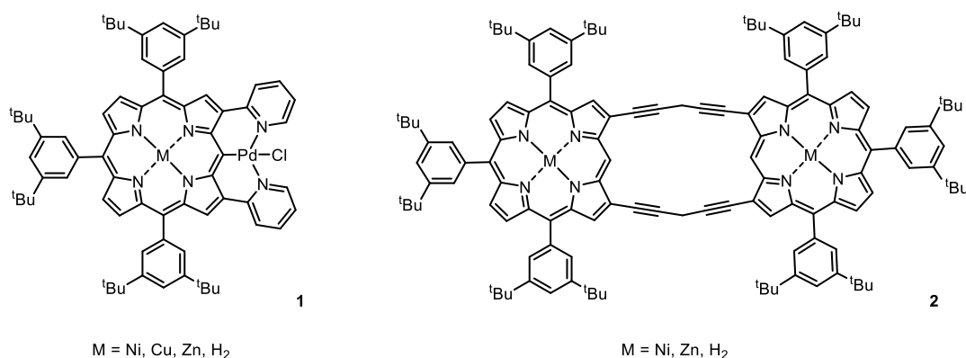
Figure 18. Exemples d'utilisation des porphyrines borylées en positions \beta . [66,68]
