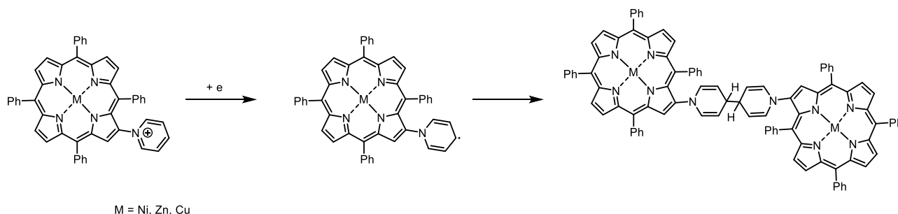
Schéma 87. Formation du dimère de type 1,1',4,4'-tétrahydro-4,4'-bipyridine par réduction d'un pyridinium non substitué en position 4 porté par une métallo-tétraphénylporphyrine. [32]
