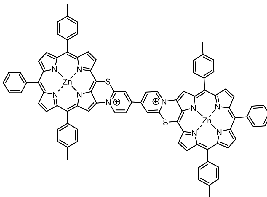
Figure 95. Structure proposée de viologène obtenu par réduction de la 5-(pyridin-2-ylthio)-10,20-bis( p -tolyl)-15-phénylporphyrine de Zn(II) fusionnée 27 + , PF 6 - au potentiel de réduction du pyridinium.
