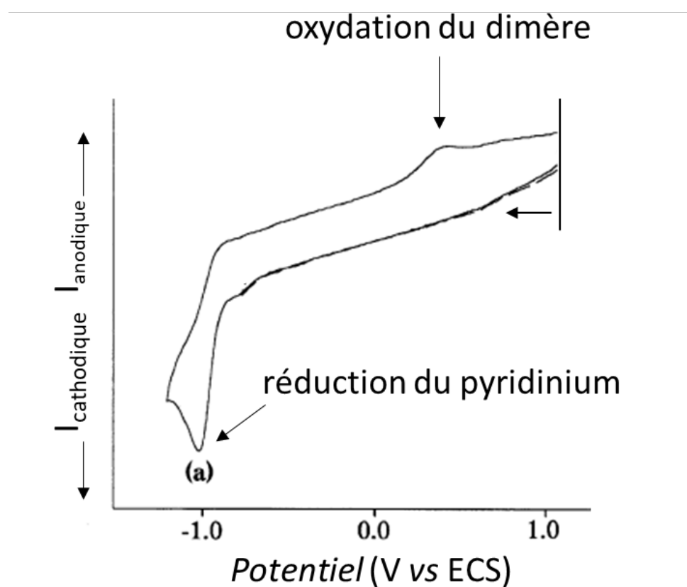
Schéma 87. Formation du dimère de type 1,1',4,4'-tétrahydro-4,4'-bipyridine par réduction d'un pyridinium non substitué en position 4 porté par une métallo-tétraphénylporphyrine. [32]
