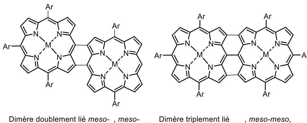
Figure 29. Structures de dimères doublement et triplements liés.
