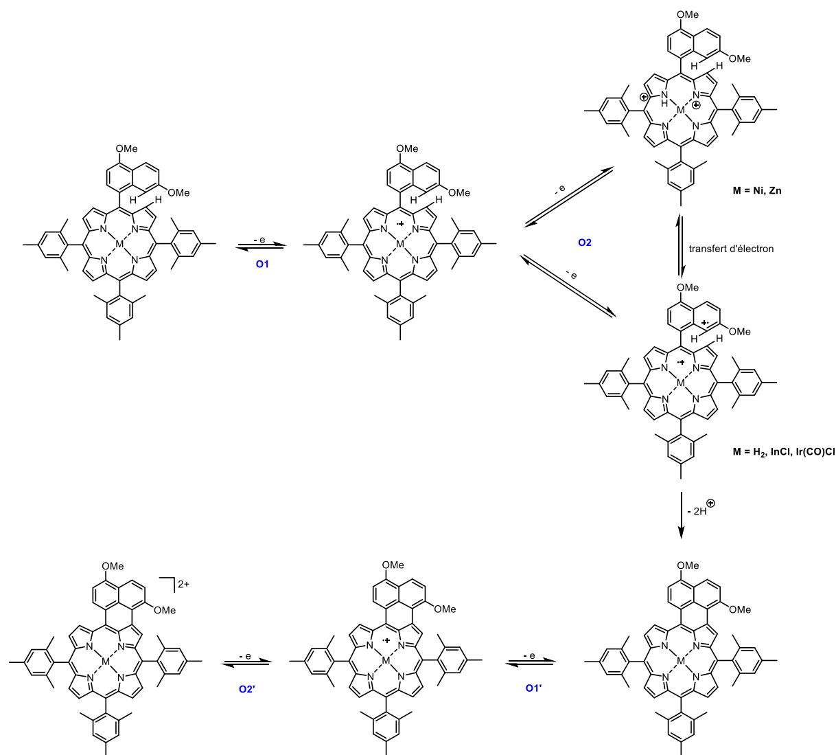
Schéma 55. Proposition de mécanisme pour le couplage oxydant aromatique C-C électrochimique du fragment 4,7-diméthoxynaphtalèn-1-yl sur le cœur porphyrinique, adapté des travaux de Kadish et Gryko. [140,159]
