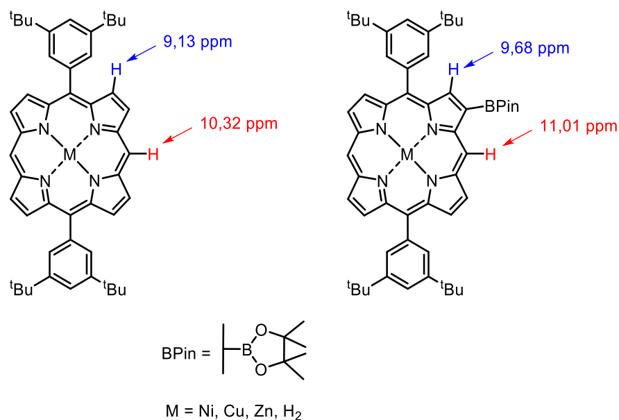
Figure 17. Effet de déblindage en RMN 1 H par l'introduction du fragment borylé. Les déplacements chimiques des protons \beta -pyrroliques et meso mentionnés correspondent à ceux observés pour les deux porphyrines base libre.
