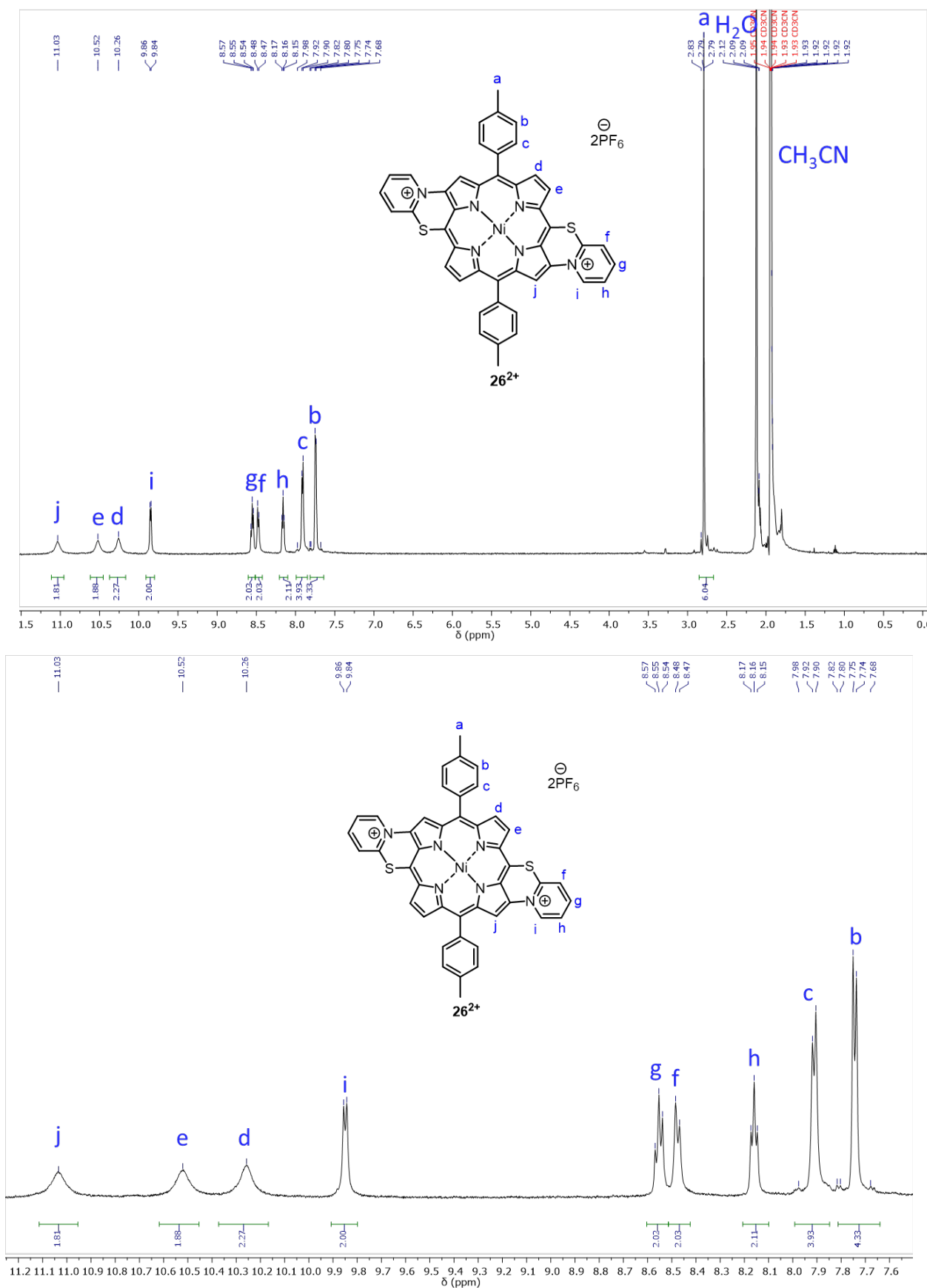
Figure 57. Vue globale (en haut) et centrée sur la partie aromatique (en bas) du spectre RMN ^1\text{H} de la 5,15-bis(pyridin-2-ylthio)-10,20-bis(p-tolyl)porphyrine de Ni(II) doublement fusionnée 26^{2+} , 2\text{PF}_6^- ( \text{CD}_3\text{CN} , 500 MHz, 298 K).
