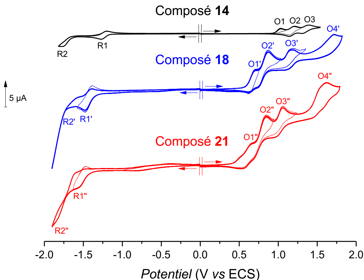
Figure 46. Voltammogrammes obtenus lors des analyses de la 5-(pyridin-2-ylthio)-10,20-bis(p-tolyl)-15-phénylporphyrine métallée au Ni(II) 14 (en noir) au Zn(II) 18 en présence d'un équivalent de pyridine séchée sur tamis moléculaire (en bleu) et au Mg(II) 21 également en présence d'un équivalent de pyridine séchée sur tamis moléculaire (en rouge) ( c = 10^{-3} M, \text{CH}_2\text{Cl}_2 0,1 M \text{TBAPF}_6 , électrode de travail : Pt \varnothing = 1 mm pour 14 et 2 mm pour 18 et 21 , v = 100 \text{mV}\cdot\text{s}^{-1} ).
