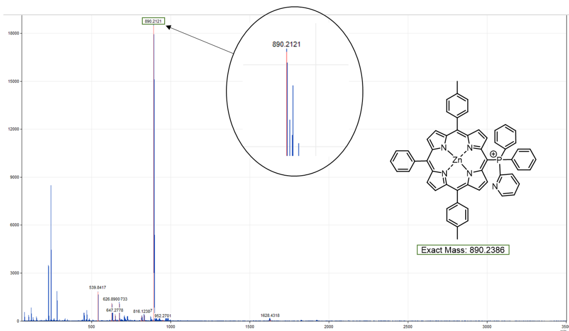
Figure 97. Spectre de masse MALDI-TOF enregistré sur la fraction 2 de la deuxième colonne réalisée pour purifier la 5-(diphényl-2-pyridylphosphine)-10,20-bis(p-tolyl)-15-phénylporphyrine de Zn(II) 31 .
