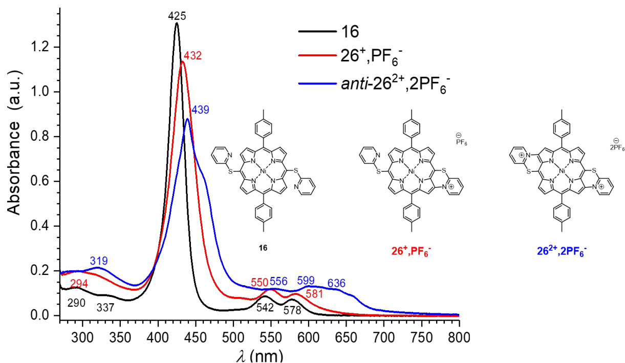
Figure 60. Superposition des spectres d'absorption UV-visibles pour les dérivés de la 5,15-bis(pyridin-2-ylthio)-10,20-bis( p -tolyl)porphyrine de Ni(II) non fusionnée 16 , monofusionnée 26 + ,PF 6 - et doublement fusionnée 26 2+ ,2PF 6 - (C = 7,5 μM, l = 1 cm, DMF).
