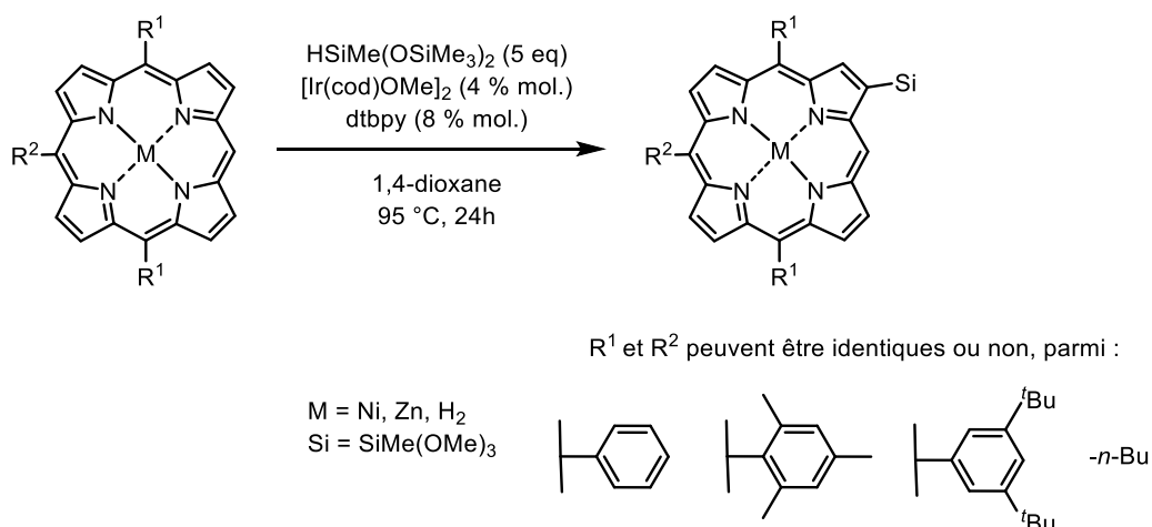
Schéma 18. Silylation en position \beta de porphyrines. [71]
