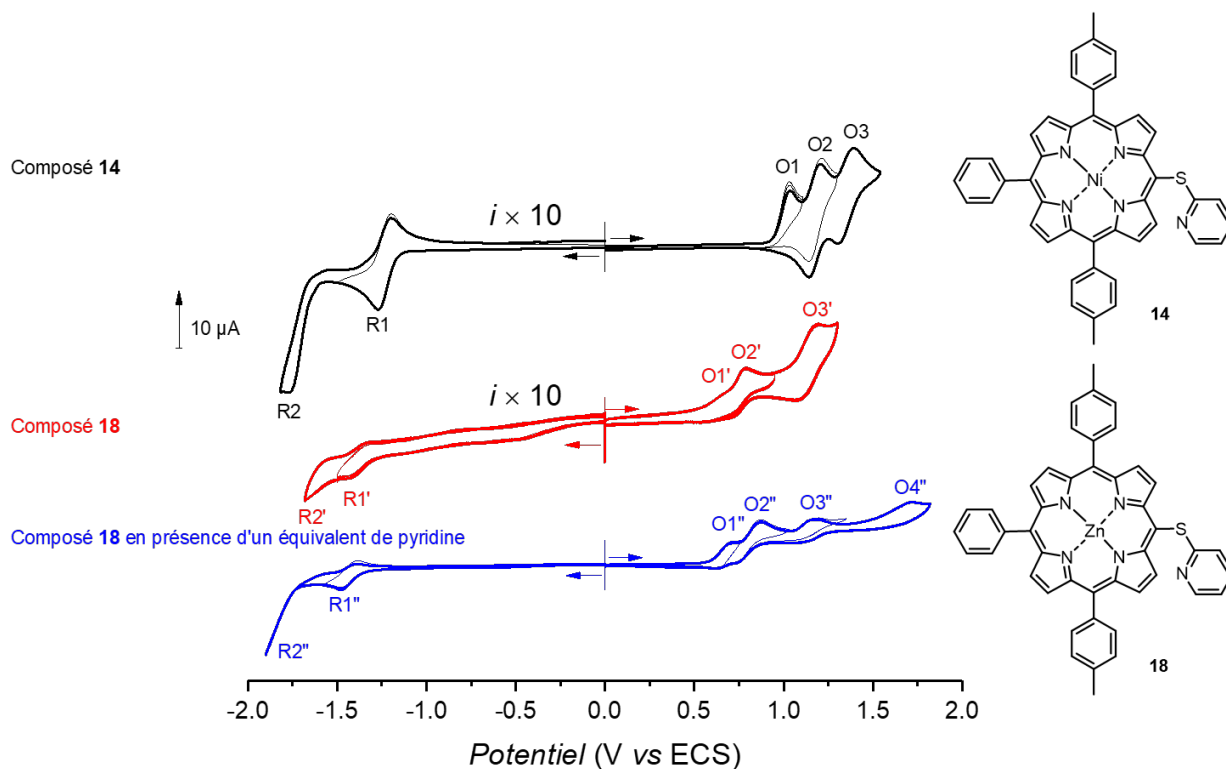
Figure 63. Voltammogrammes cycliques de 14 (en noir), 18 (en rouge) et 18 avec un équivalent de pyridine séchée sur tamis moléculaire (en bleu) ( c = 10^{-3} \text{ M} , \text{CH}_2\text{Cl}_2 0,1 M TBAPF 6 , électrode de travail : Pt \varnothing = 1 \text{ mm} (pour 14 ) et 2 mm (pour 18 ), v = 100 \text{ mV}\cdot\text{s}^{-1} ). Afin d'améliorer la visibilité des pics redox de chaque produit, les intensités des voltammogrammes de 14 (en noir) et 18 sans pyridine dans le milieu (en rouge) ont été multipliées par un facteur 10.
