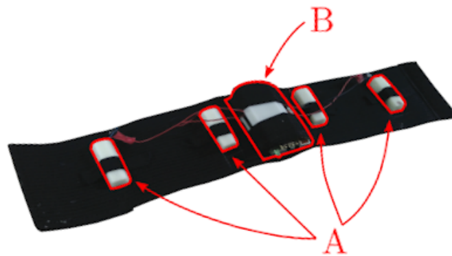
Figure 8.3 – Brassards vibrotactiles, composés de quatre moteur vibrants (A). L'électronique est protégée par un boîte imprimée en 3D (B). [Scheggi et al., 2016].
