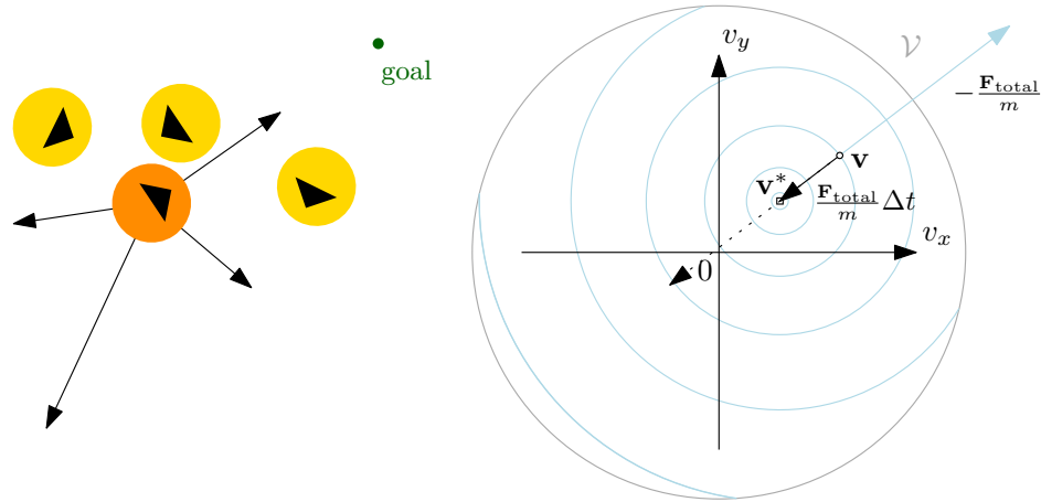
Figure 5.1 – Application du principe unificateur aux méthodes de navigation utilisant des forces. Gauche : un agent est soumis à des forces exercées par d'autres agents, et par son objectif ( goal ). Droite : Le coût \mathcal{C}(\mathbf{v}') dépend de la distance entre \mathbf{v}' et la vitesse \mathbf{v}^* obtenue par application de la deuxième loi de Newton.
