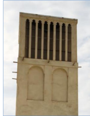
Figure 93 : Cage et colonne d'un Badgir
