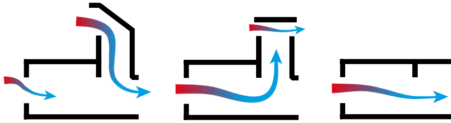
Figure 19 : Passage du vent dans un bâtiment
