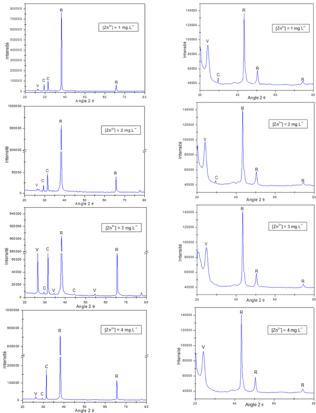
Figure 8 : Diagramme DRX des précipités solides déposés sur la surface pré-entartée en présence du chlorure de zinc
