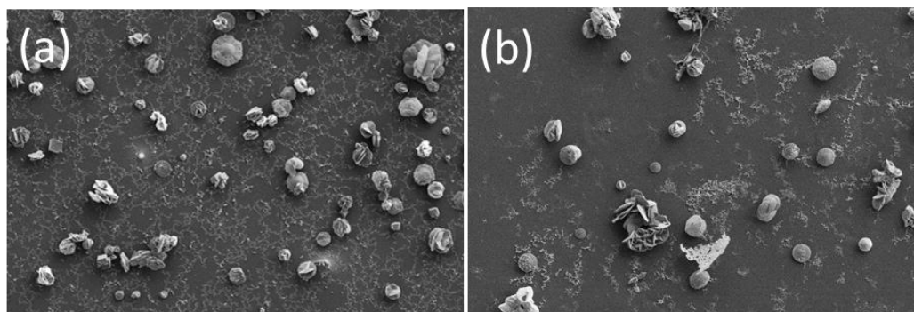
Figure IV-19 : Images MEB des cristaux déposés sur le film sol-gel dopés par des ions cuivre (a) 10^{-5} mol et (b) 10^{-4} mol.
