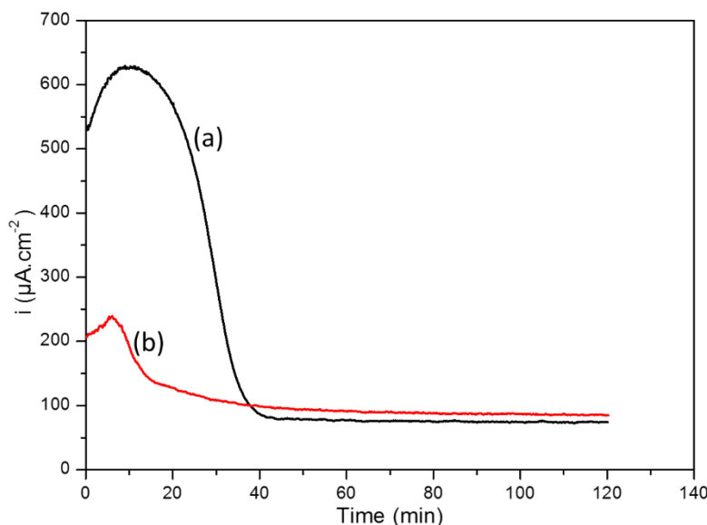
Figure IV-4 : Evolution du courant en fonction du temps sur une électrode en acier au carbone sans et avec revêtement sol-gel. (a) Acier au carbone nu, (b) Acier au carbone avec revêtement sol-gel. Solution de CaCO 3 à 50°F, 30 °C.
