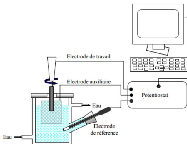
Figure II-9 : Dispositif expérimental de la mesure de chronoampérométrie.
