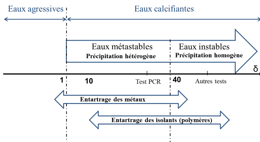
Figure I-3 : Nature des eaux en fonction de \delta et domaine thermodynamiques des entartrages.
