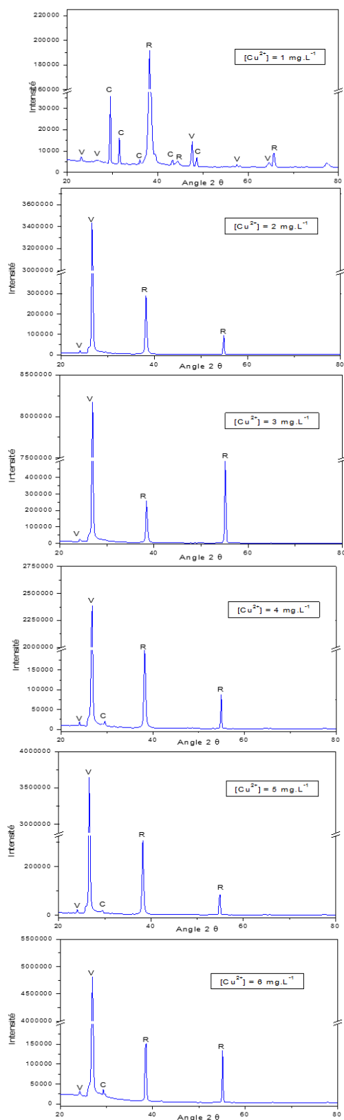
Figure 7 : Diagramme DRX des précipités solides déposés sur la surface pré-entartée en présence du sulfate de cuivre
