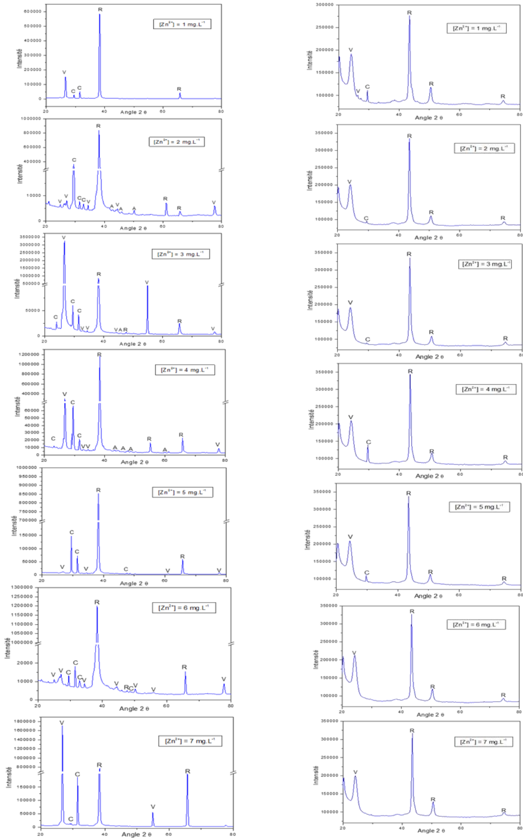
Figure 9 : Diagramme DRX des précipités solides déposés sur la surface pré-entartée en présence du nitrate de zinc
