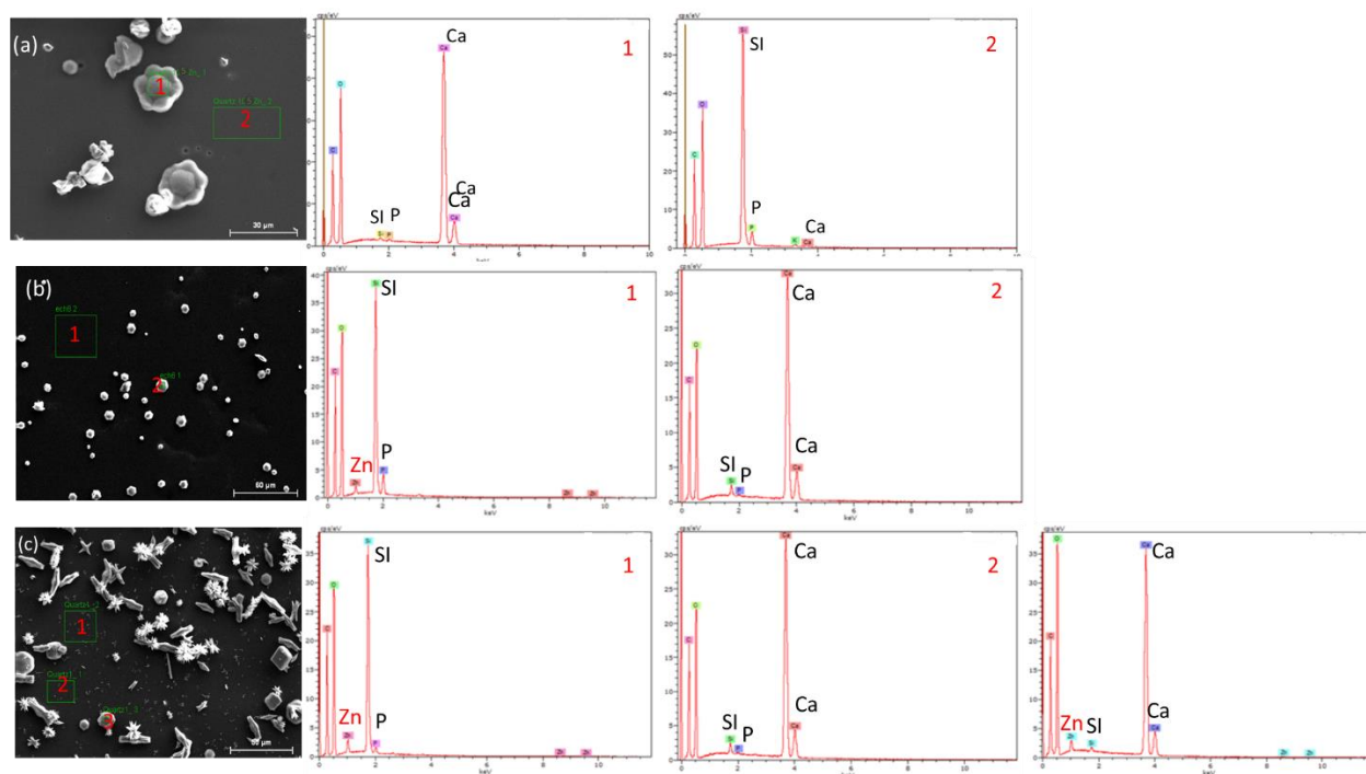
Figure 14 : Analyse EDX de la surface de l'acier inoxydable recouverte par un film sol-gel dopés par des ions Zn^{2+} avec (a) 10^{-5} mol, (b) 10^{-3} mol et (c) 10^{-2} mol.
