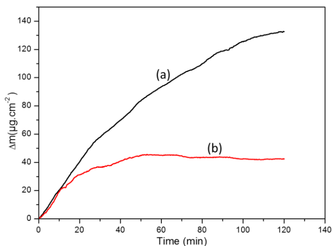
Figure IV-14 : Evolution de la masse du carbonate de calcium mesurée sur acier 316L sans et avec revêtement sol-gel. (a) Acier 316L nu, (b) Acier 316L avec revêtement sol-gel.
