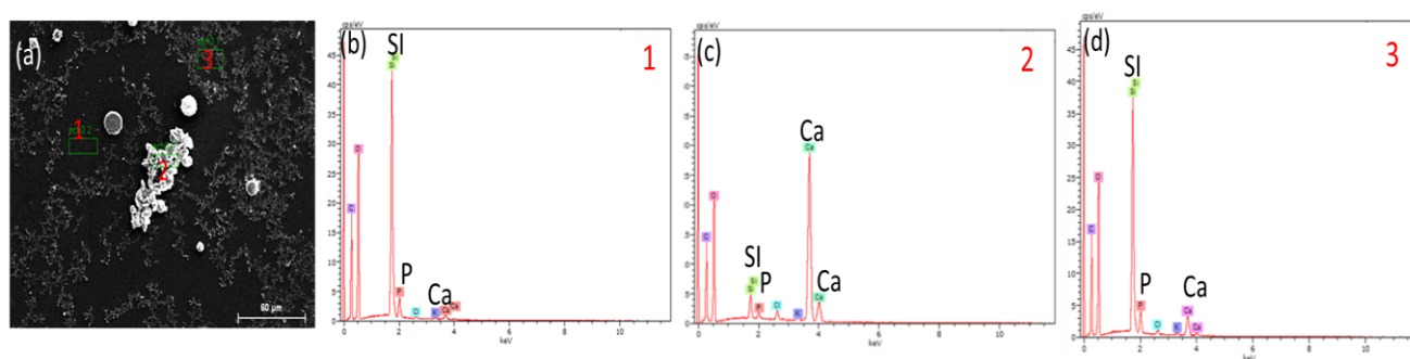
Figure IV-18 : (a) Photo MEB de la surface d'acier inoxydable recouverte par un film sol-gel après un test de QCM. Analyse EDX du film déposé sur acier inoxydable après application de la technique de QCM pour (b) la zone 1, (c) la zone 2 et (d) la zone 3.
