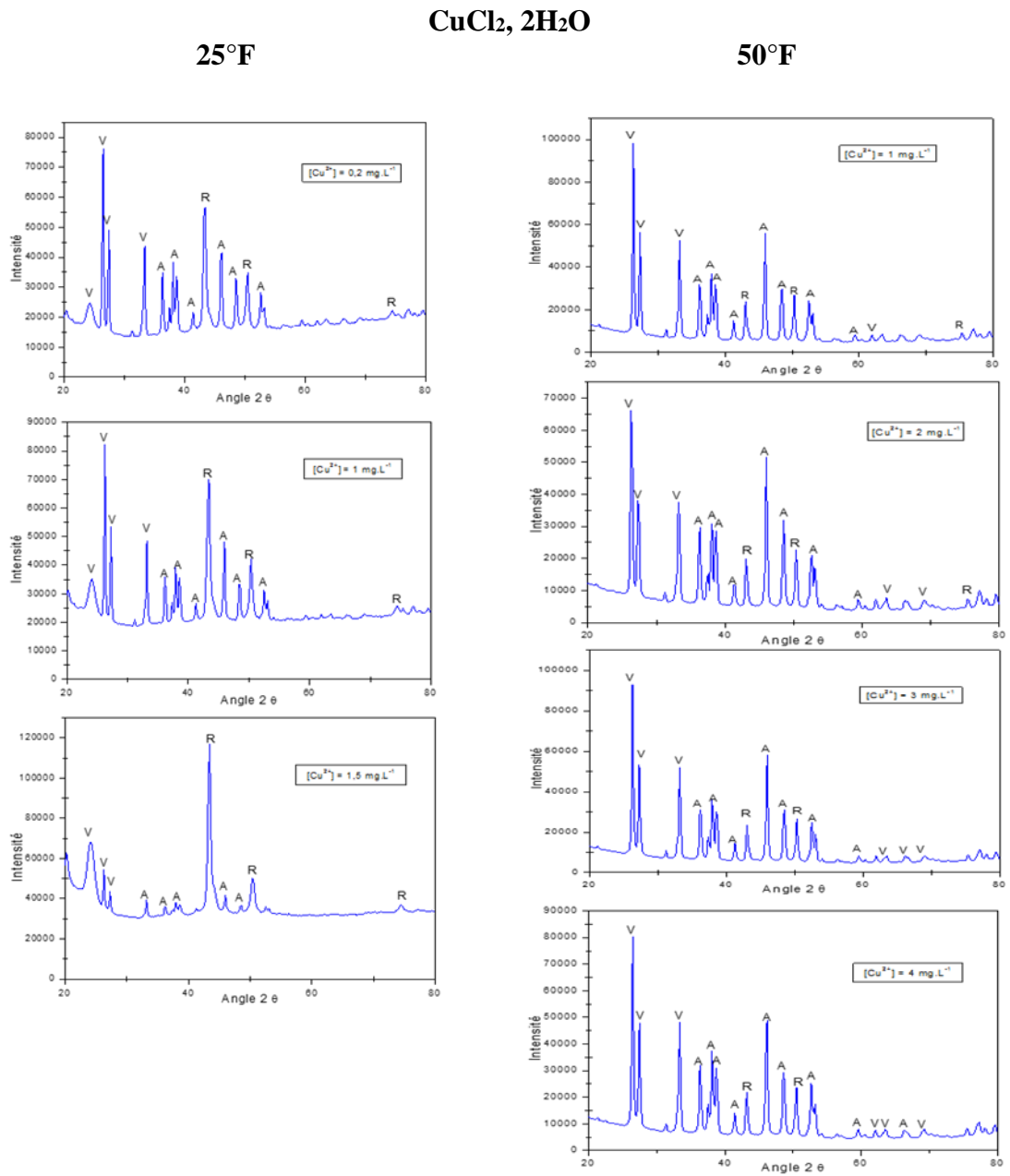
Figure 1 : Diagramme DRX des solutions calcocarboniques pures en présence de différentes concentrations de CuCl 2 , 2H 2 O
