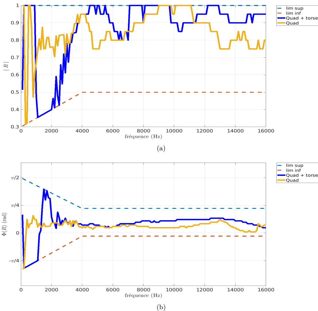
FIGURE 4.34: Modules (a) et phases (b) des coefficients de réflexion obtenus grâce aux deux recherches quadrillées. En jaune, le résultat sans torse absorbant. En bleu, le résultat avec torse absorbant.
