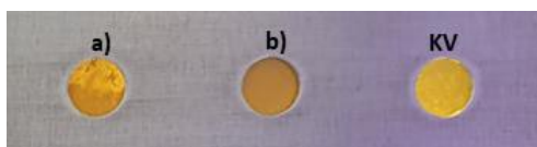
Figure 41 : Photographie des deux échantillons de \text{TiO}_2\text{-NM102} avec, a) la pastille inhomogène, b) la pastille homogène et compacte et KV le scotch en kapton vide « ligne de base »
