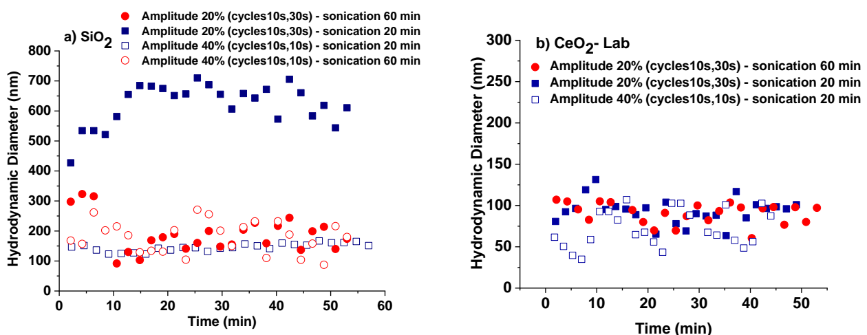
Figure 33 : Évolution du diamètre hydrodynamique moyen ( D_h ) en fonction du temps en faisant varier le temps d'ultrasonication total entre 20 min et 60 min avec des cycles de 10 s ON et 10s OFF à 40% d'amplitude ou 10s ON et 30 s OFF à 20% d'amplitude, pour (a) SiO 2 -Tixosil43 (pH=7) et (b) CeO 2 -Lab (pH=2).
