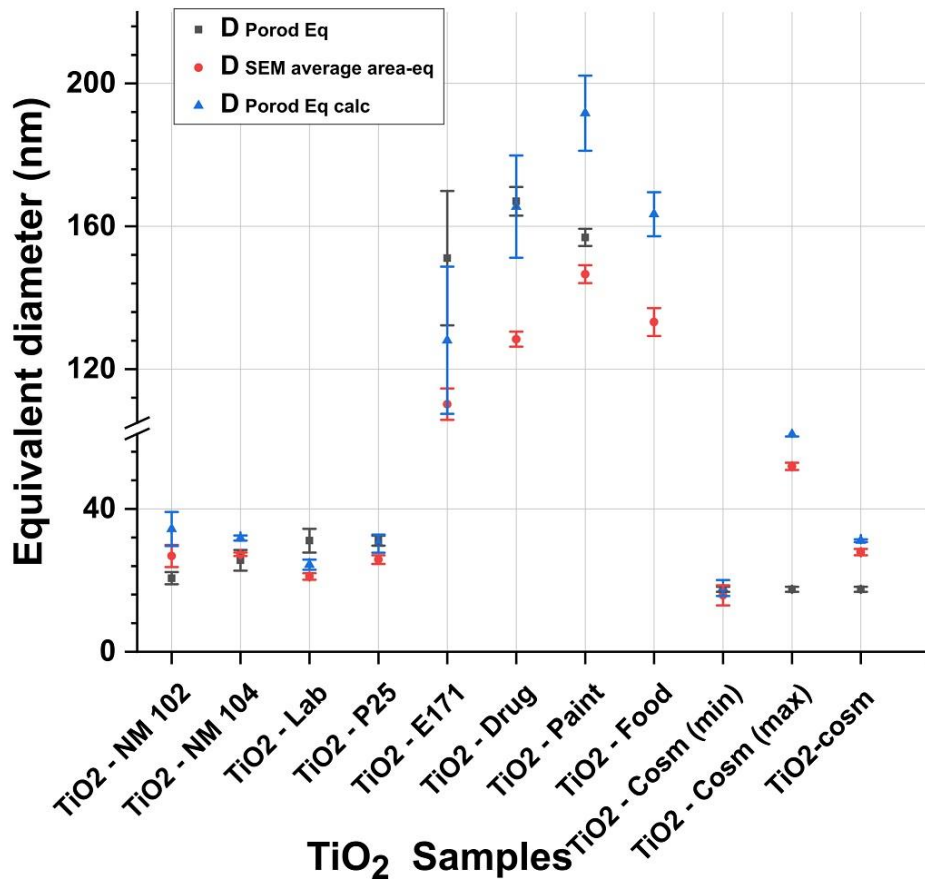
Figure 48 : Les diamètres équivalents mesurés par SAXS et MEB ainsi que les diamètres équivalents de Pord calculé à partir de la distribution en taille du MEB (avec les répétabilité en barres d'erreurs)
