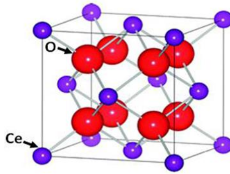
Figure 5 : Représentation de la maille cristalline élémentaire du CeO 2 , de type fluorine (Figure tirée de [41])
