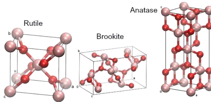
Figure 3 : Représentation des trois mailles cristallines élémentaires du TiO 2 : Rutile, Brookite et Anatase (Figure tirée de [32]).
