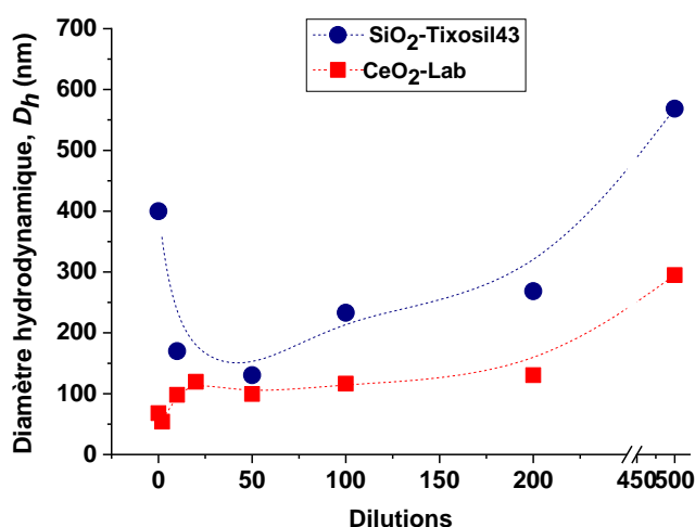
Figure 30 : Evolution du D_h en fonction des différents facteurs de dilutions
