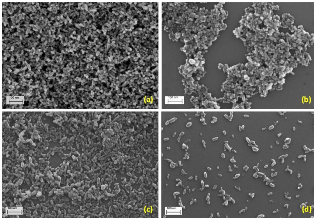
Figure 28 : Images MEB des particules de TiO 2 -Lab déposées à a) pH=6 sans spin-coating, b) pH=6 avec spin-coating, c) pH=2 sans spin-coating et d) pH=2 avec spin coating.
