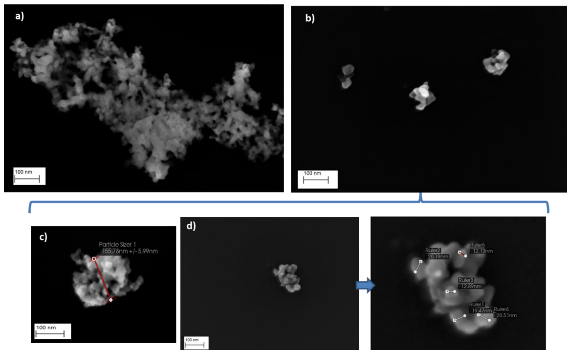
Figure 34 : Impact des paramètres d'ultrasonication pour le SiO 2 -Tixosil43, a) image MEB avec les paramètres habituels d'ultrasonication (20%, 10s ON et 30s OFF, 20 min), b) image MEB obtenue après optimisation des paramètres d'ultrasonication (40%, 10s ON et 10s OFF, 20 min), c) image MEB de la mesure de la taille d'un agglomérat/agrégat avec les paramètres optimisés et d) un exemple de mesure de taille de nanoparticules constitutive d'agglomérats à l'aide du logiciel Platypus.
