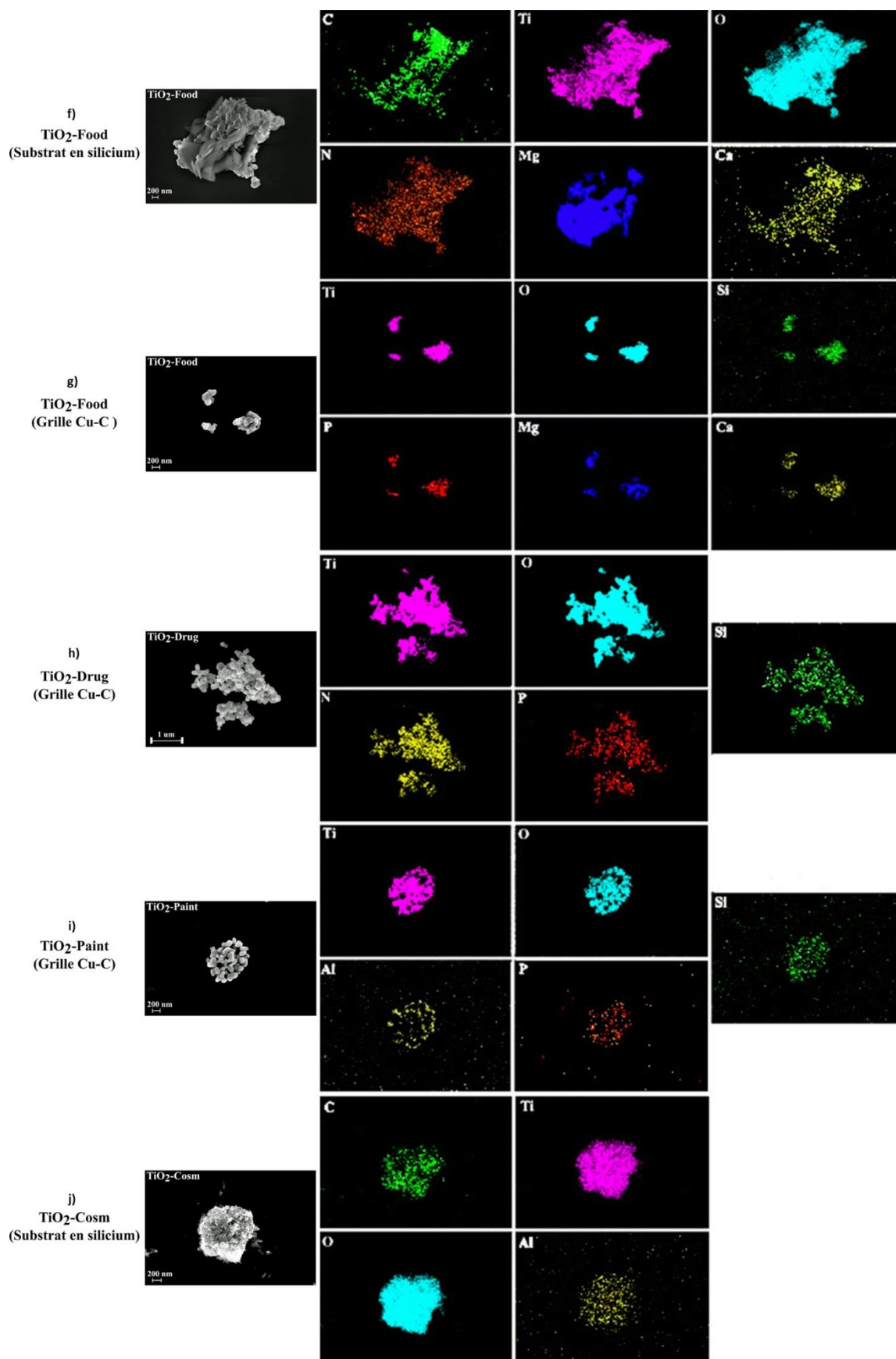
Figure 38 : Les cartographies EDS des échantillons de \text{TiO}_2 extraits de produits manufacturés, réalisées sur un substrat en silicium ou une grille Cu-C
