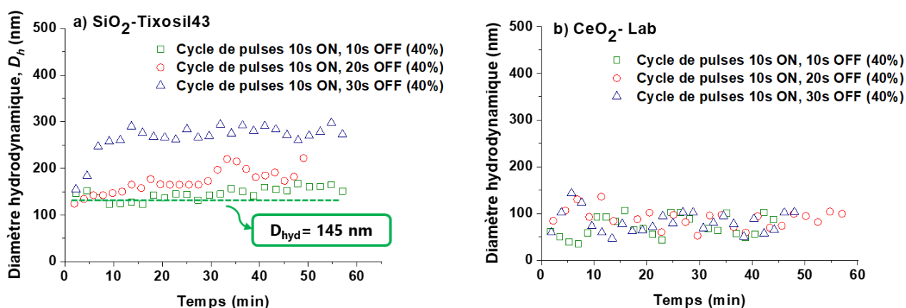
Figure 32 : Évolution du diamètre hydrodynamique moyen ( D_h ) en fonction du temps après 20 minutes d'ultrasonication avec des cycles de 10 s ON et 10, 20 ou 30 s OFF, pour (a) SiO 2 (pH= 8) et (b) CeO 2 -Lab (pH= 2) avec une amplitude fixée à 40% dans les deux cas.
