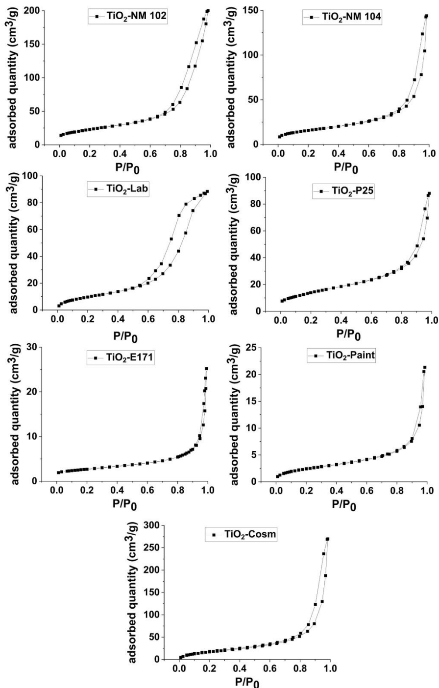
Figure 45 : Isothermes BET correspondants aux échantillons de TiO 2 analysés
