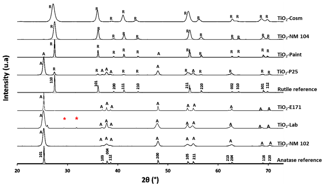
Figure 39 : Diffractogrammes DRX des échantillons de TiO 2 (avec les spectres de références (A) anatase et (R) rutile). Les (*) identifie des impuretés autre que le TiO 2 .
