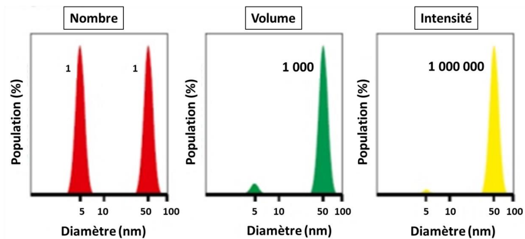
Figure 24 : Distribution en taille en nombre, volume et intensité d'un système bimodal (5nm et 50nm) (Figure tirée de [64])
