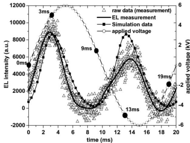
Figure 8: Comparaison entre l'électroluminescence mesurée et la recombinaison des charges simulée sous tension alternative.
