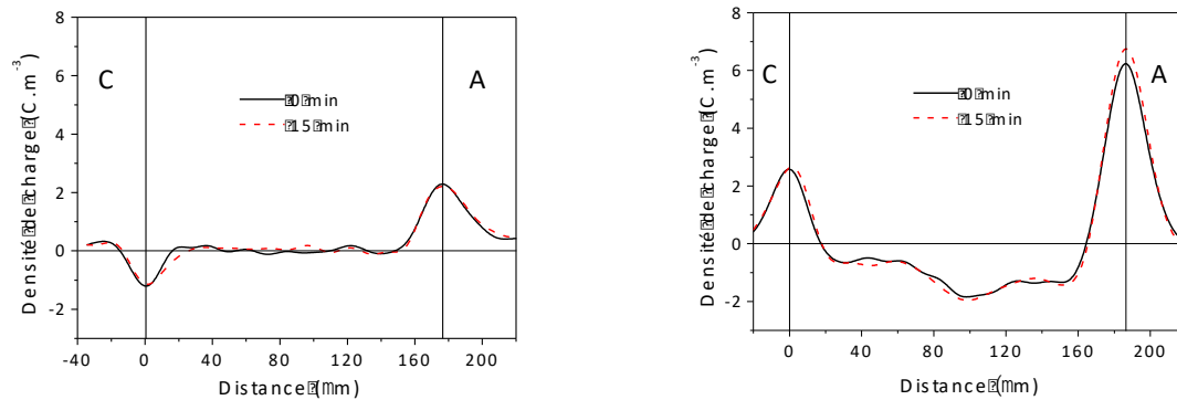
Figure 20: Profils de charge d'espace obtenus par la méthode PEA en condition de court-circuit à 25^\circ\text{C} avant la rampe de température (PEA-1 sur la Figure 18), pour un PEN pré-polarisé a) à 130^\circ\text{C} et b) à 170^\circ\text{C} .
