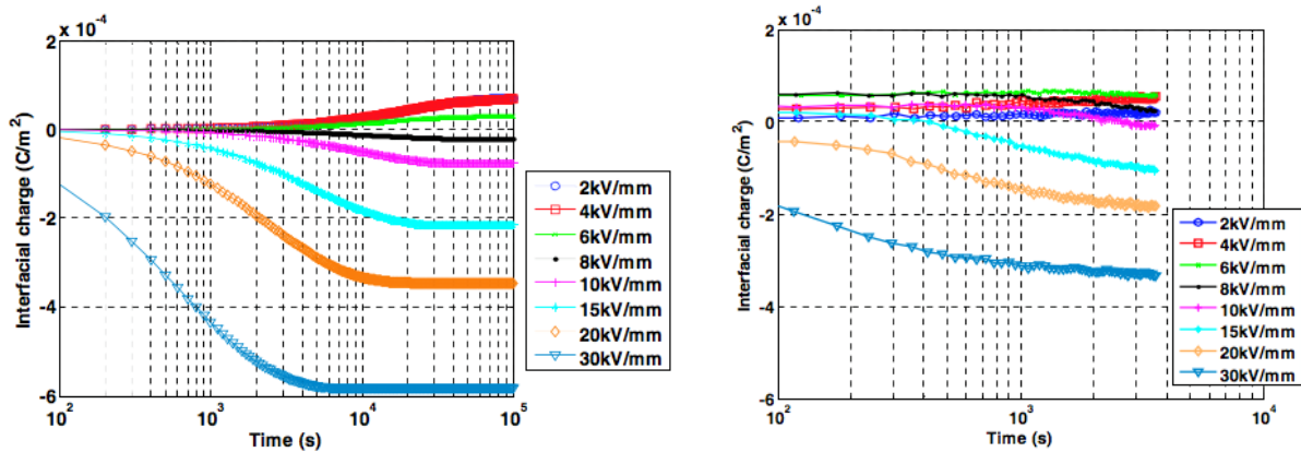
Figure 27. Charge interfaciale en fonction du temps pour différents champs électriques à T=40^{\circ}\text{C} obtenus a) par la modélisation macroscopique, et b) par la mesure (PEA) pour un bicouche XLPE/EPDM.
