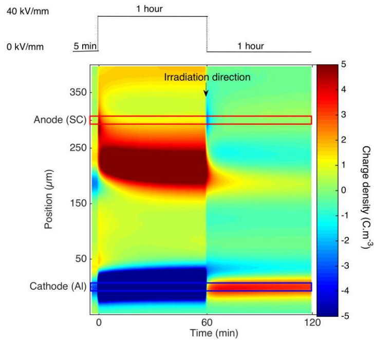
Figure 36: Cartographie de densité de charge nette pour un LDPE de 300 µm irradié par un faisceau d'électrons de 80keV pendant 10 min avec un courant de faisceau de 1 nA/cm 2 , mis en court-circuit pendant 5 min, polarisé ensuite pendant une heure à un champ électrique de 40 kV/mm, puis mis en court-circuit pendant une heure.
