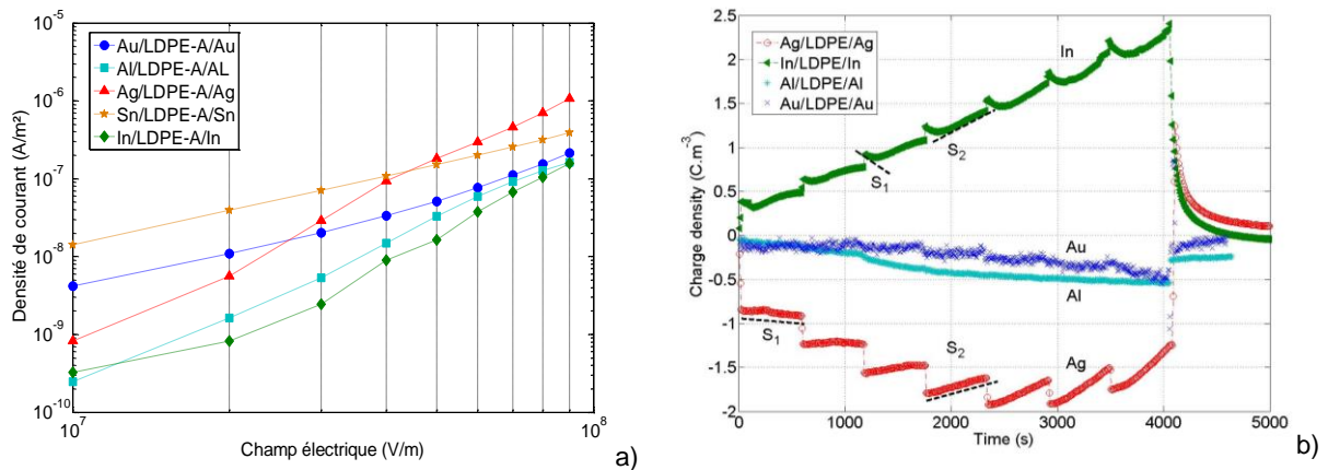
Figure 9: a) Densités de courant en fonction du champ électrique pour du LDPE avec différents métaux d'électrode à T=25^{\circ}\text{C} . b) Variation de la valeur moyenne de la densité nette de charges en fonction du temps pour le cycle de tension appliquée, pour différents métaux d'électrode. Les paliers correspondent aux champ électriques de 30, 40 ... 90 et 0 kV/mm.
