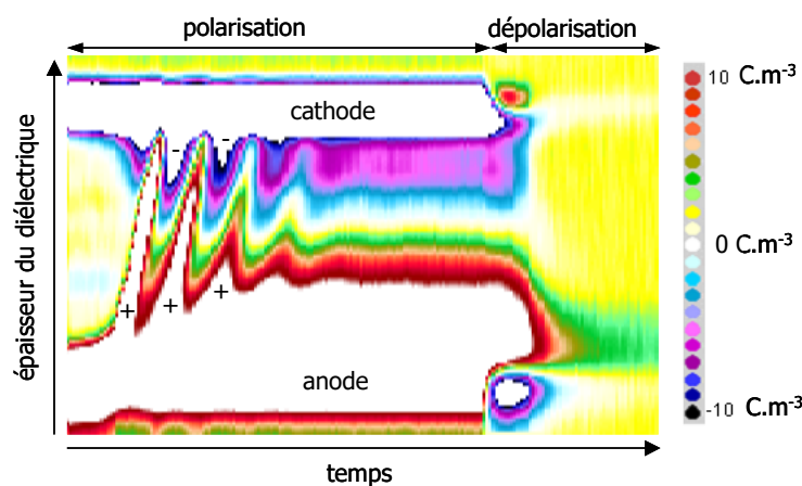
Figure 14: Mesure de la charge d'espace par PEA sur du polyéthylène basse densité, pour un champ appliqué de 80 \text{ kV}\cdot\text{mm}^{-1} , montrant la propagation de paquets de charges positives [68] (film de PE de 200 \mu\text{m} d'épaisseur, pour trois heures de polarisation et trois heures de dépolariation). La couleur blanche à proximité de chaque électrode montre une saturation de la densité nette de charges, et non une densité nulle.
