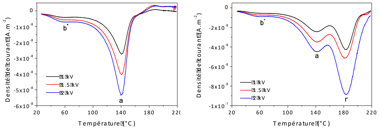
Figure 19: Spectres TSDC obtenus sur du PEN pour différentes tensions de polarisation a) pour une température de polarisation de 130°C et b) pour une température de polarisation de 170°C.
