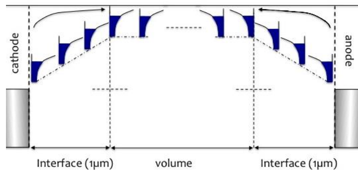
Figure 10. Représentation schématique de la modélisation d'une zone d'interface à chaque électrode, avec une distribution exponentielle de pièges dont les variables diminuent en s'éloignant de l'électrode.
