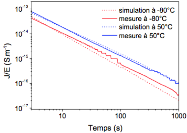
Figure 24. Comparaison des courants mesurés et simulés par le modèle de transport de charges où les phénomènes dipolaires ont été implémentés.
