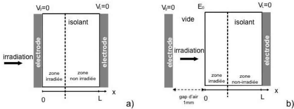
Figure 31. Schéma représentatif des configurations simulées pour le transport de charges dans un polymère irradié par faisceau d'électrons. a) configuration 'court-circuit' (i.e. électrodes à la masse), et b) configuration 'ouverte' (i.e. face irradiée en potentiel flottant, face non-irradiée à la masse).
