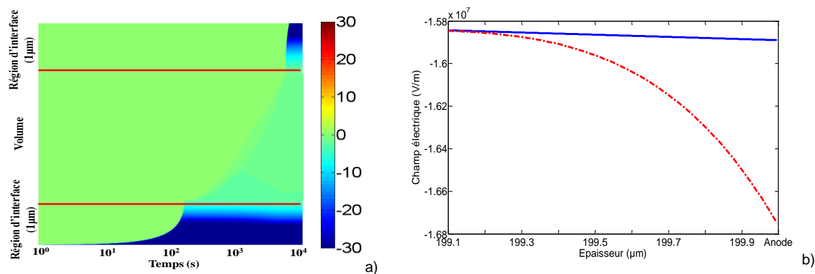
Figure 11. a) Cartographie de la densité d'électrons simulée en fonction de l'épaisseur de l'échantillon et du temps pour un champ appliqué de 10 kV/mm. Echelle logarithmique pour l'axe des x. De haut en bas: région d'interface proche de l'anode, volume du diélectrique, région d'interface proche de la cathode. b) Champ électrique en fonction de la position dans la zone d'interface proche de l'anode, avec (ligne pointillée) et sans (trait plein) états d'interface. Les données sont prises après 3h de polarisation à 10 kV/mm et à température ambiante.
