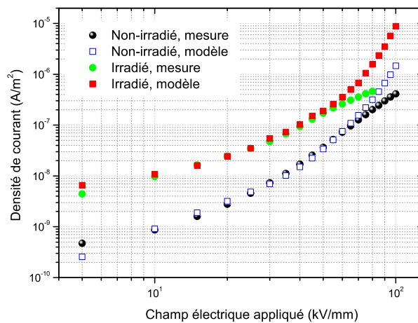
Figure 37. Densité de courant mesurée et modélisée en fonction du champ électrique appliqué pour des films LDPE irradiés et non-irradiés.
