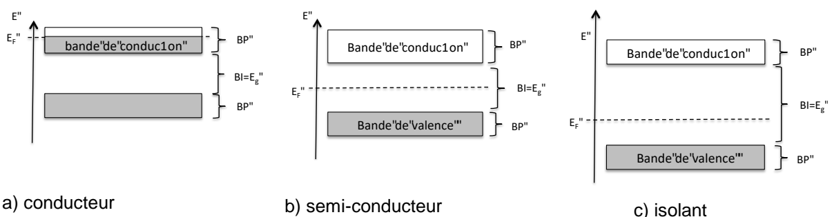
Figure 1. Remplissage des niveaux d'énergie à T=0K : a) cas d'un conducteur, b) cas d'un semi-conducteur, dont la bande interdite, ou E_G < 2 eV, c) cas d'un isolant.
