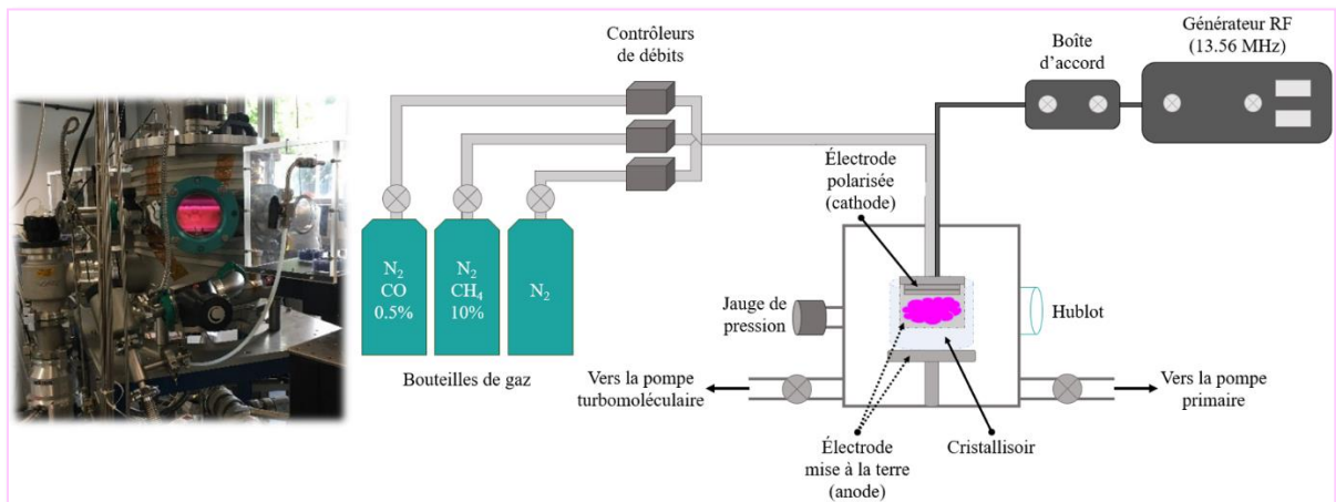
Figure E : Photographie (à gauche) et schéma (à droite) du dispositif expérimental PAMPRE utilisé pour simuler la chimie atmosphérique de Pluton et synthétiser des analogues d’aérosols photochimiques.
