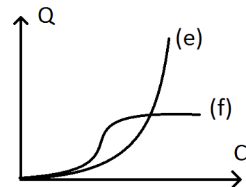
Figure 10. Différents types de relations observés entre la concentration d'un composé sorbé Q et dissout C (Schwarzenbach et al., 2003)
