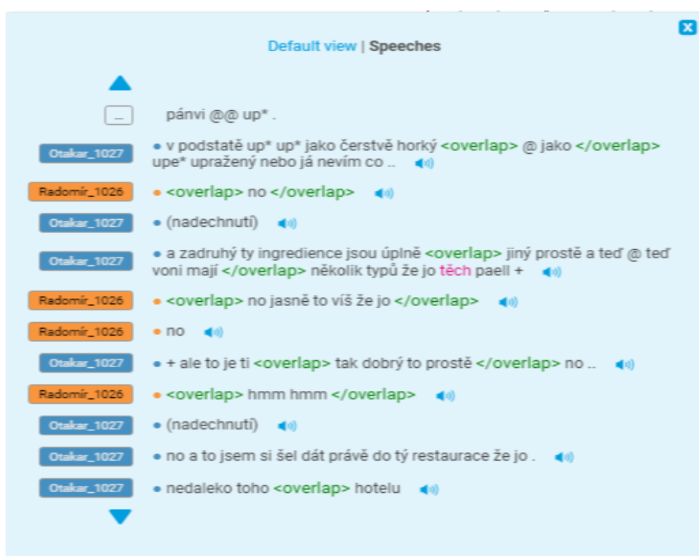
Figure 2.1 : Interface d'ORTOFON v1 (CNT)
