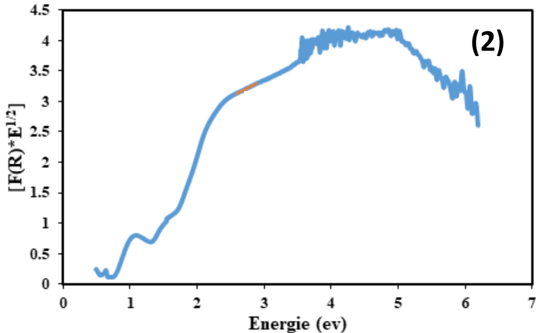
Figure III.24: Courbes de Tauc pour l'échantillon copécipité à partir de nitrates de Zn et de Fe introduits en quantités stœchiométriques et avec une addition de 3,6 g de surfactant L64, à, pH=12. La première courbe (A) est relative à la mesure du BG sur un oxyde semi-conducteur présentant un BG direct. La seconde courbe (B) est relative à un oxyde semi-conducteur présentant un BG indirect.
