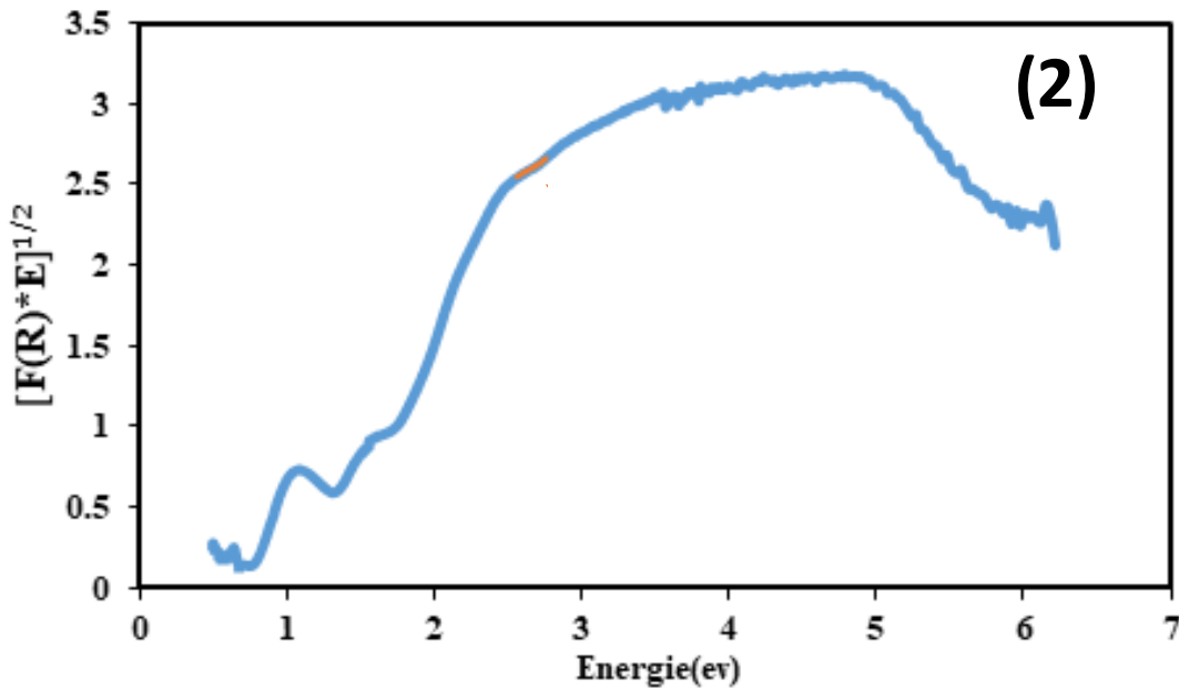
Figure III.22: Courbes de Tauc pour l'échantillon copécipité à l'éthanol à partir de nitrates de Zn et de Fe. La première courbe (A) est relative à la mesure du BG sur un oxyde semi-conducteur présentant un BG direct. La seconde courbe (B) est relative à un oxyde semi-conducteur présentant un BG indirect..
