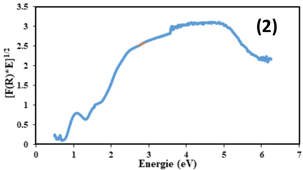
Figure III.21: Courbes de Tauc, pour l'échantillon coprécipité à l'eau à partir de nitrates de Zn et de Fe. La première courbe (1) est relative à la mesure du BG sur un oxyde semi-conducteur présentant un BG direct. La seconde courbe (2) est relative à un oxyde semi-conducteur présentant un BG indirect.
