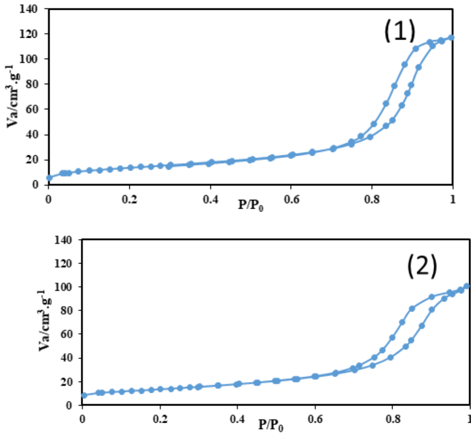
Figure III.16: Isothermes de physiorption d'azote. Co-précipitation de \text{Zn}(\text{NO}_3)_2 \cdot 6\text{H}_2\text{O} et \text{Fe}(\text{NO}_3)_3 \cdot 9\text{H}_2\text{O} à pH 14 dans l'eau et en présence de (1) : 1,8 g et (2) : 0,5 g de L64.
