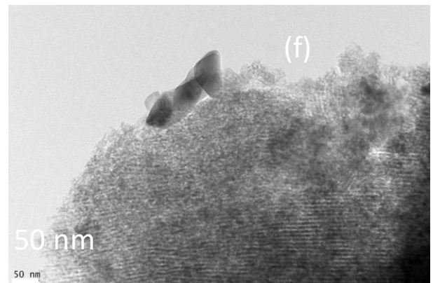
Figure IV.1: Micrographies MEB des poudres de l'échantillon (a) Fe Zn/SBA-15_NO 3 _ (b) Micrographies MEB des poudres de l'échantillon Fe Zn/SBA-15_Cl_ (c) Micrographies MET des poudres de l'échantillon Fe Zn/SBA-15_NO 3 _ (d), (e) et (f). Micrographies MET des poudres de l'échantillon Fe Zn/SBA-15_Cl
