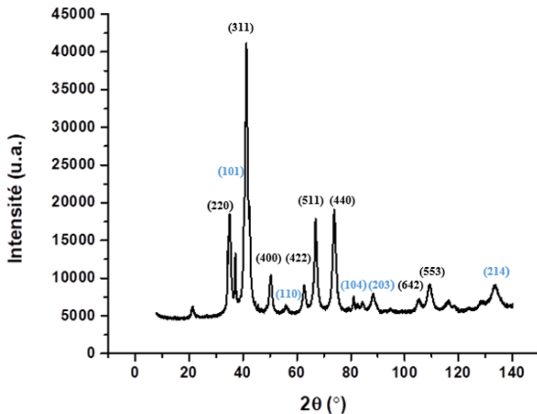
Figure III.8: DRX obtenus sur un appareil muni d’une anticathode au cobalt : coprécipité avec des nitrates métalliques et avec addition de 3,6g de L64 (pH=12). Indexation pour une maille cubique de ZnFe_2O_4 en noir (conforme à la fiche ICDD 77-0011). Indexation pour une maille hexagonale de ZnO en bleu (conforme à la fiche ICDD 01-089-1397).
