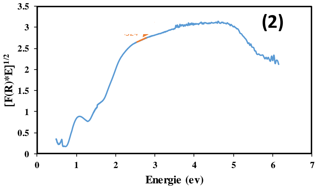
Figure III.23: Courbes de Tauc, pour l'échantillon coprécipité à partir de nitrates de Zn et de Fe introduits en quantités stœchiométriques et avec une addition de surfactant P123=3,6 g, pH=12. La première courbe (1) est relative à la mesure du BG sur un oxyde semi-conducteur présentant un BG direct. La seconde courbe (2) est relative à un oxyde semi-conducteur présentant un BG indirect.
