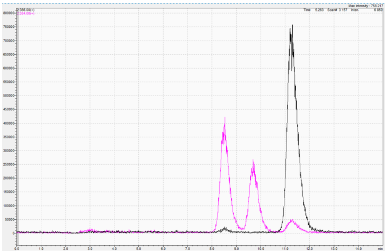
Figure III.26: Chromatogrammes HPLC pour une solution d'AMX dans l'eau après 48 h sous irradiation visible (en noir) et pour une solution d'AMX après un test photocatalytique (en rose).
