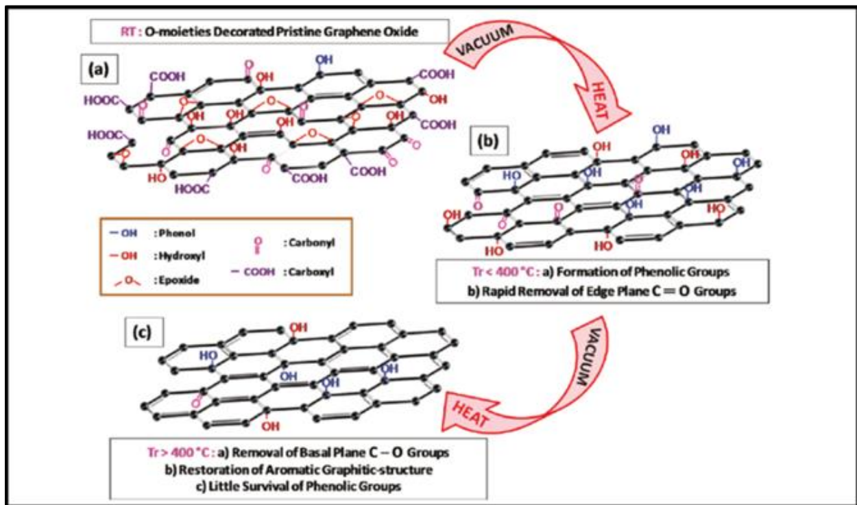
Figure I.4: Une représentation d'un plan de graphène et de son évolution lors d'un traitement thermique (84).
