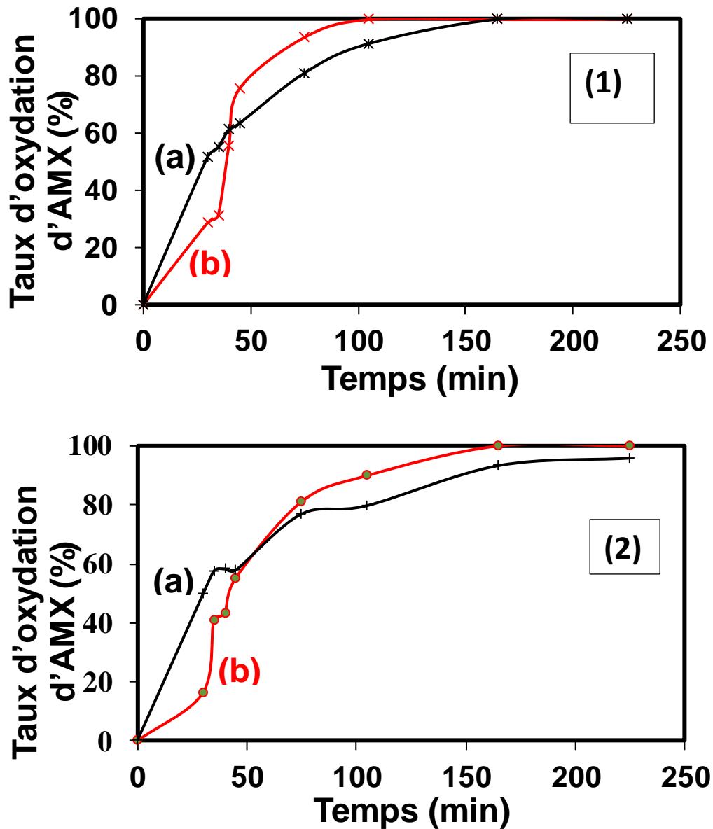
Figure V.11: Activités catalytiques des mélanges contenant de la phase spinelle ZnFe_2O_4 obtenu par synthèse hydrothermale (a) :avec graphène oxydé (GO) %.(b) : sans graphène ZnFe_2O_4 86%, ZnO 10%, hémate 4% (1) : Lumière, (2) : Obscurité.
