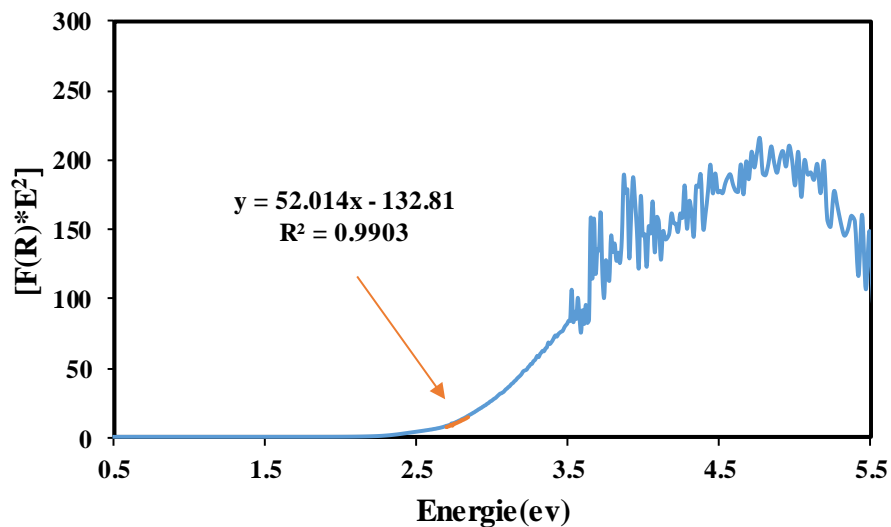
Figure IV.10: Courbe de Tauc pour l'échantillon Fe Zn/SBA-15, Nitrate 2S (1). La courbe est relative à la mesure du BG sur un oxyde semi-conducteur présentant un BG direct.
