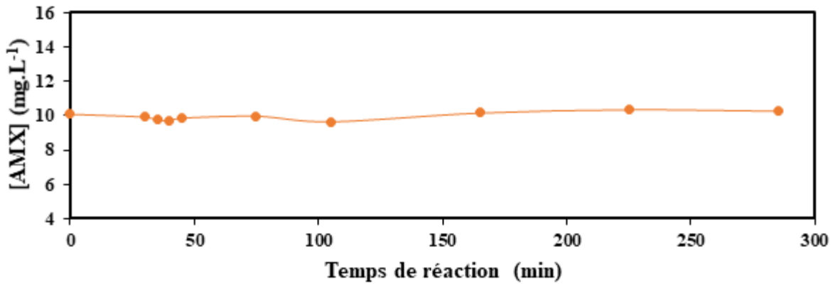
Figure III.25: Concentration d'AMX en fonction du temps dans le cas d'un test sous lumière en absence de catalyseur. La concentration d'AMX a été suivie par HPLC.
