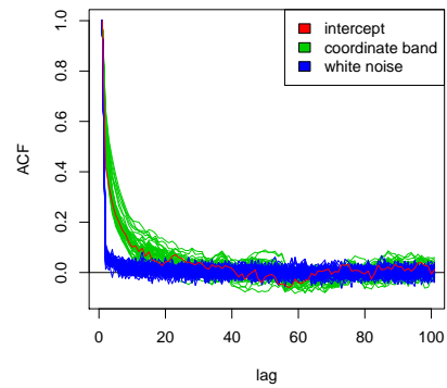
(d) Autocorrelations of our implementation
