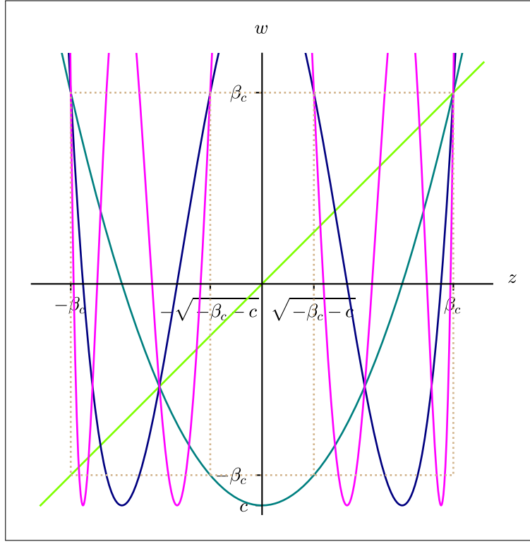
FIGURE 4. Courbes représentatives des applications z \mapsto f_c^{on}(z) , avec c \in ]-\infty, -2] fixé et n \in \{0, \dots, 3\} .
