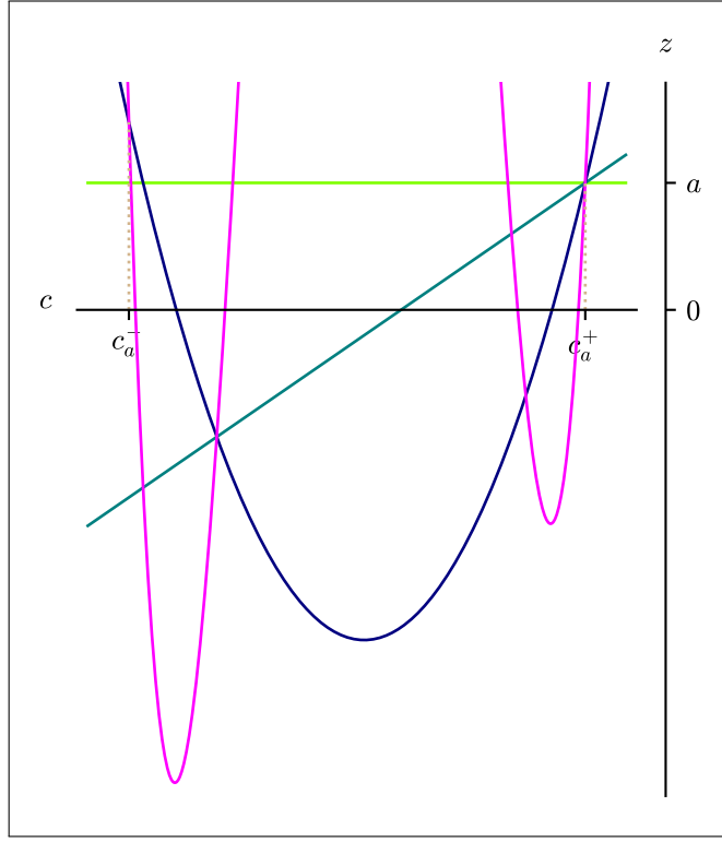
FIGURE 6. Courbes représentatives des applications c \mapsto f_c^{on}(a) , avec a \in [2, +\infty[ fixé et n \in \{0, \dots, 3\} .
