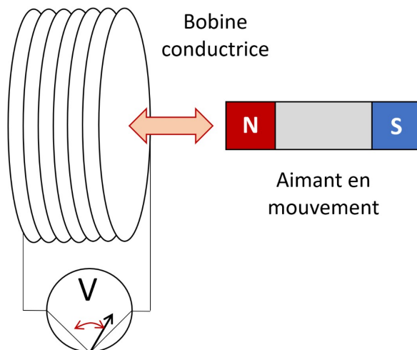
FIGURE 3.2 – Illustration de la loi de l'induction électromagnétique à la base de l'apparition des courants de Foucault. Le mouvement d'un aimant à proximité d'une bobine conductrice provoque l'apparition d'une force électromotrice au sein de cette dernière.
