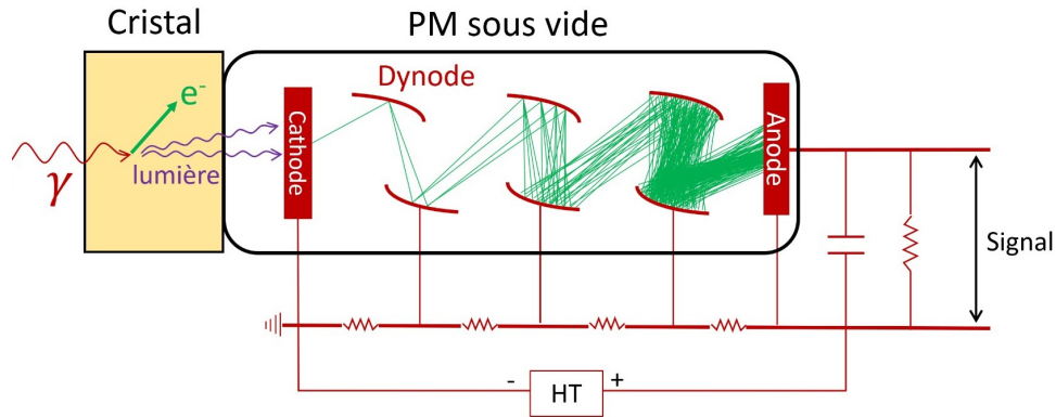
FIGURE 1.3 – Schéma simplifié du fonctionnement d'un tube PMT. La haute tension (HT) appliqué est de l'ordre de 1000 V (elle est d'autant plus haute que le nombre de dynodes est important). Seules trois dynodes ont été représentées sur le schéma. Un véritable PMT de système TEP en compte une dizaine. Pour simplifier, la trajectoire des électrons entre les dynodes a été représenté par une ligne droite.
