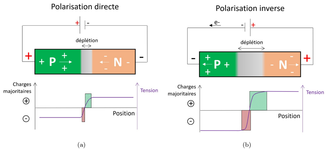
FIGURE 1.9 – Représentation schématique de deux jonctions PN. (a) Jonction PN polarisée en direct. Cette configuration réduit la zone de déplétion et la barrière de potentiel associée, et autorise la circulation du courant dans la diode. (b) Jonction PN polarisée en inverse. Les électrons du côté N sont attirés par la cathode (borne +) et réciproquement, ce qui augmente sensiblement le volume de la zone de déplétion et la barrière de potentiel. La diode polarisée en inverse s'oppose au passage du courant.
