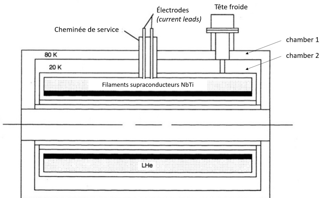
FIGURE 2.17 – Coupe sagittale de l’aimant Signa 1.5 T commercialisé par General Electric Healthcare dans les années 1980. Un cryostat GMc à deux étages assure le blindage thermique du supraconducteur baignant dans l’hélium liquide dont l’évaporation est évaluée à 0.2 l/h.
