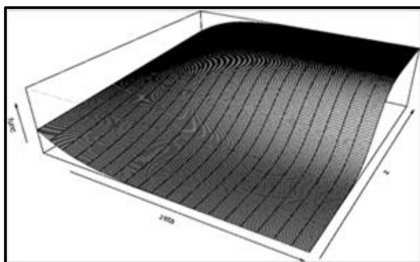
Figure 30 : La fonction de transition pour le modèle logistique LSTAR 92 .
