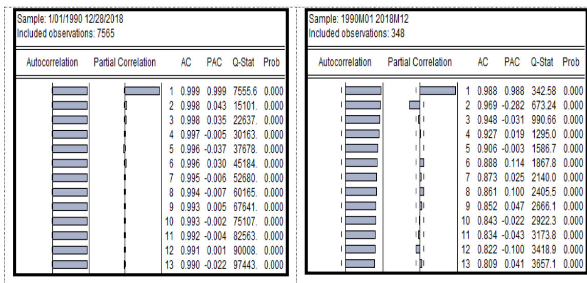
Figure 28 : Le corrélogramme de prix du pétrole journalier et mensuelle.
