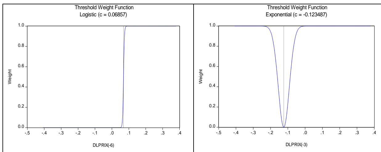
Figure 42 : les fonctions Logistique et Exponentiel de lissage estimé pour la fréquence mensuelle.
