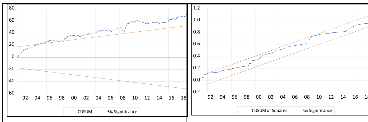
Figure 41 : Tests de stabilité Cusum et Cusum aux carrés
