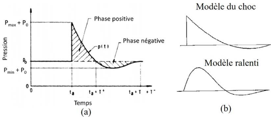
Figure 1.4: Modèle idéal d'onde de choc (a), issu de [Strehlow and Baker, 1976]. Schémas simplifié du modèle idéal d'une onde de choc et d'un modèle ralenti (non-discontinuité de la pression)-(b), issue de [C.J.H. van den Bosch and R.A.P.M. Weterings, 1996]
