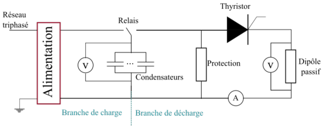
Figure 2.3: Schéma de principe du circuit électrique
